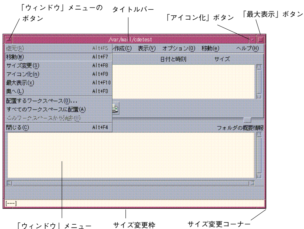
図 1-4 CDE ウィンドウのコントロール
