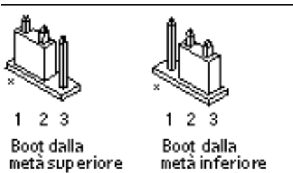
Figura 5-6 Impostazione del jumper di controllo del boot per l'esecuzione del boot dalla metà inferiore o dalla metà superiore
