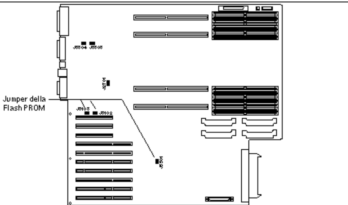
Figura 5-7 Posizione dei jumper della Flash PROM sui sistemi Sun Enterprise 450 e sulle workstation Sun Ultra 450
