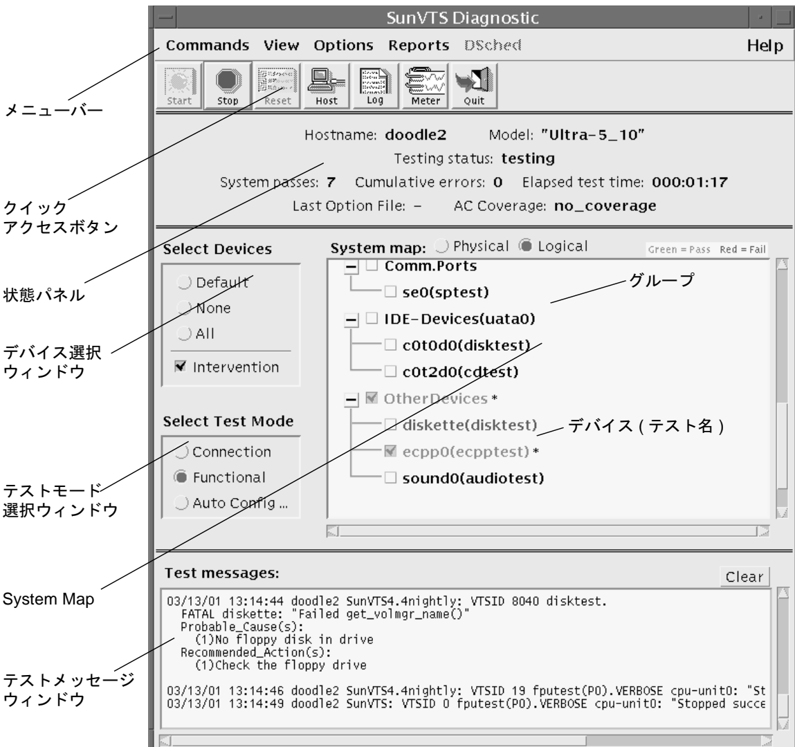
図 A-1 SunVTS CDE メインウィンドウ
