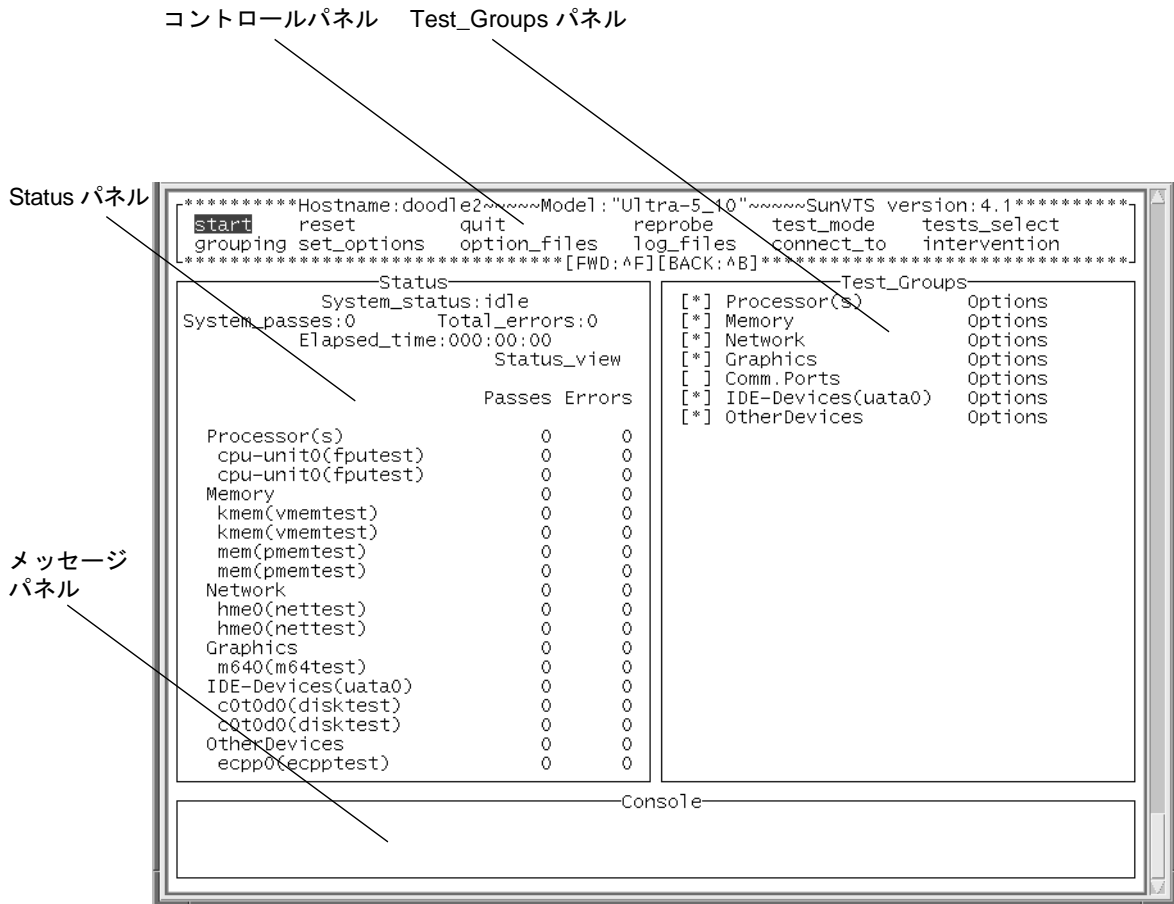
図 6-1 SunVTS TTY メインウィンドウ
