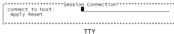
図 A-6 Connect to Host ダイアログボックス
