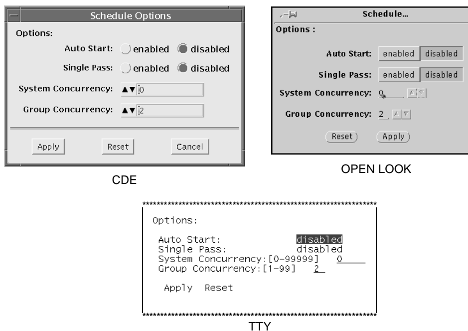
図 A-10 Schedule ダイアログボックス
