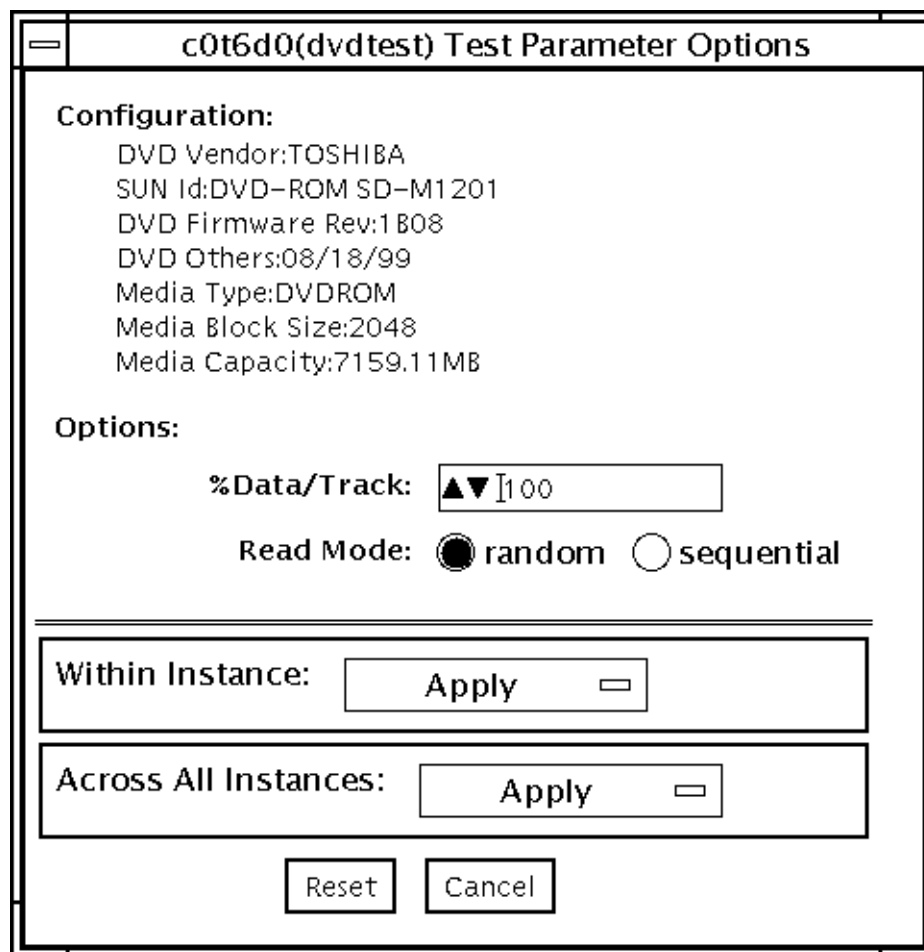
図 15-1 dvdtest のテストパラメタオプションダイアログボックス
