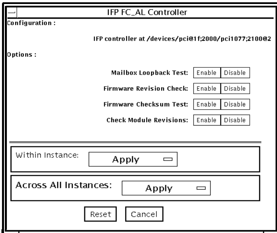
図 32-1 ifptest テストパラメタオプションダイアログボックス
