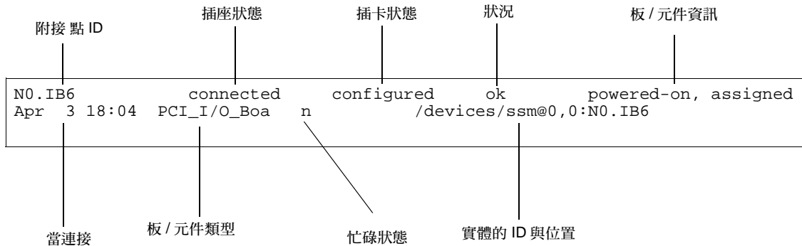
圖 2-1 cfmadm -av 顯示的詳細內容
