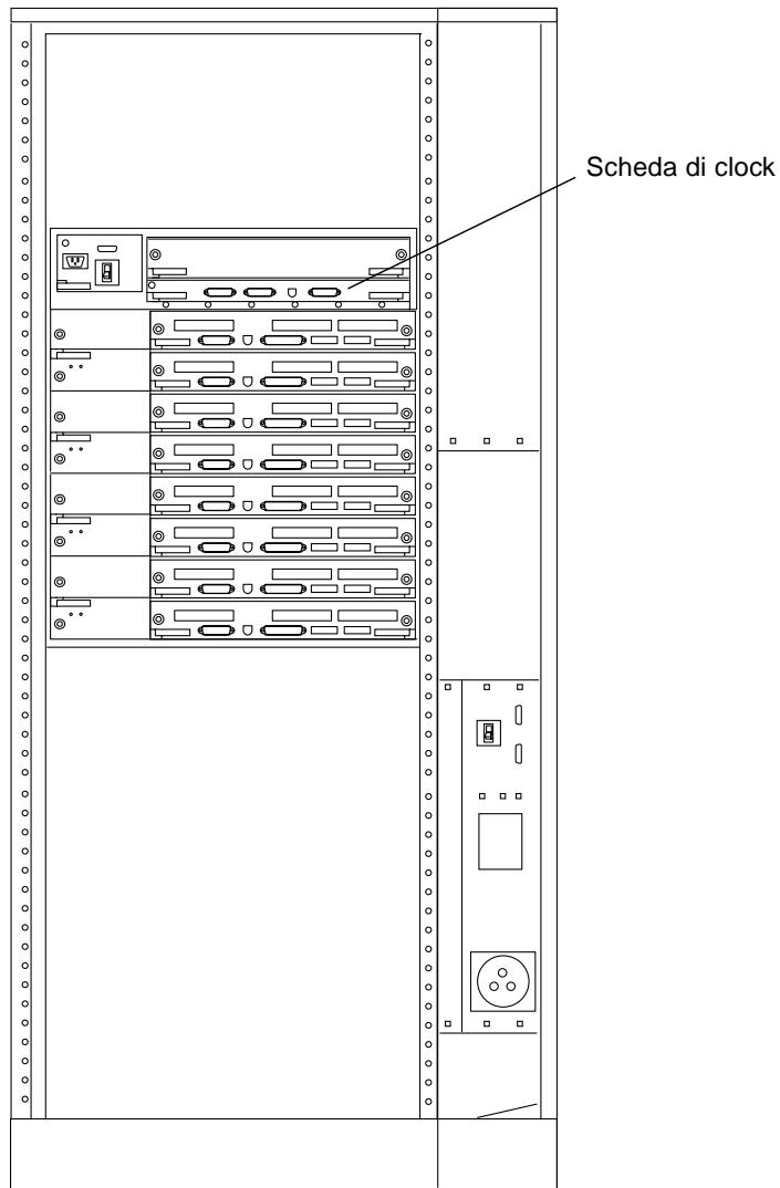
FIGURA 6-2 Vista posteriore del sistema Sun Enterprise 6000
