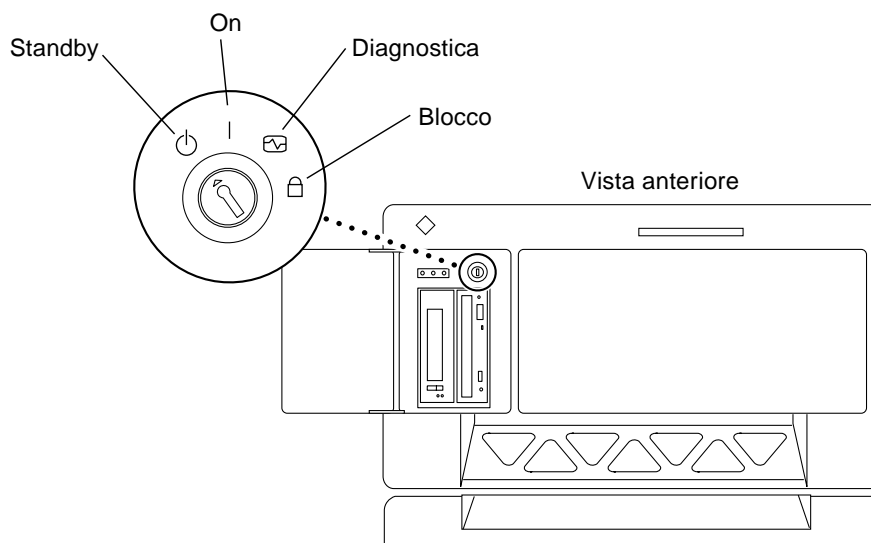
FIGURA 6-1 Posizione degli interruttori a chiave sui sistemi Sun Enterprise 6x00, 5x00, 4x00, 3x00
