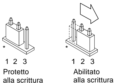
FIGURA 5-3 Impostazione del jumper di protezione/abilitazione alla scrittura nella posizione di abilitazione alla scrittura
