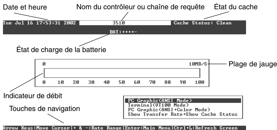
FIGURE 6-1 Fenêtre initiale du microprogramme
