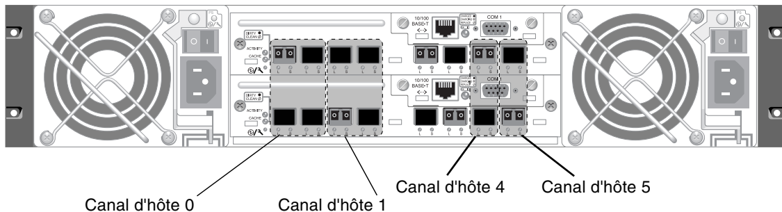
FIGURE 4-10 Canaux d'hôte sur une baie Sun StorEdge 3511 FC à deux contrôleurs
