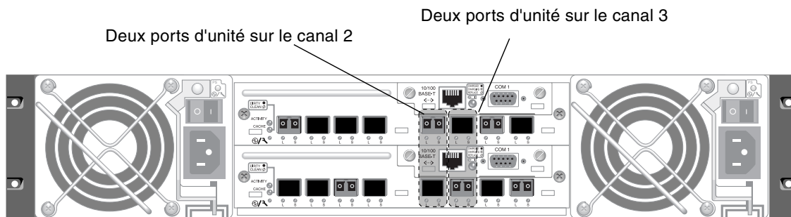
FIGURE 4-8 Canaux d'unité dédiés n°2 et 3 (sur les deux contrôleurs) dans une baie Sun StorEdge 3511 FC à deux contrôleurs
