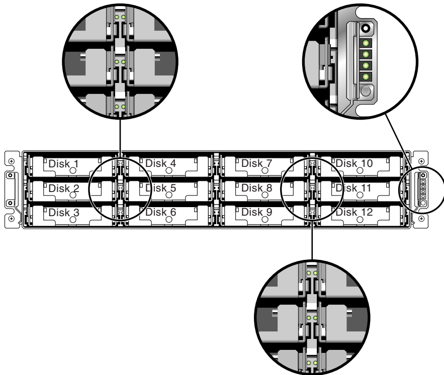
FIGURE 4-6 Panneau avant des baies Sun StorEdge 3510 et 3511 FC avec les DEL
