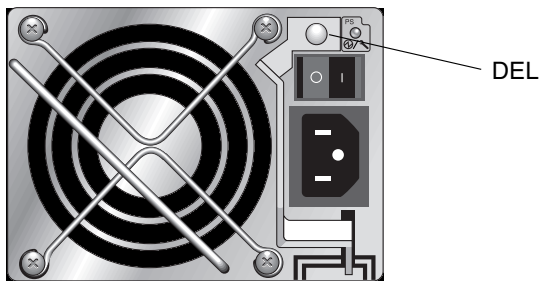
FIGURE 7-7 Module d'alimentation CA et de ventilation
