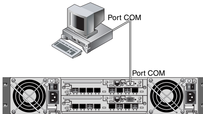
FIGURE J-1 Port COM d'une baie RAID connecté localement au port série d'un système hôte
