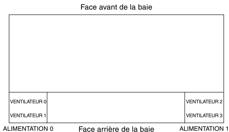
FIGURE 8-1 Emplacement des ventilateurs de refroidissement
