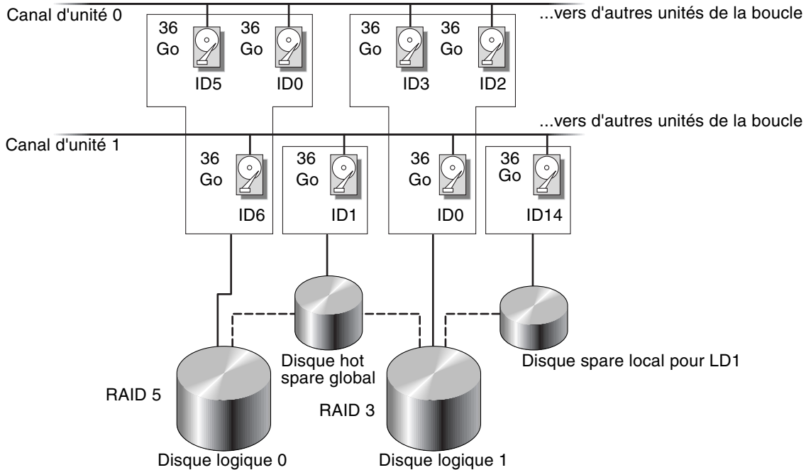
FIGURE 6-3 Exemple d'allocation de disques hot spare locaux et globaux dans les configurations logiques
