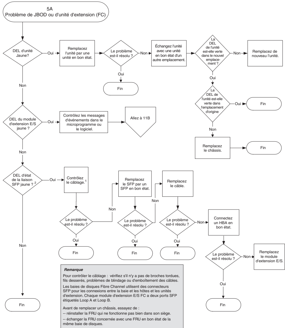
FIGURE B-4 Organigramme de dépannage d'une unité JBOD/d'extension 1/2
