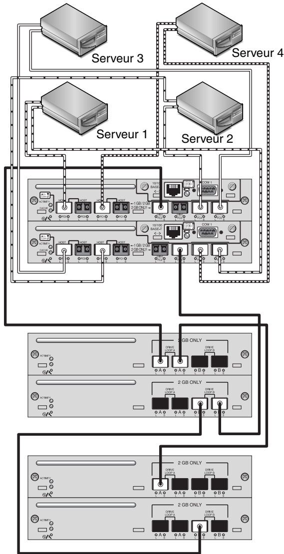
FIGURE 5-4 Configuration DAS incluant quatre serveurs, une baie Sun StorEdge 3511 FC à deux contrôleurs et deux unités d'extension
