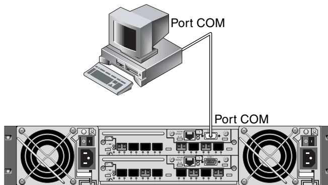
FIGURE F-1 Port COM d'une baie RAID connecté localement au port série d'une station de travail
