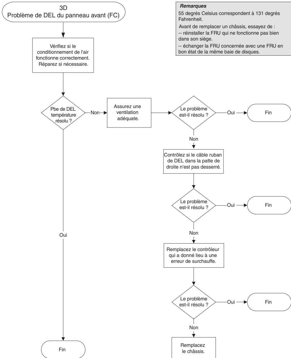
FIGURE 9-13 Organigramme des DEL du panneau avant, 4/4
