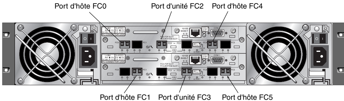
FIGURE 4-11 Mise en place par défaut des SFP d'une baie Sun StorEdge 3510 FC à deux contrôleurs
