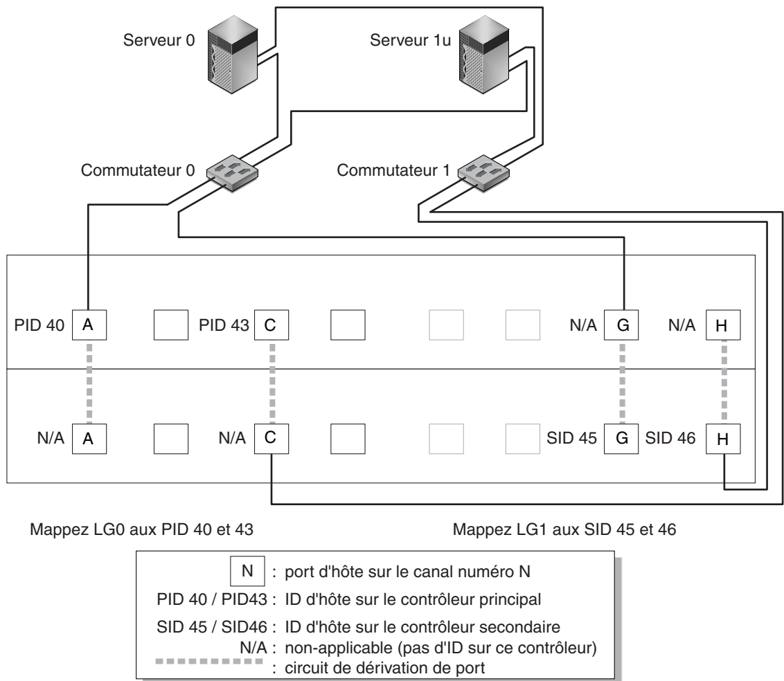
FIGURE 5-2 Configuration point-à-point avec une baie Sun StorEdge 3511 FC à deux contrôleurs et deux commutateurs
