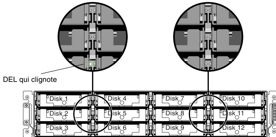
FIGURE 9-3 Clignotement de la DEL d'une unité sélectionnée
