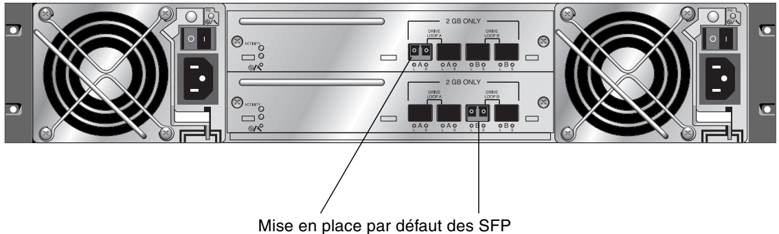
FIGURE 4-16 Mise en place par défaut des SFP dans une unité d'extension SUN StorEdge 3511
