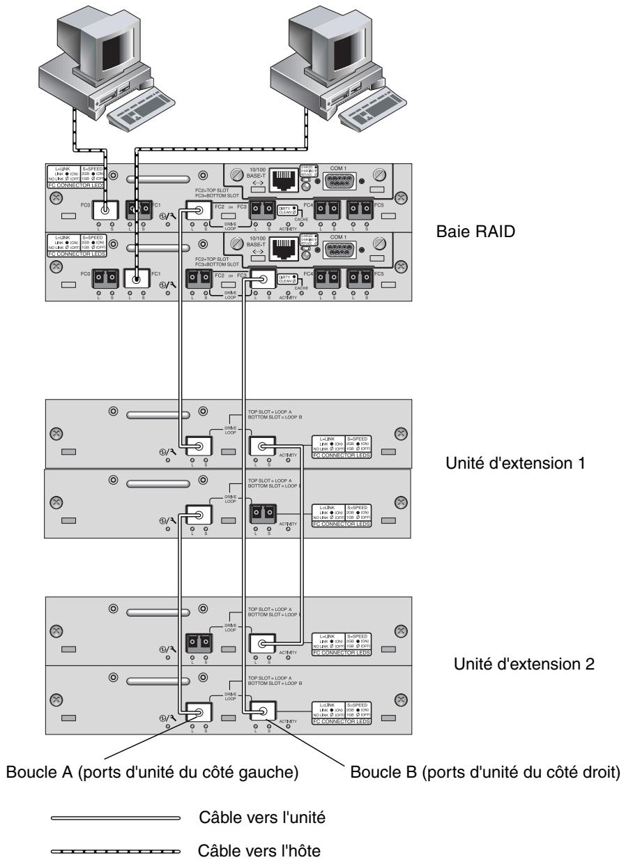
FIGURE 4-18 Baie Sun StorEdge 3510 FC rattachée à deux hôtes et deux unités d'extension
