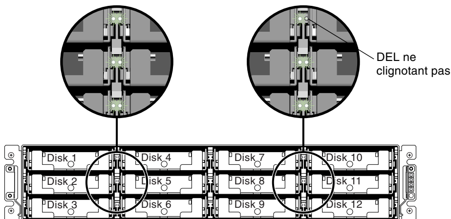
FIGURE 9-5 Clignotement de toutes les DEL d'unités à l'exception d'une DEL d'unité sélectionnée
