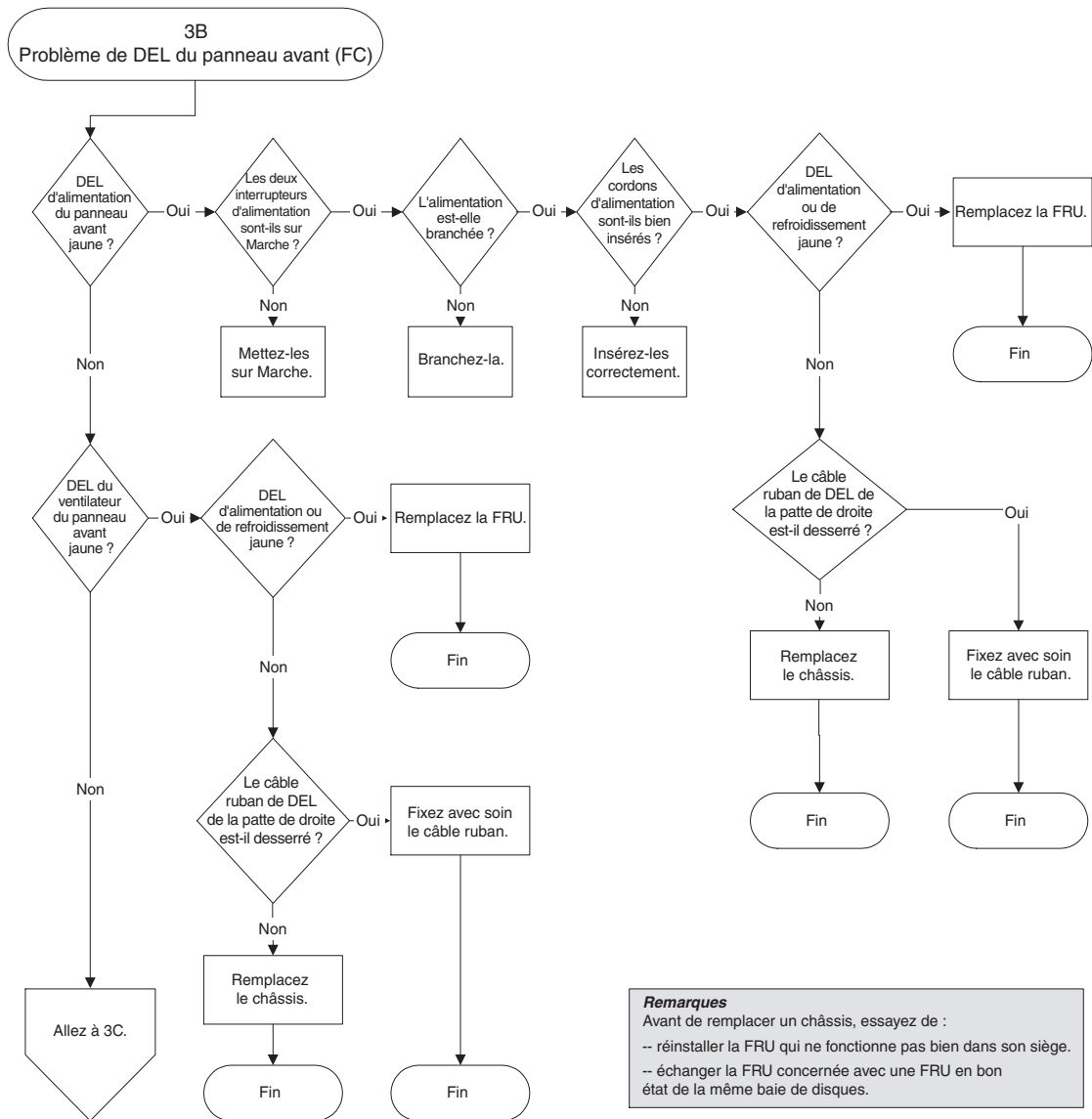
FIGURE 9-11 Organigramme des DEL du panneau avant, 2/4
