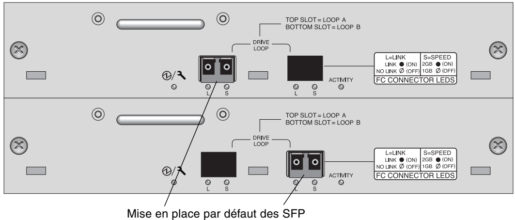
FIGURE 4-15 Mise en place par défaut des SFP dans une JBOD/unité d'extension Sun StorEdge 3510
