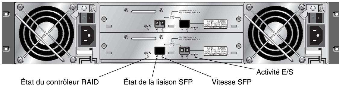
FIGURE 7-5 Modules d'extension E/S pour une unité d'extension Sun StorEdge 3510 FC
