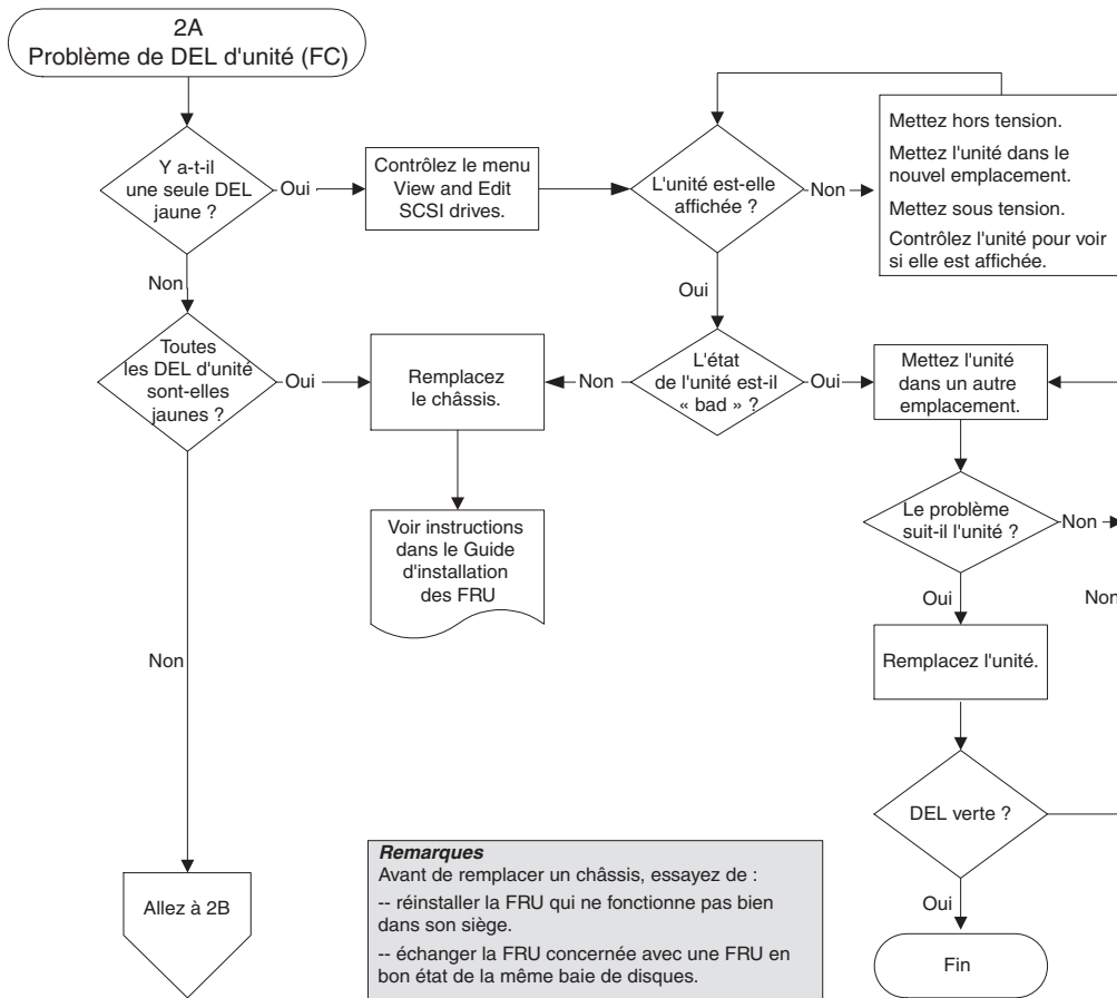
FIGURE 9-8 Organigramme des DEL des unités FC, 1/2
