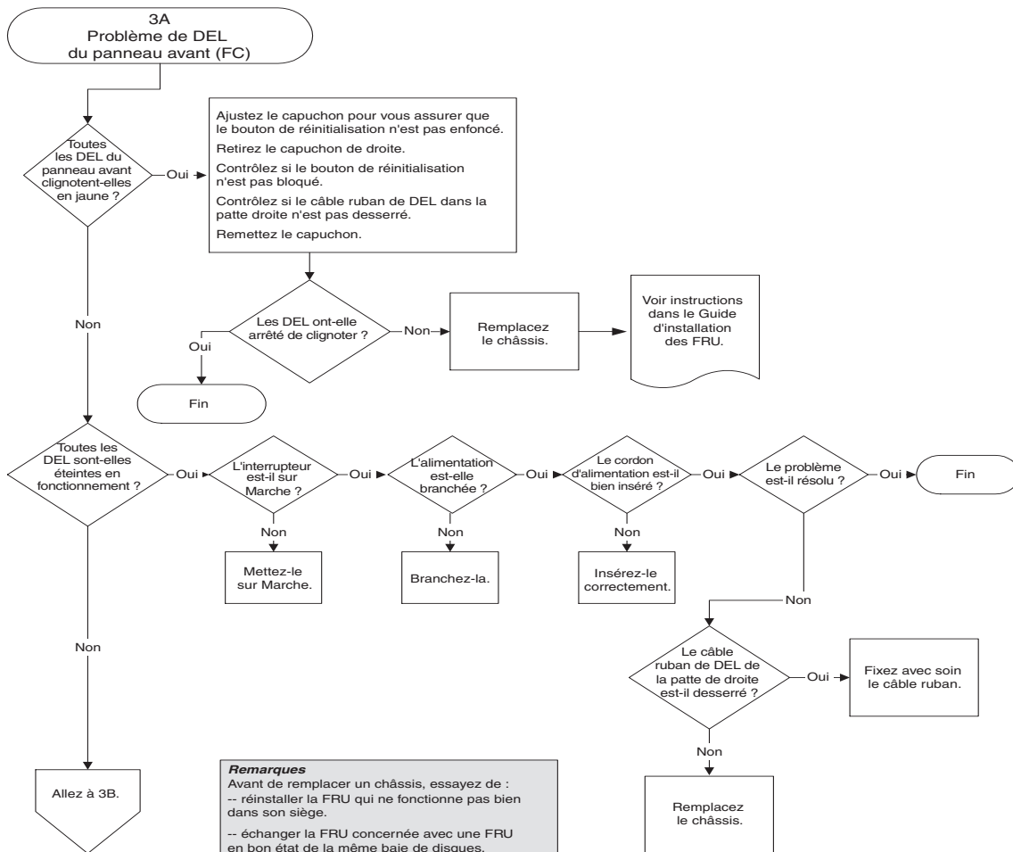
FIGURE 9-10 Organigramme des DEL du panneau avant (FC), 1/4
