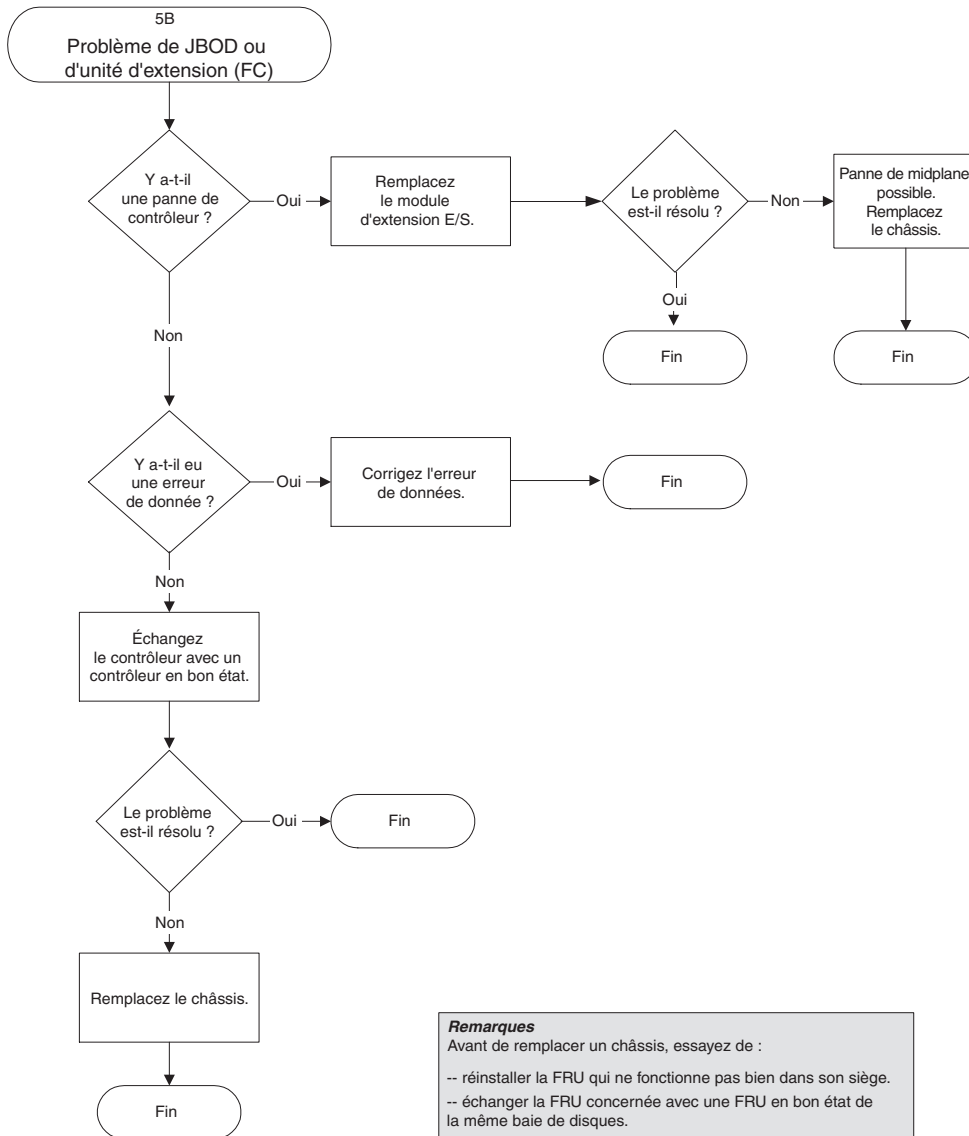
FIGURE B-5 Organigramme de dépannage d'une unité JBOD/d'extension 2/2
