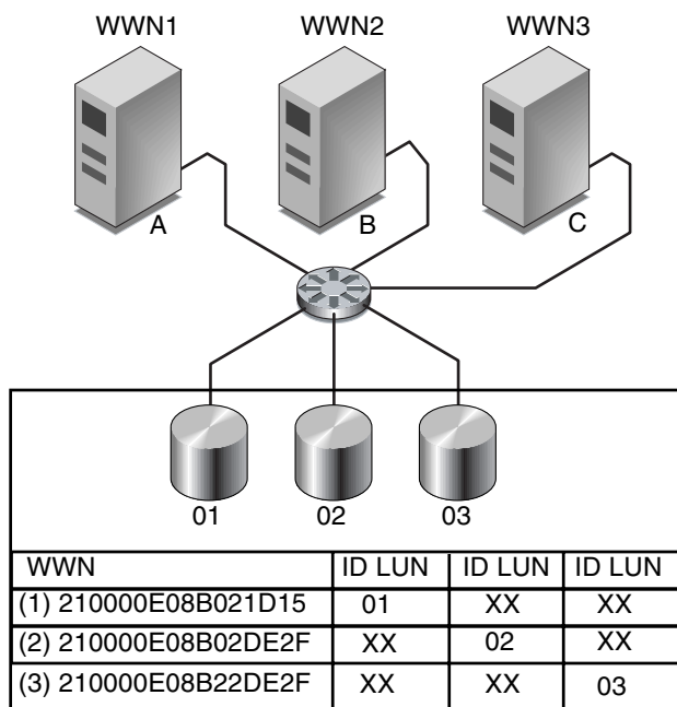
FIGURE 6-6 Exemple de filtrage de LUN
