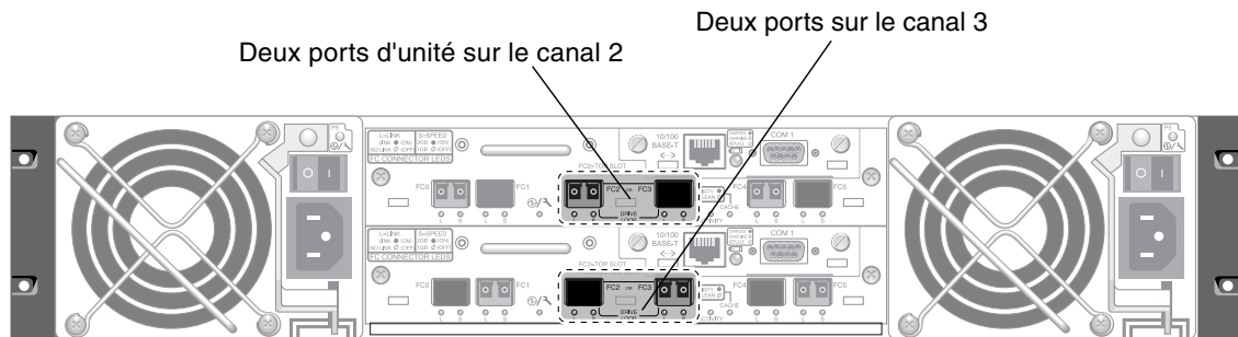
FIGURE 4-7 Canaux d'unité dédiés n°2 sur le contrôleur supérieur et 3 sur le contrôleur inférieur dans une baie Sun StorEdge 3510 FC à deux contrôleurs
