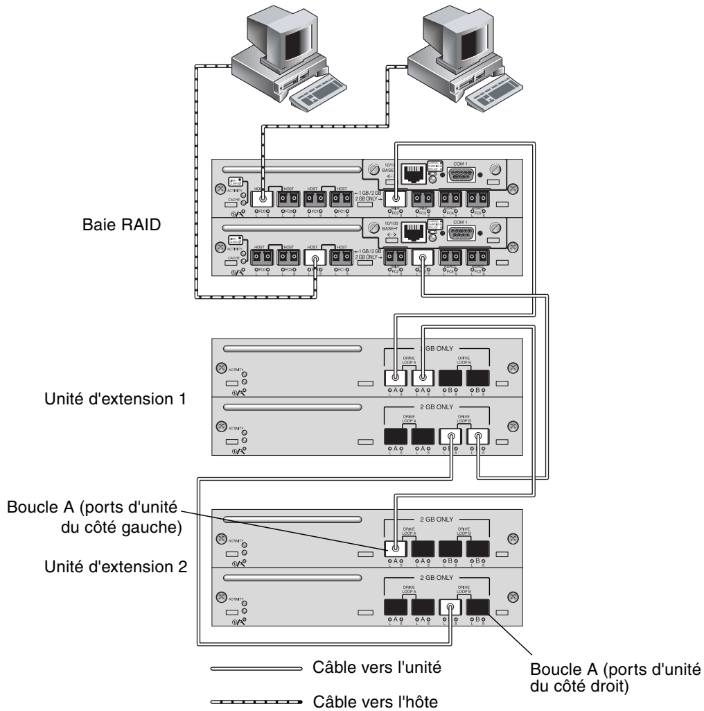
FIGURE 4-19 Baie Sun StorEdge 3511 FC rattachée à deux hôtes et deux unités d'extension
