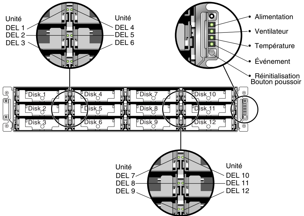
FIGURE 7-1 DEL du panneau avant
