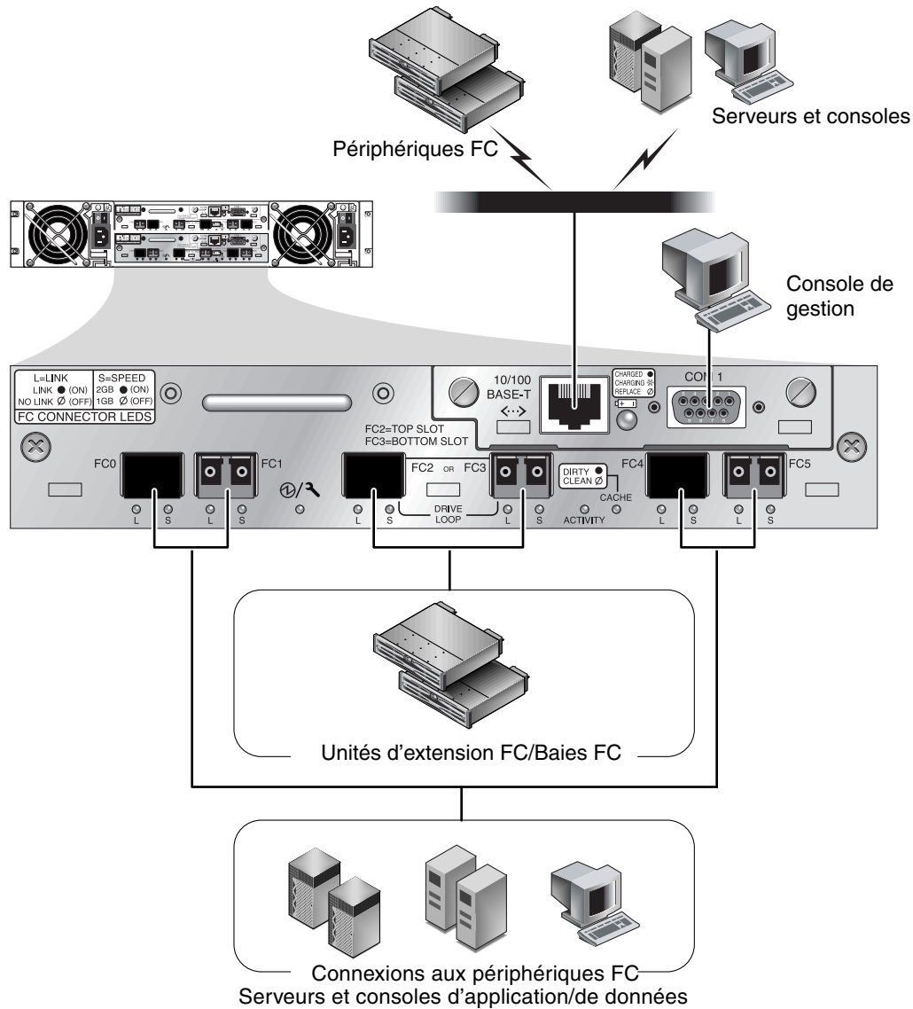
FIGURE 4-3 Connexions physiques à l'arrière d'une baie de disques Sun StorEdge 3510 FC à deux contrôleurs
