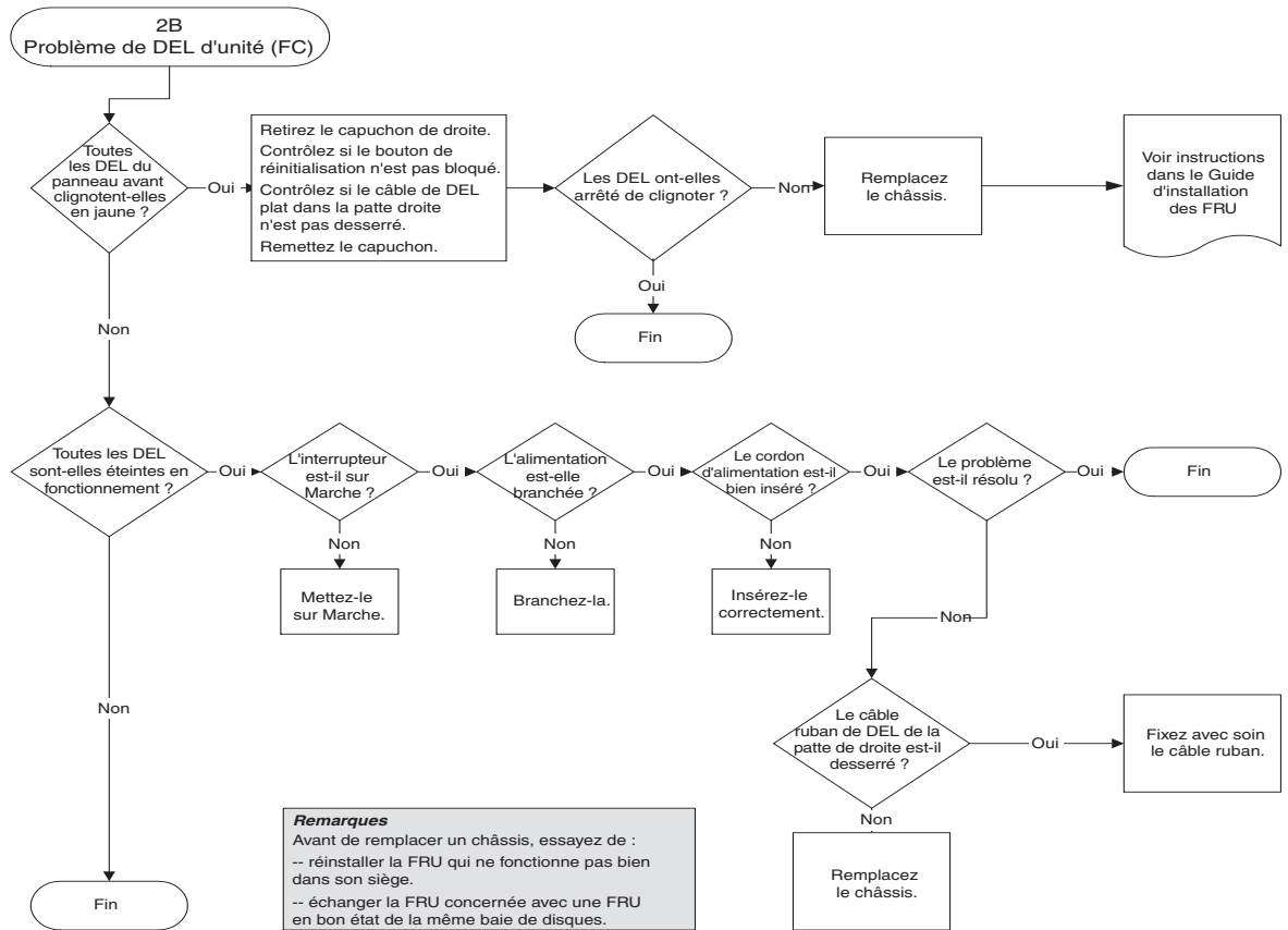
FIGURE 9-9 Organigramme des DEL des unités FC, 2/2
