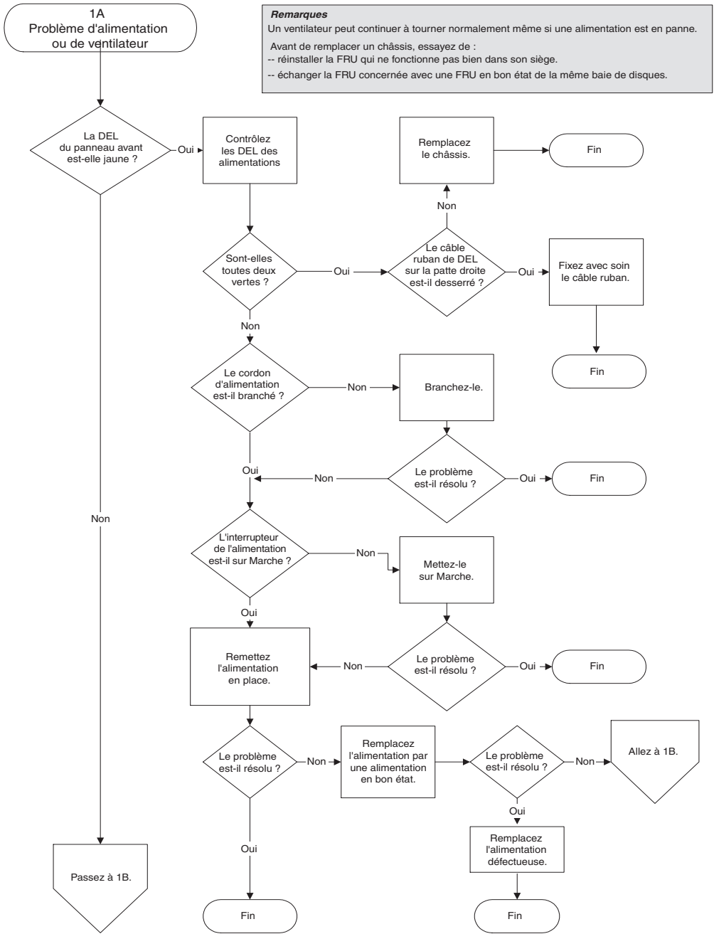
FIGURE 9-6 Organigramme du module de ventilation et d'alimentation, 1/2
