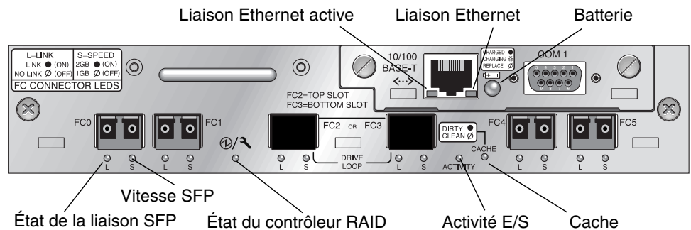
FIGURE 7-3 DEL du module contrôleur E/S et du module batterie d'une baie FC Sun StorEdge 3510
