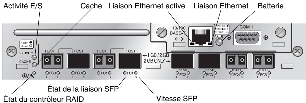
FIGURE 7-4 DEL du module contrôleur E/S et du module batterie d'une baie FC Sun StorEdge 3511
