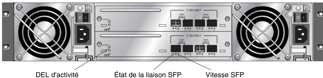
FIGURE 7-6 Modules d'extension E/S pour une unité d'extension Sun StorEdge 3511 FC
