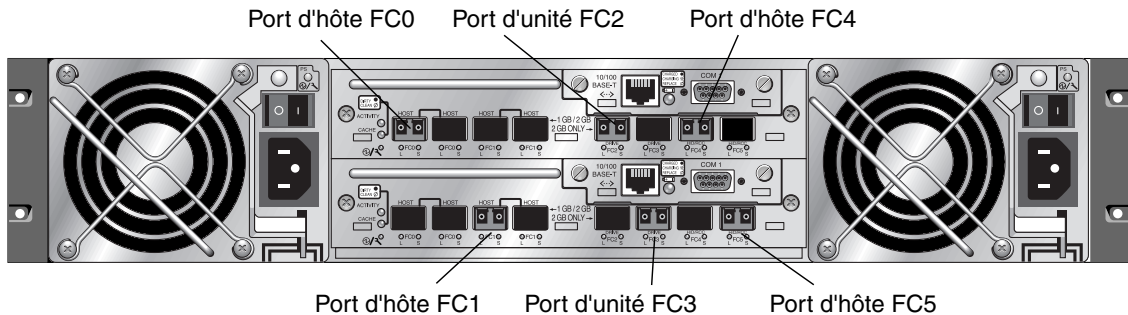
FIGURE 4-12 Mise en place par défaut des SFP d'une baie Sun StorEdge 3511 FC à deux contrôleurs
