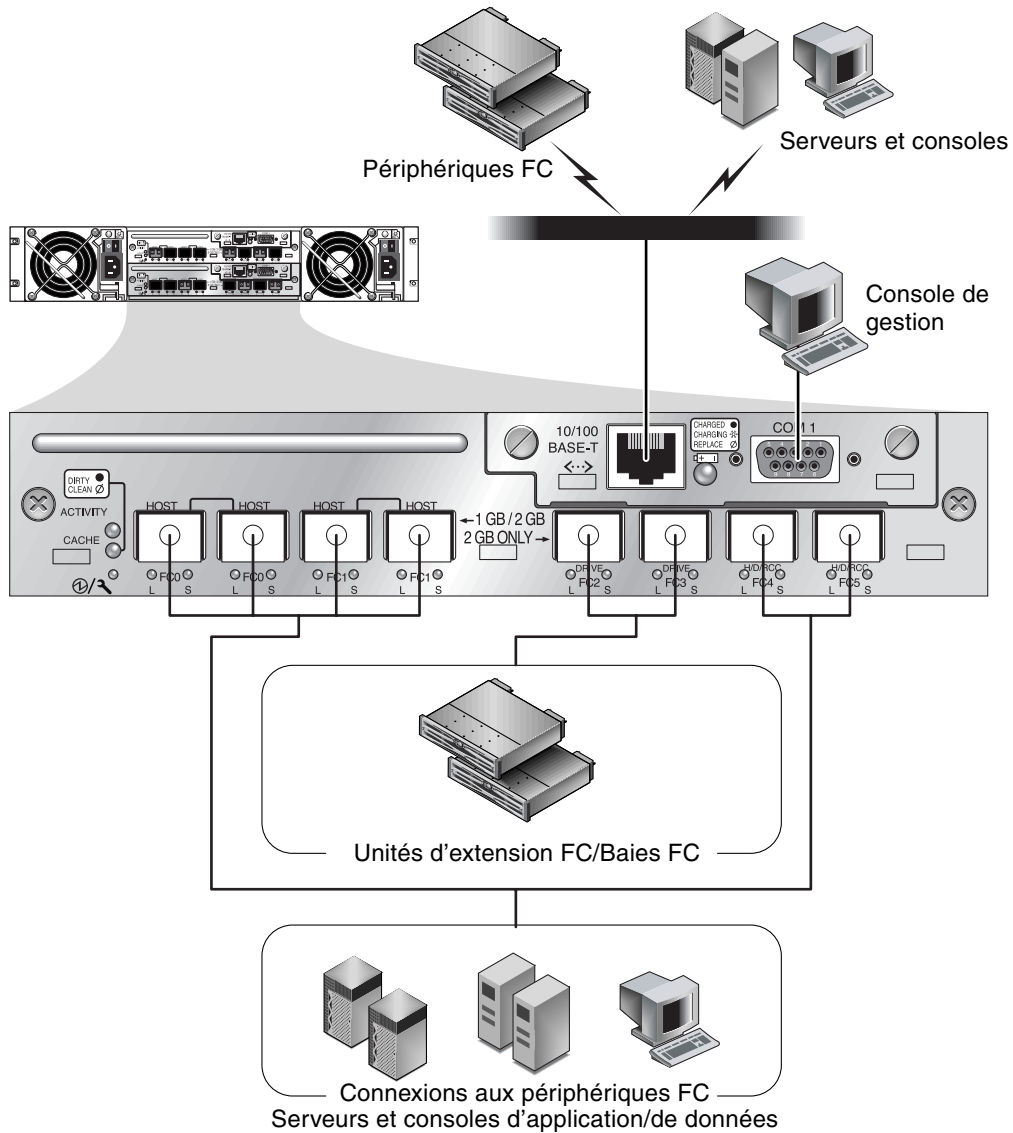
FIGURE 4-4 Connexions physiques à l'arrière d'une baie de disques Sun StorEdge 3511 FC à deux contrôleurs
