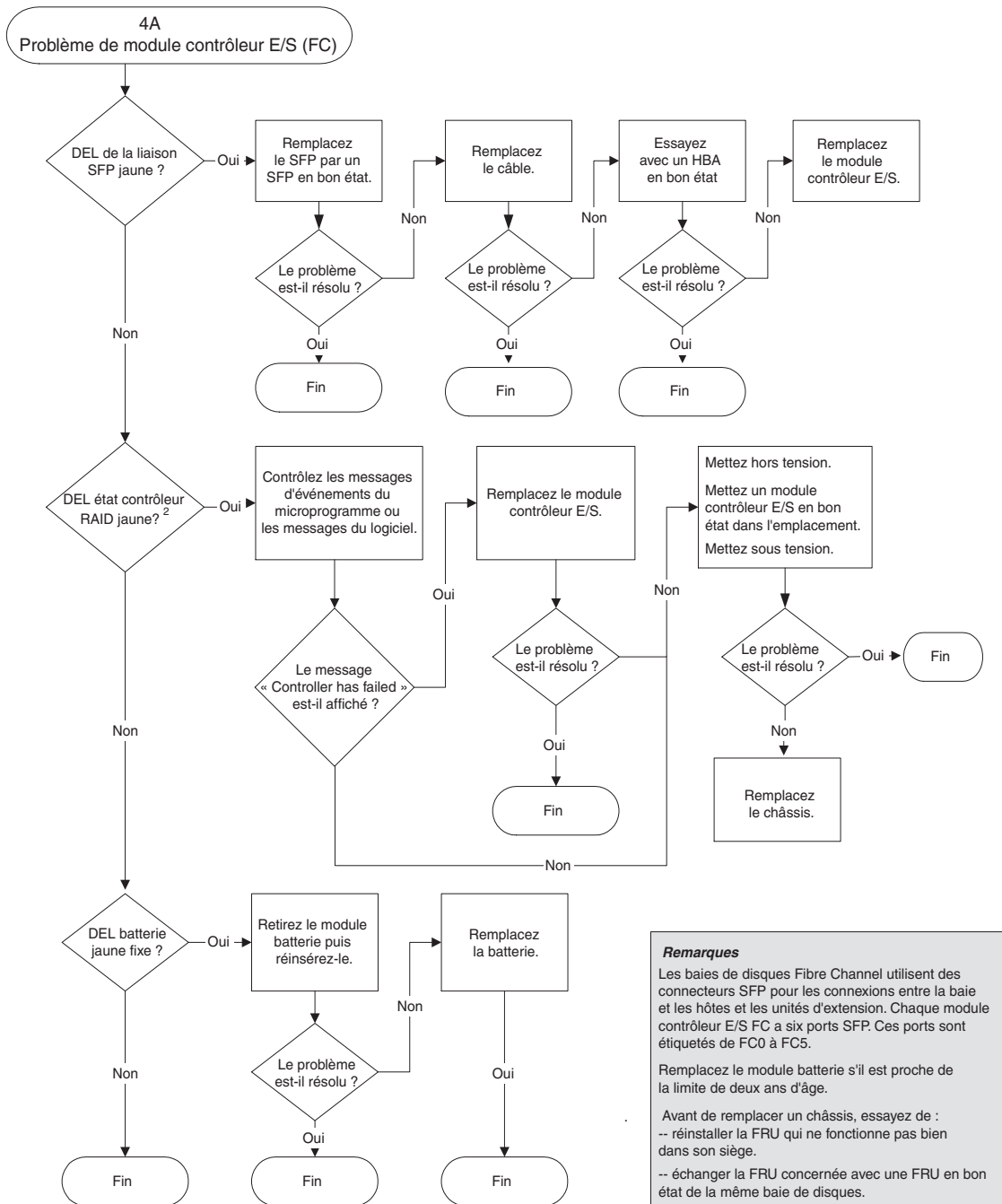
FIGURE 9-14 Organigramme d'un module contrôleur E/S
