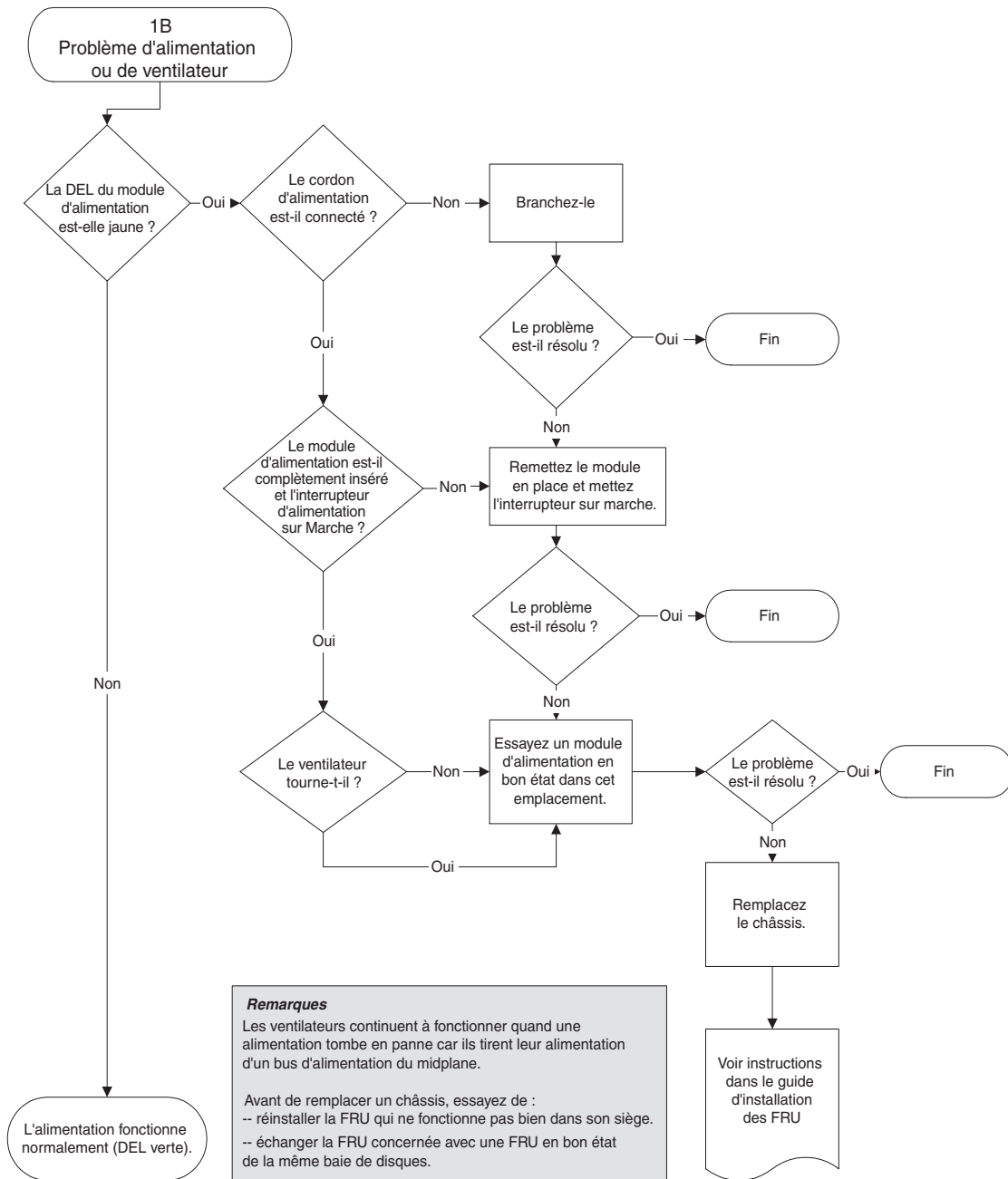
FIGURE 9-7 Organigramme du module de ventilation et d'alimentation, 2/2
