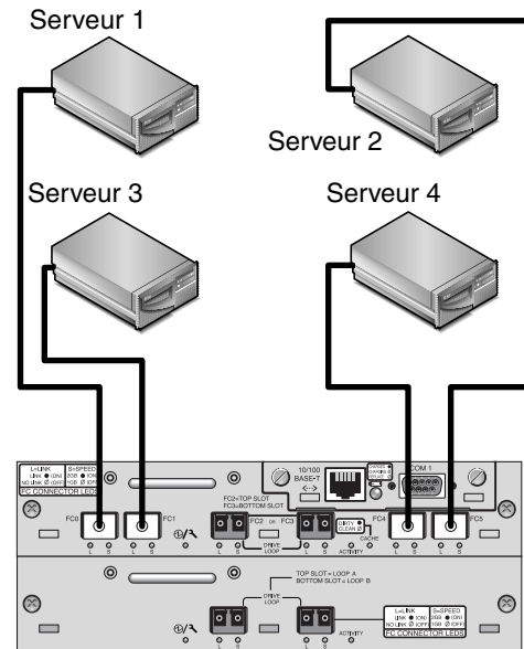
FIGURE 5 Connexions DAS non redondantes d'une baie Sun StorEdge 3510 FC
