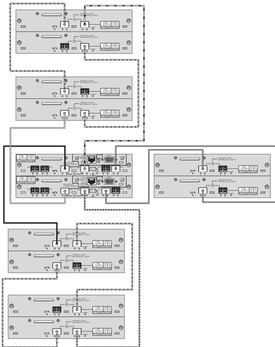
FIGURE 21 Configuration d'une baie Sun StorEdge 3510 FC avec cinq unités d'extension
