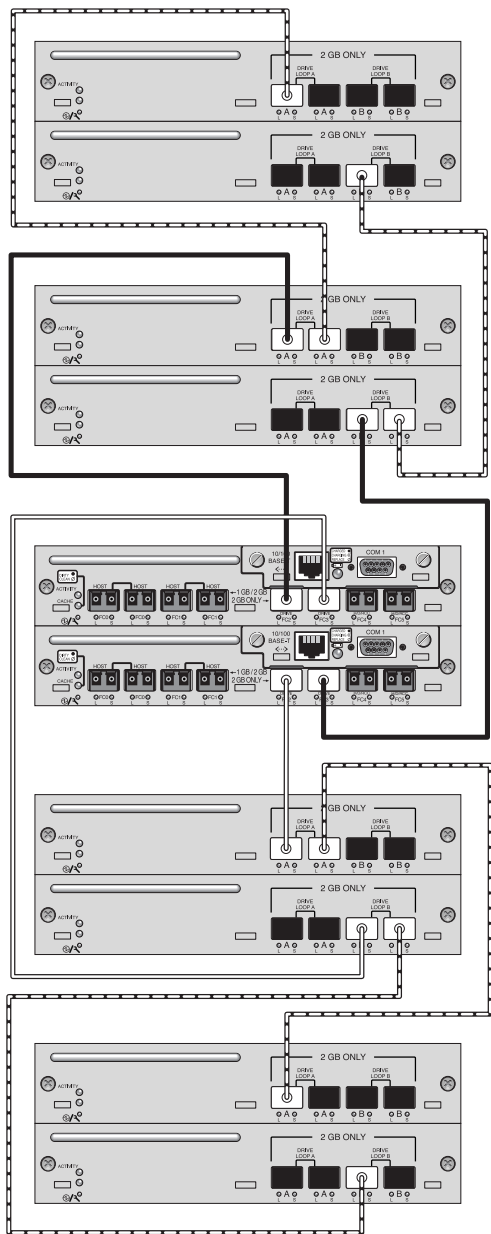
FIGURE 28 Configuration d'une baie Sun StorEdge 3511 SATA avec quatre unités d'extension
