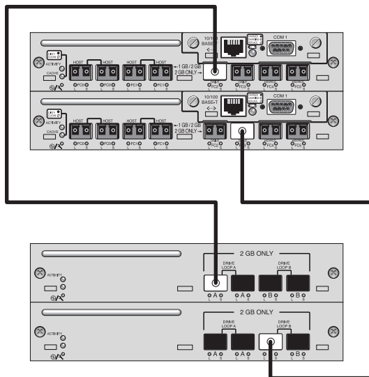
FIGURE 25 Configuration d'une baie Sun StorEdge 3511 SATA avec une unité d'extension
