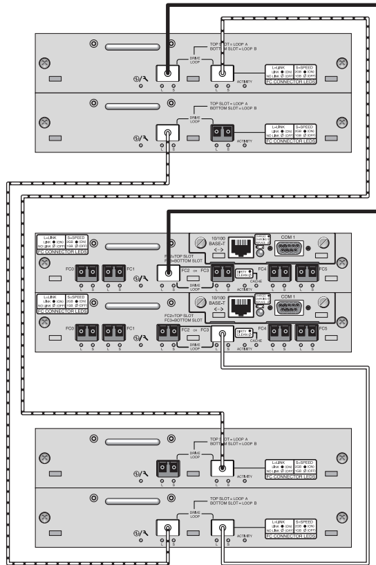
FIGURE 18 Configuration d'une baie Sun StorEdge 3510 FC avec deux unités d'extension
