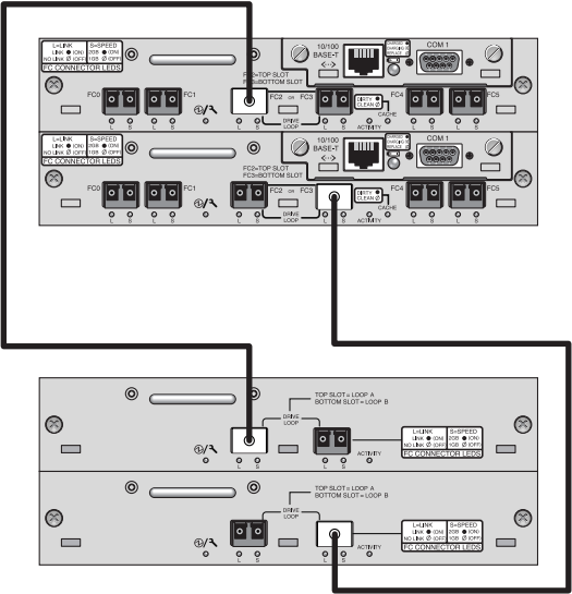
FIGURE 17 Configuration d'une baie Sun StorEdge 3510 FC avec une unité d'extension
