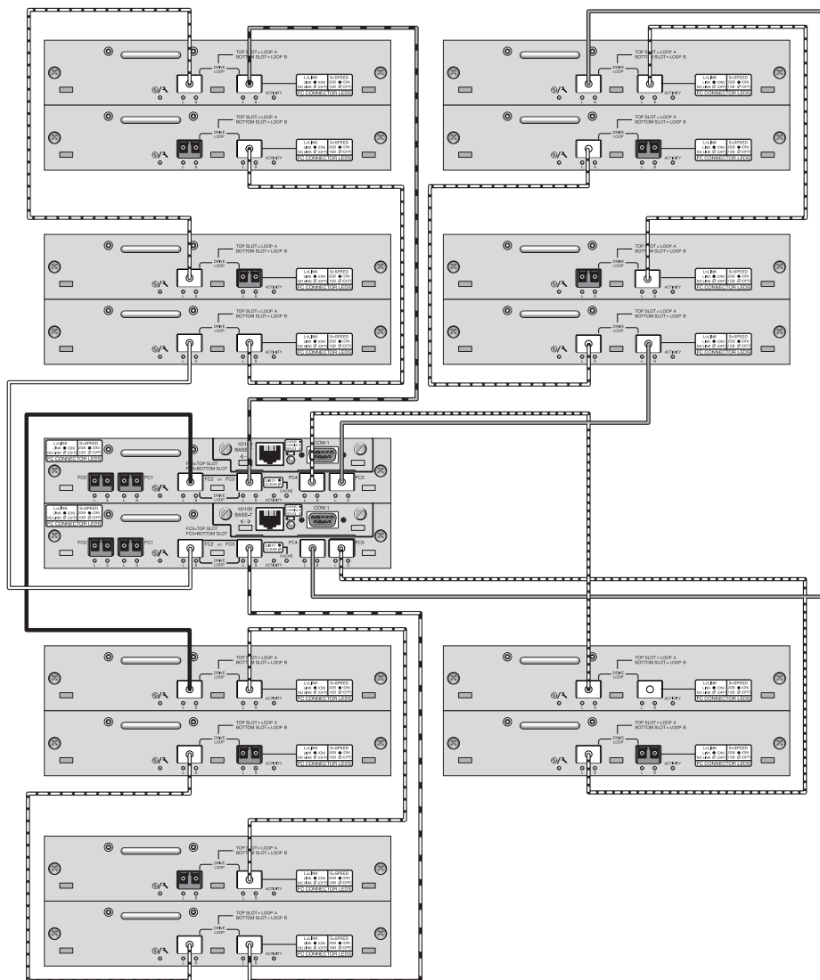
FIGURE 23 Configuration d'une baie Sun StorEdge 3510 FC avec sept unités d'extension
