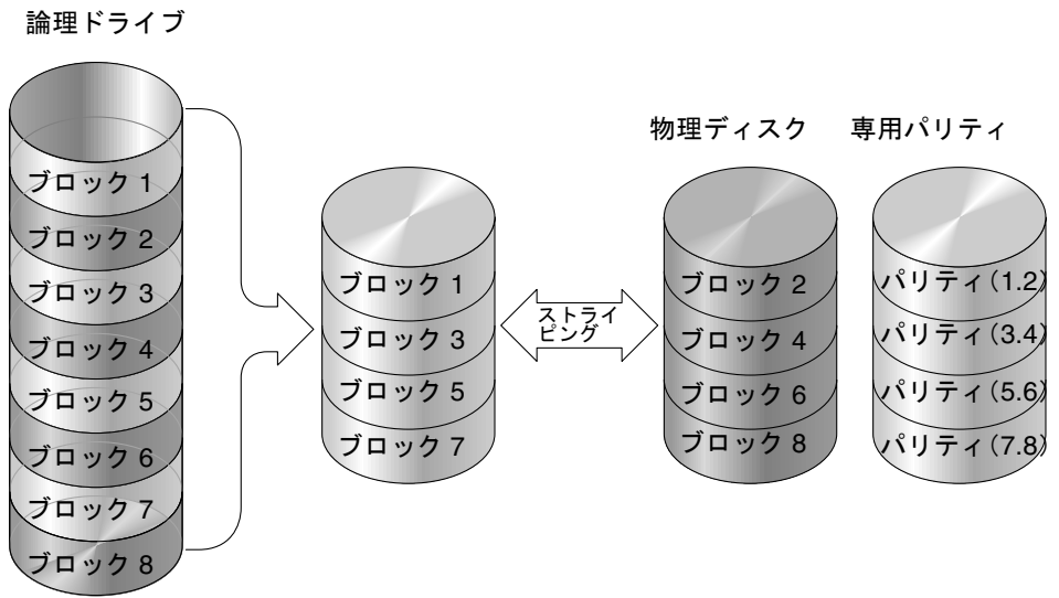
図 1-9 RAID 3 構成
