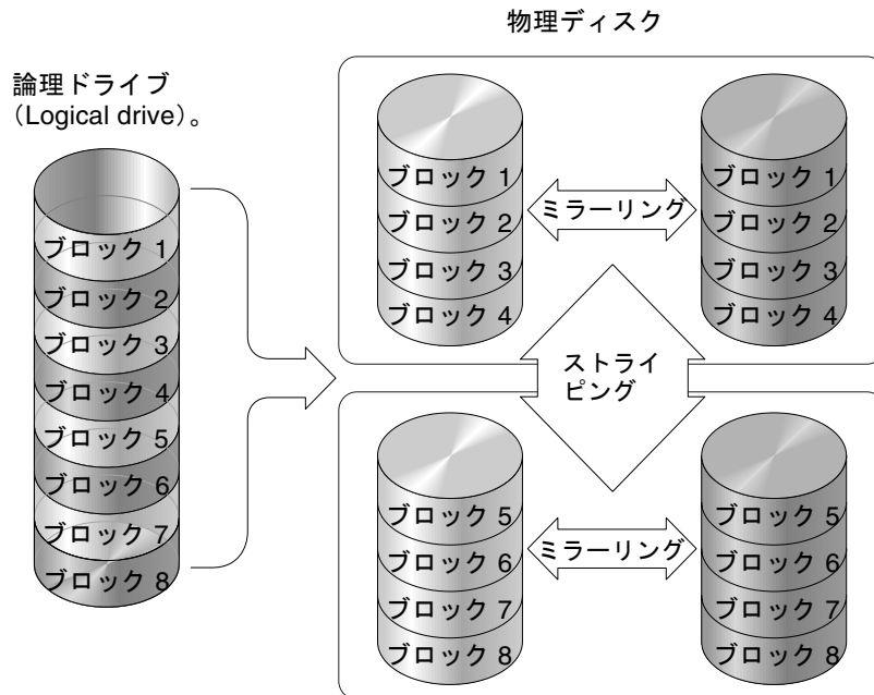
図 A-9 RAID 1+0 構成
