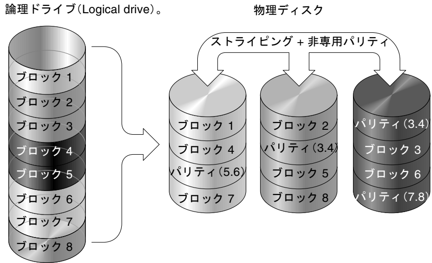
図 A-11 RAID 5 構成
