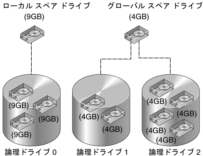
図 A-14 ローカル スペア ドライブとグローバル スペア ドライブの混在
