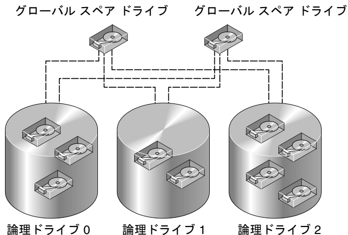
図 A-13 グローバル スペア
