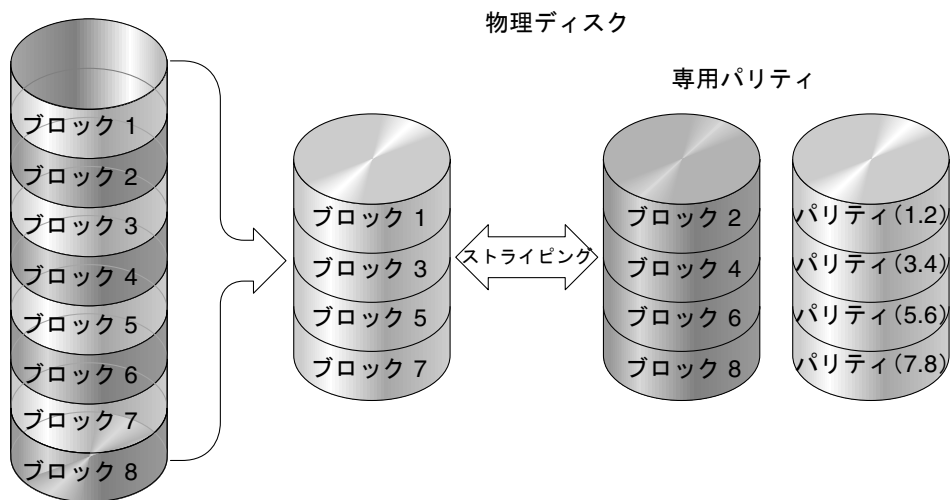
図 A-10 RAID 3 構成
