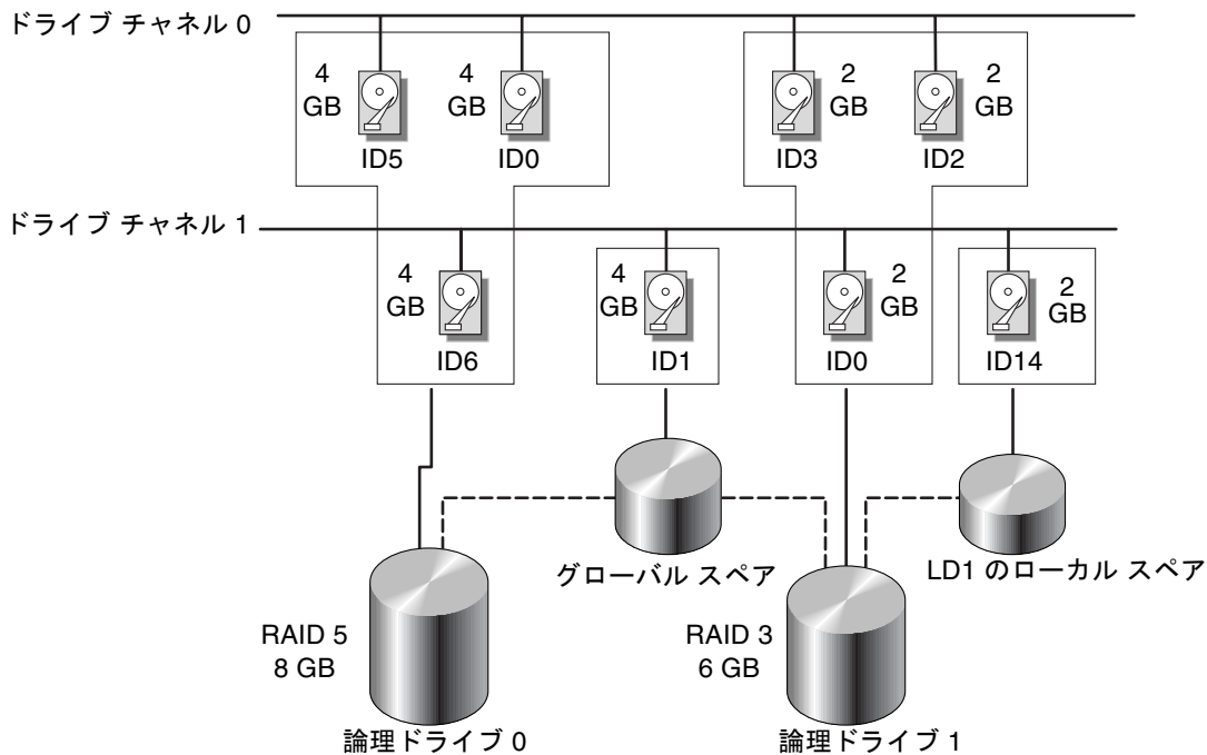
図 A-3 論理ドライブ構成内のドライブの割り当て
