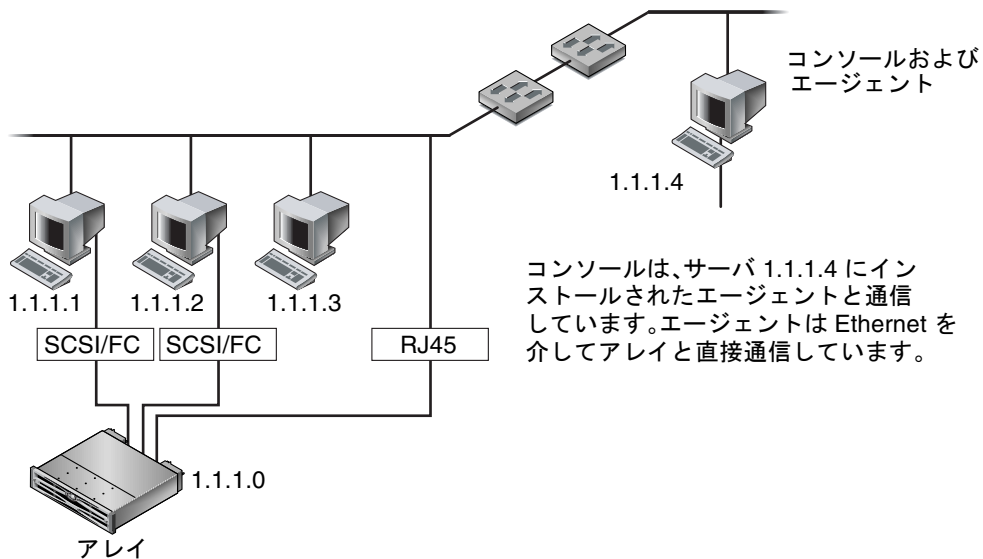
図 9-2 アウトオブバンドストレージ管理
