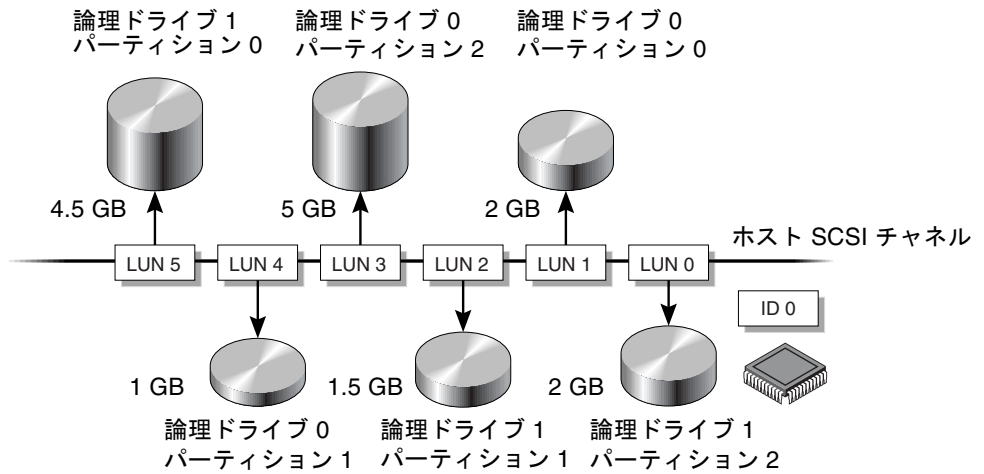
図 A-6 パーティションを ID 下の LUN にマップする
