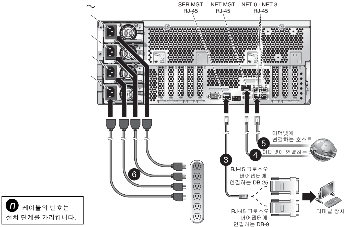
그림 2 서버 연결
