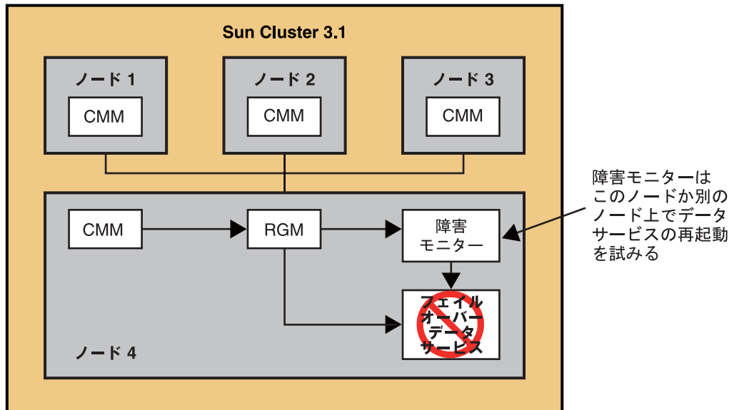
図 12-7 Sun Cluster 3.1 アーキテクチャーでのアプリケーション障害と復旧
