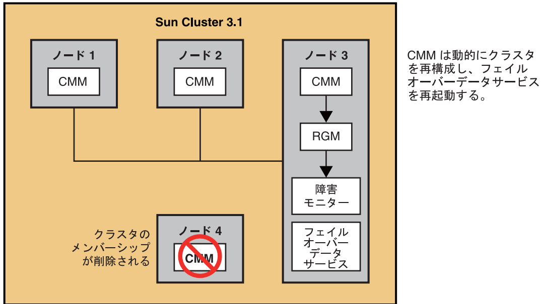
図 12-8 Sun Cluster 3.1 アーキテクチャでのサーバー障害と復旧
