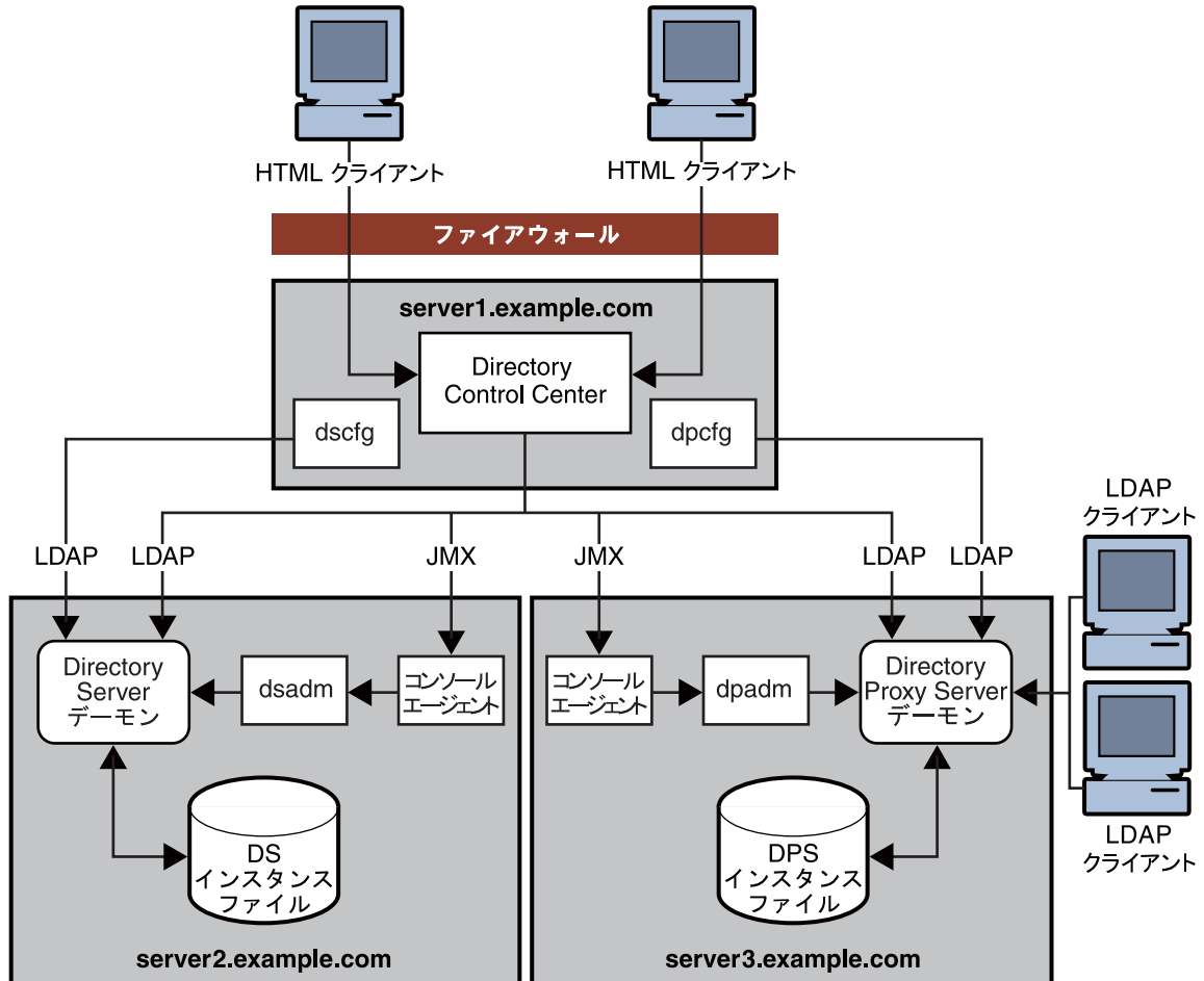
図 8-1 Directory Server Enterprise Edition の管理モデル
