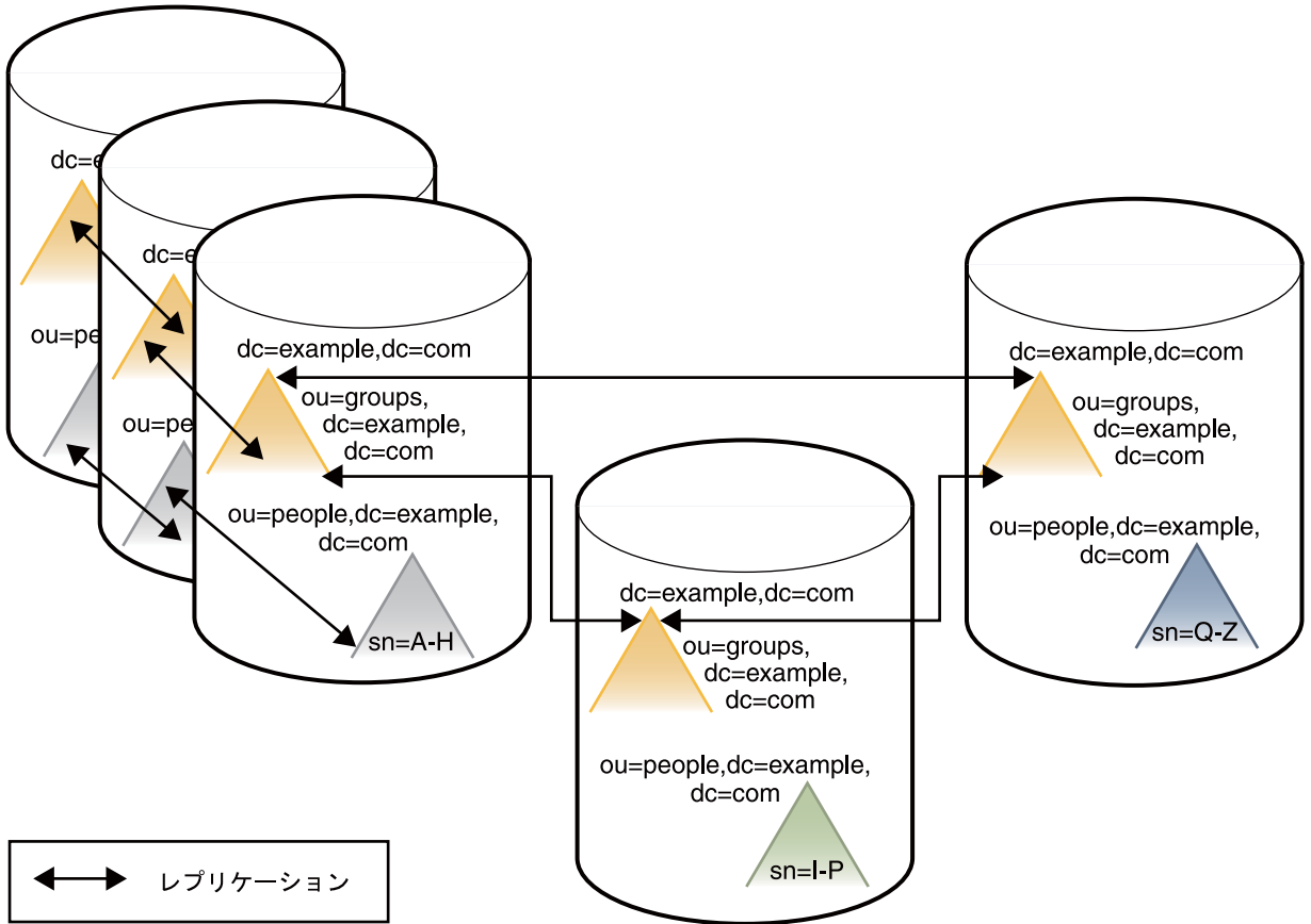
図 10-12 Directory Server 設定
