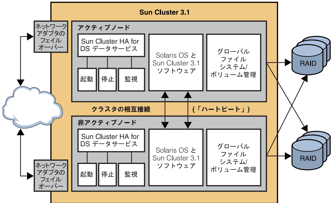
図 12-6 Sun Cluster 3.1 アーキテクチャ
