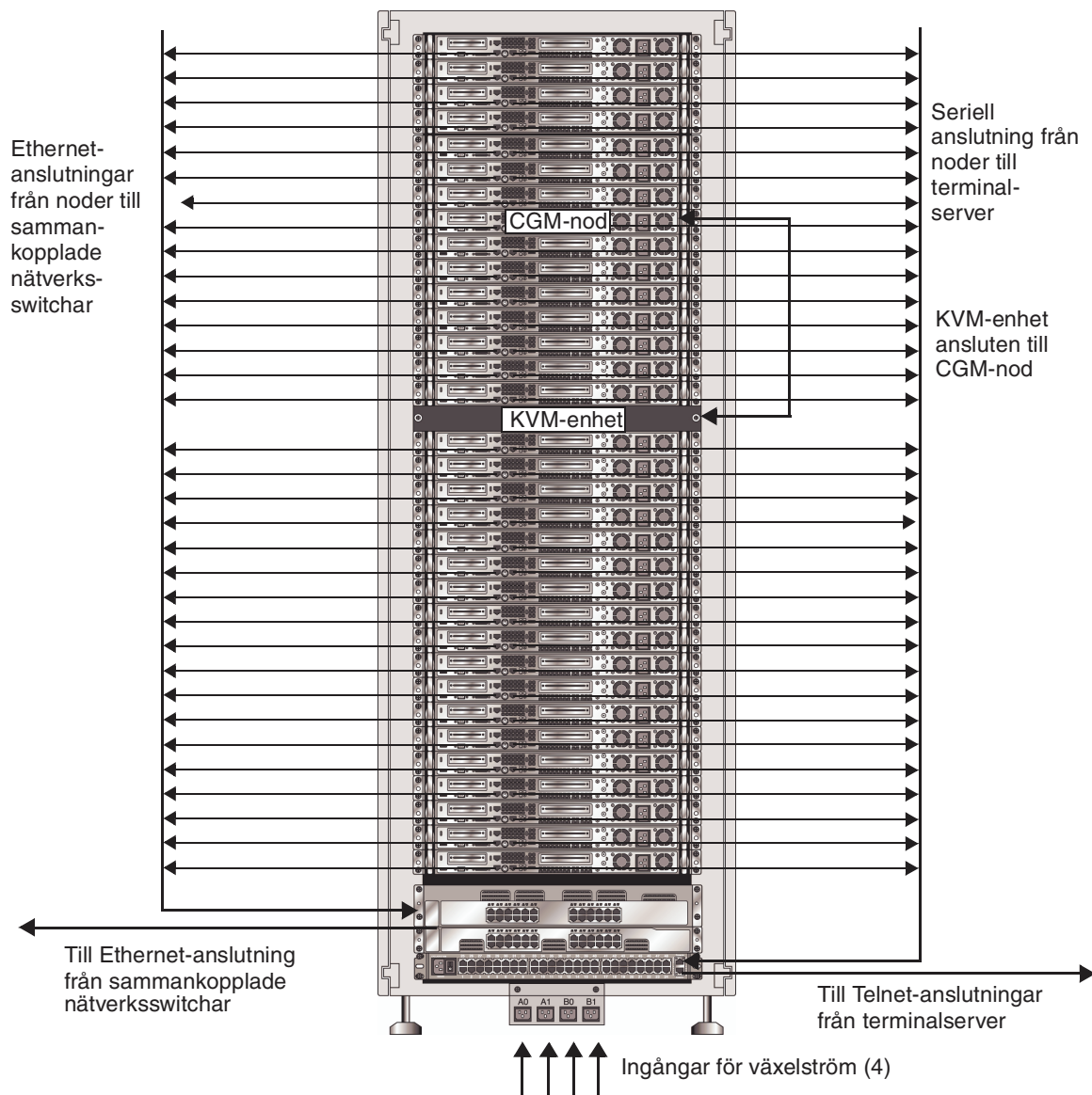
BILD 1-3 Kabelldiagram för ett rack, baksida
