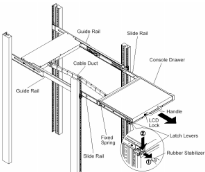
Схема выдвигения скользящего модуля
