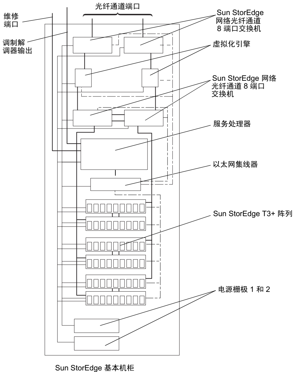
图 3-7 Sun StorEdge 6910 存储系统缆线连接
