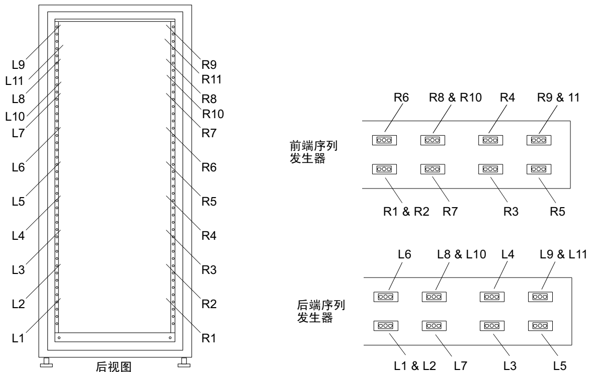
图 6-6 电源线分布
