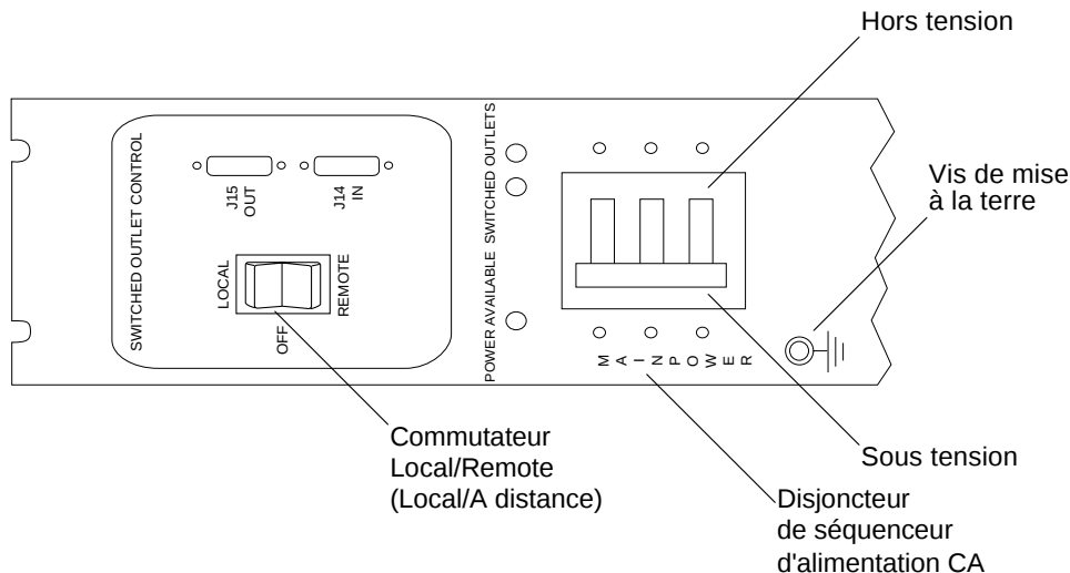
FIGURE 4-6 Panneau de contrôle d'un séquenceur d'alimentation CA
