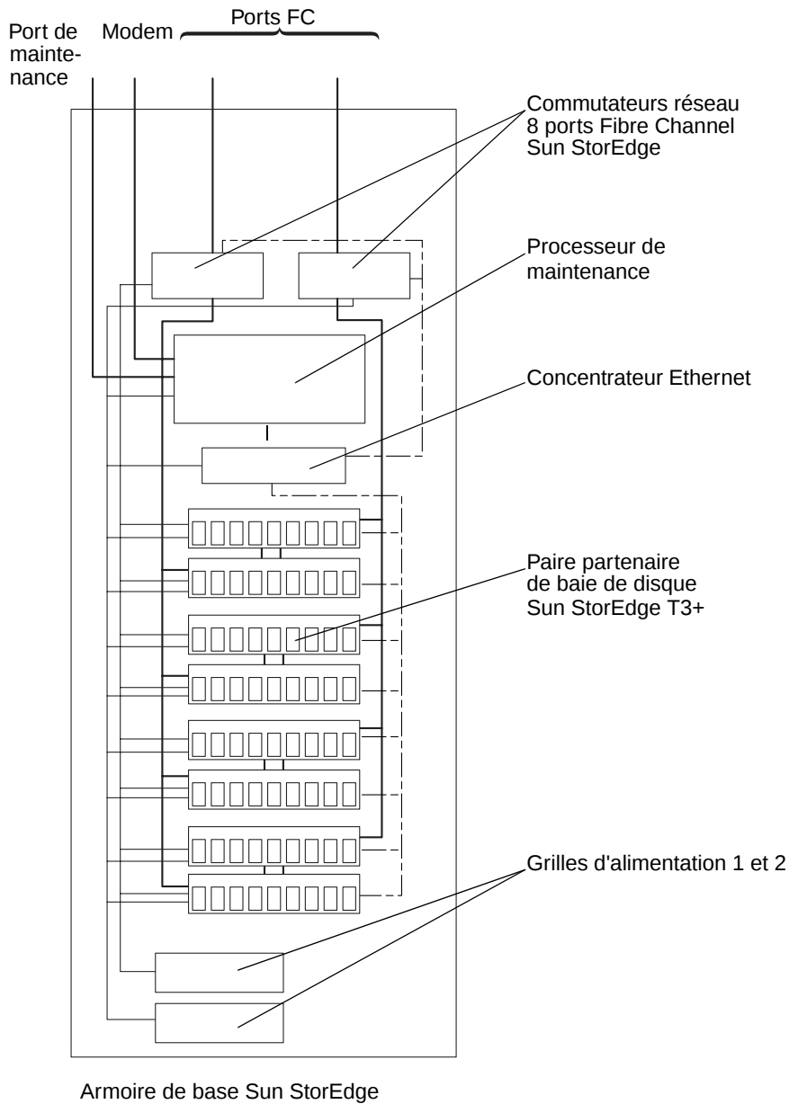
FIGURE 8-1 Câblage du système de stockage Sun StorEdge 3910
