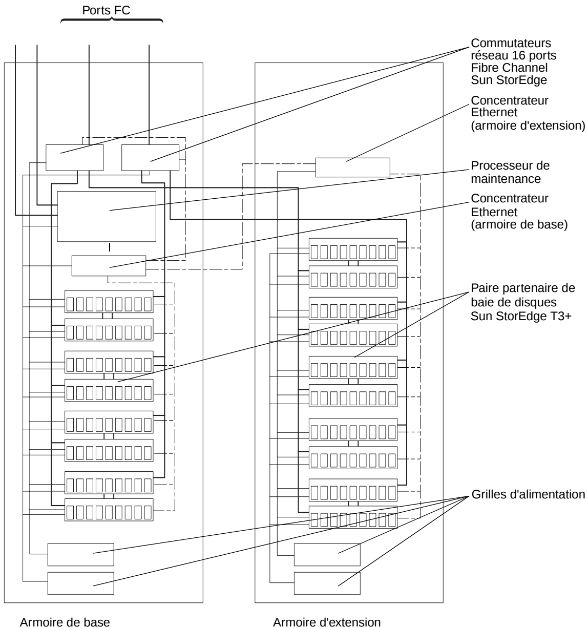
FIGURE 8-3 Câblage du système de stockage Sun StorEdge 3960
