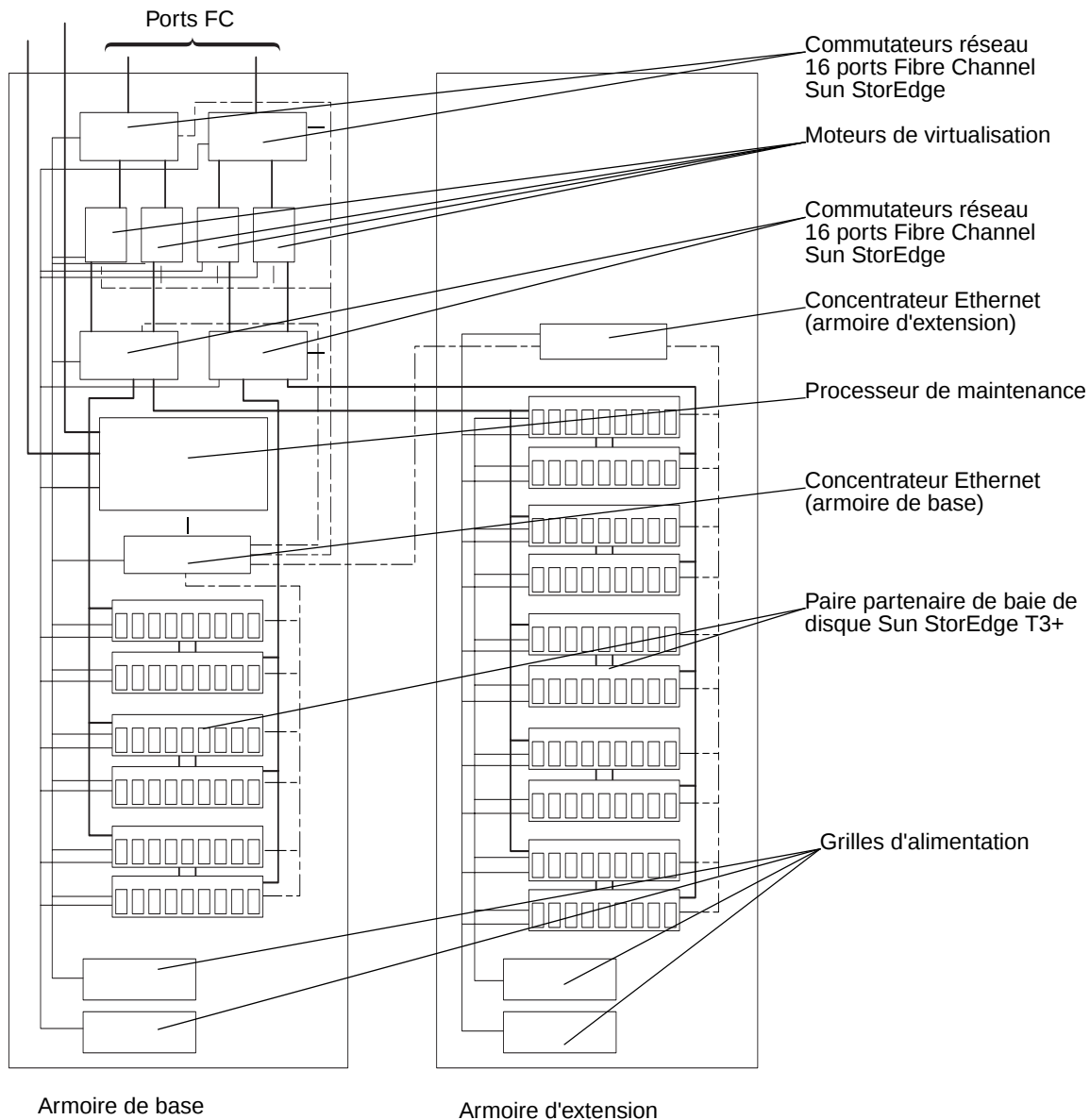
FIGURE 3-4 Câblage du système de stockage Sun StorEdge 6960
