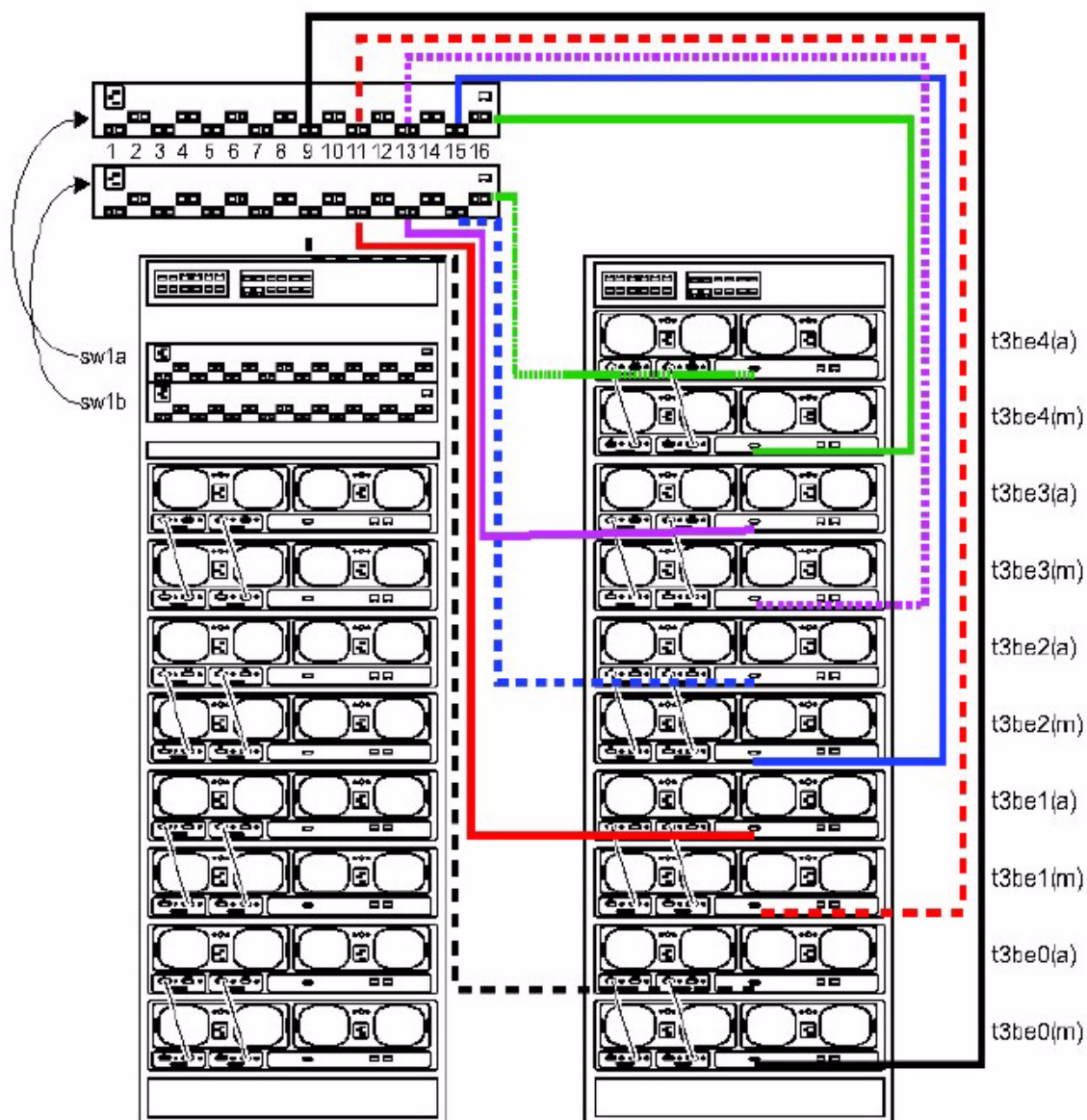
FIGURE 3-1 Câblage de l'armoire d'extension Sun StorEdge 3960
