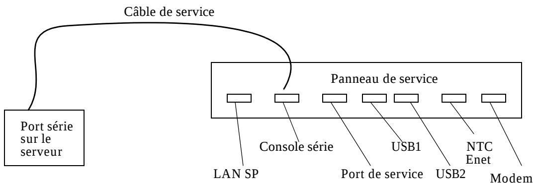
FIGURE 5-1 Connexion du câble de service à un serveur
