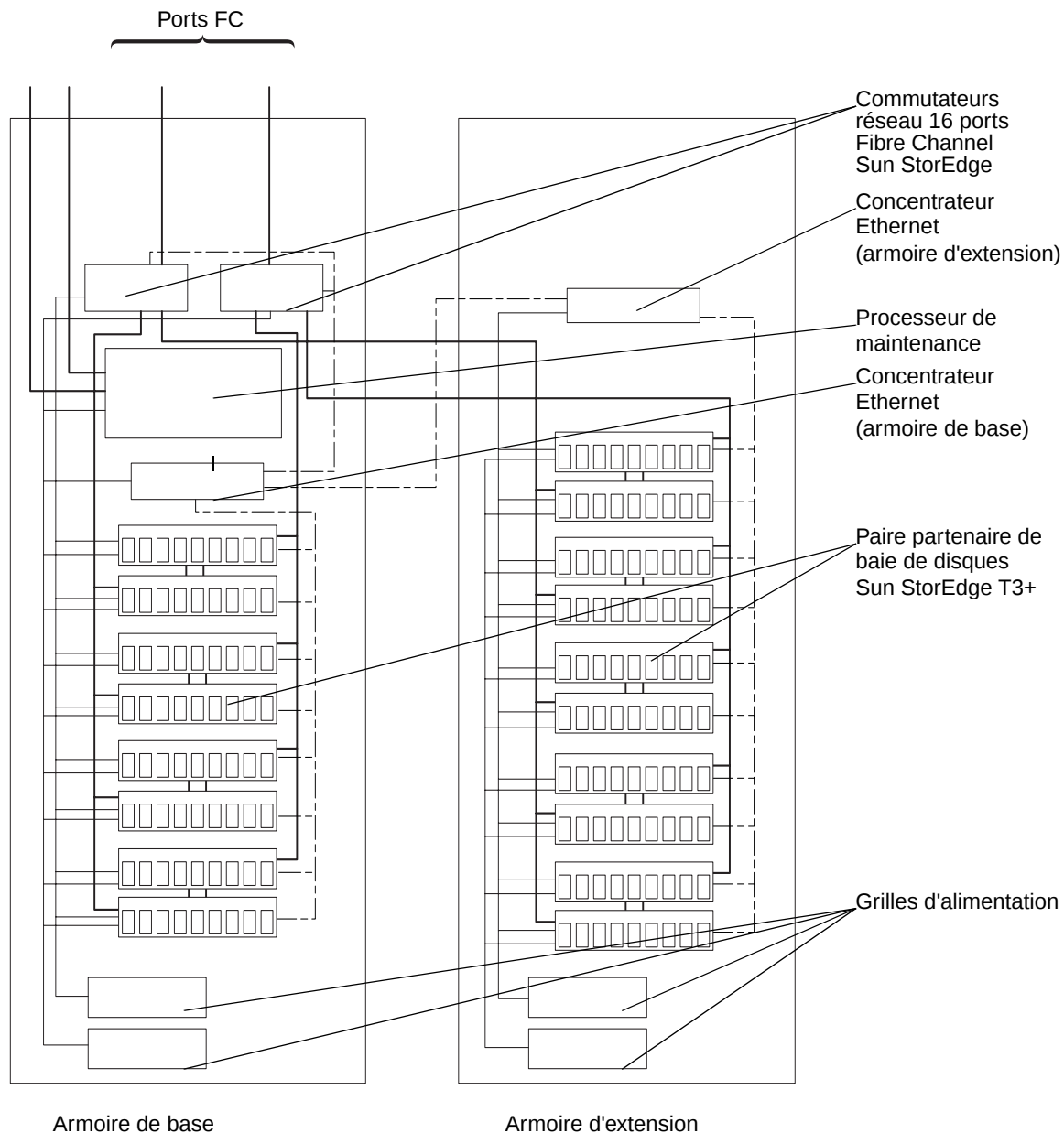
FIGURE 3-2 Câblage du système de stockage Sun StorEdge 3960
