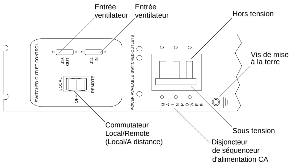
FIGURE 4-2 Panneau de contrôle du séquenceur d'alimentation
