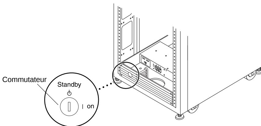
FIGURE 4-5 Emplacement du commutateur au bas du panneau avant
