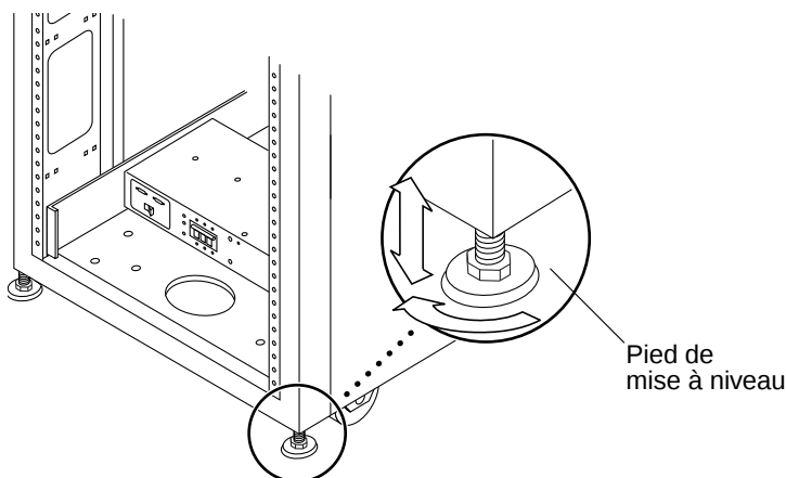
FIGURE 2-1 Pied de mise à niveau
