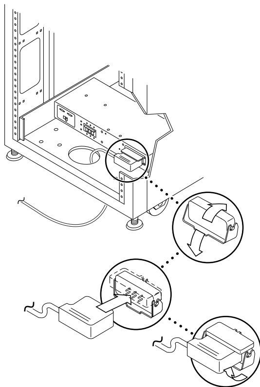
FIGURE 4-3 Connexion du cordon d'alimentation
