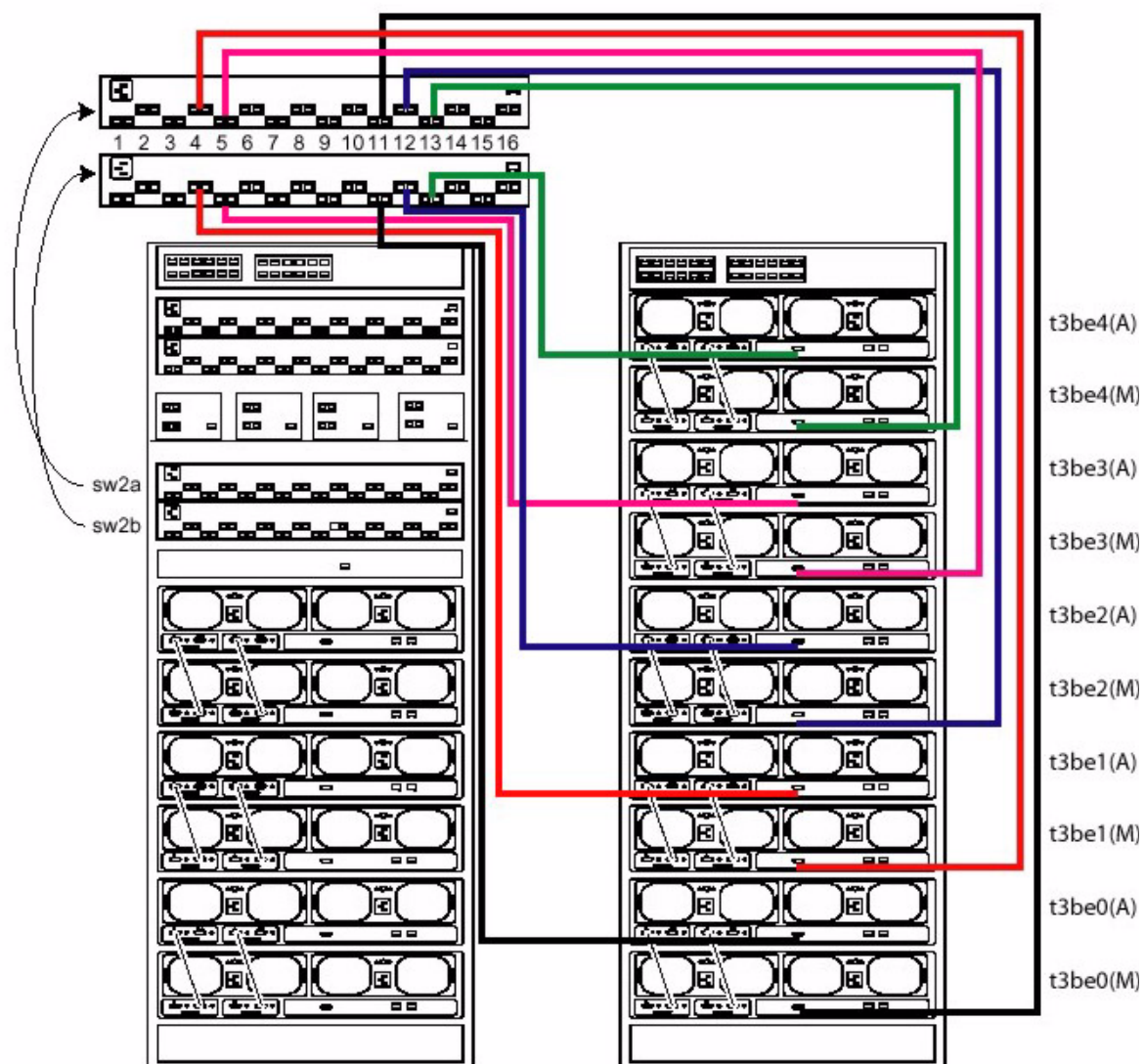
FIGURE 3-3 Câblage de l'armoire d'extension Sun StorEdge 6960
