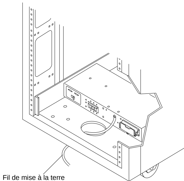
FIGURE 4-4 Connexion du fil de mise à la terre au séquenceur d'alimentation avant
