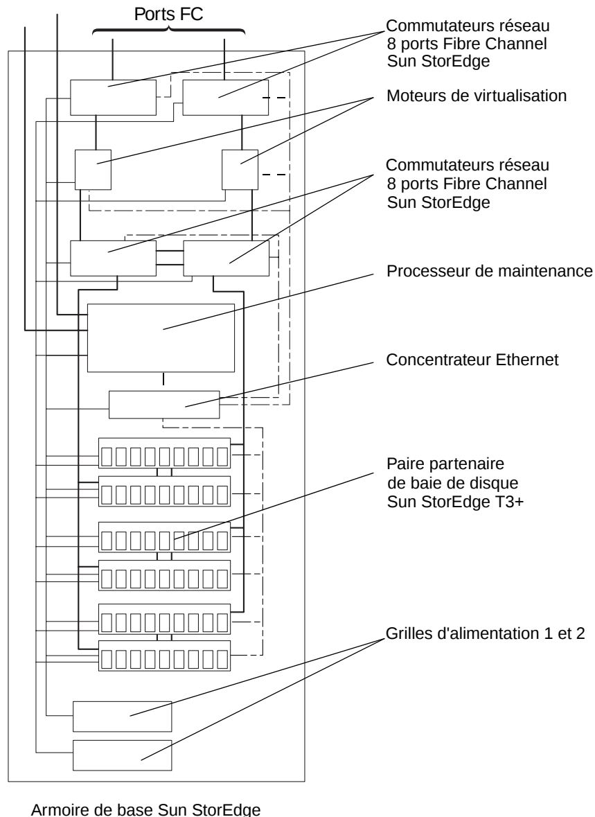
FIGURE 8-2 Câblage du système de stockage Sun StorEdge 6910
