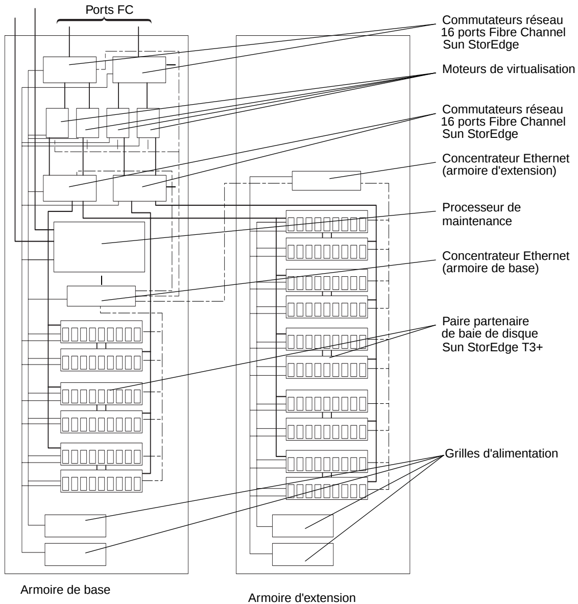
FIGURE 8-4 Câblage du système de stockage Sun StorEdge 6960
