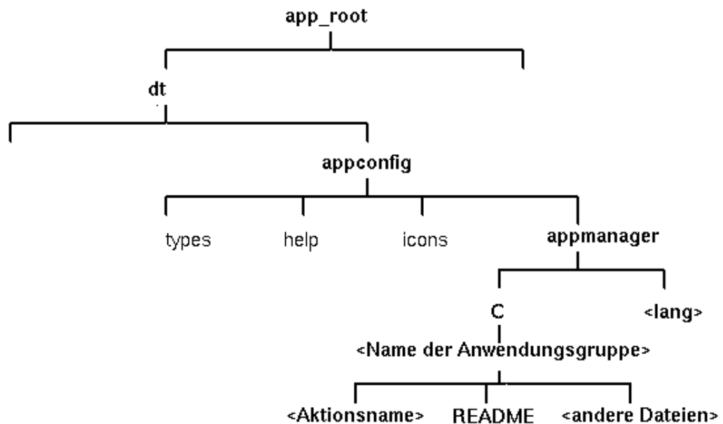
Abbildung 5-7 Das Verzeichnis appmanager
