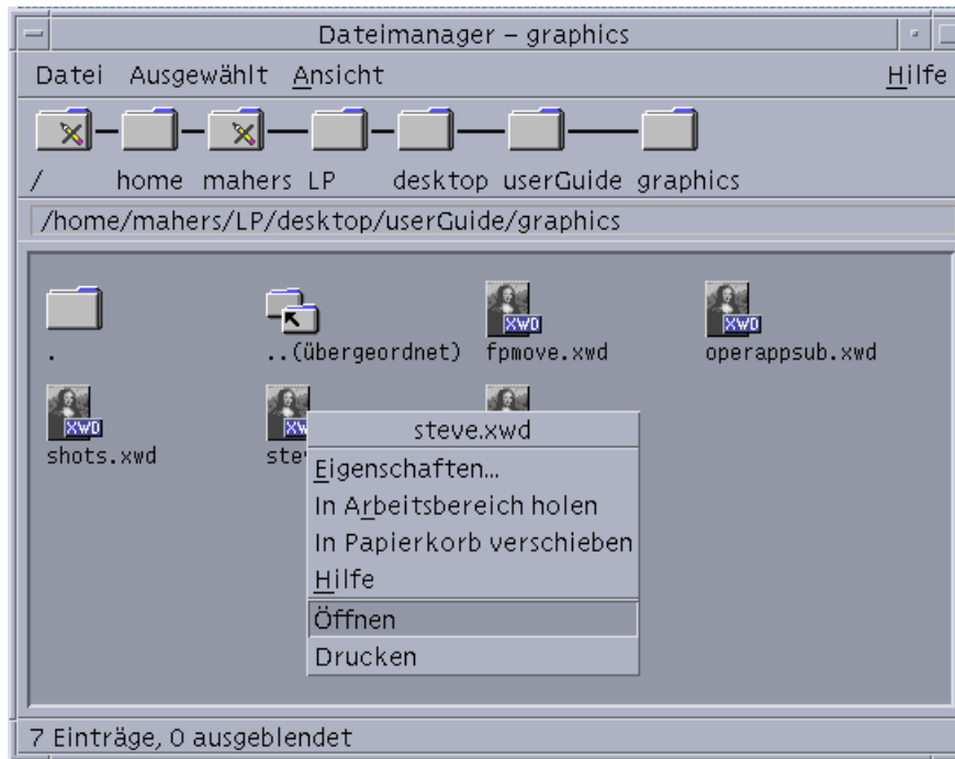
Abbildung 10-2 Aktion 'Öffnen' für Dateien des Datentyps XWD
