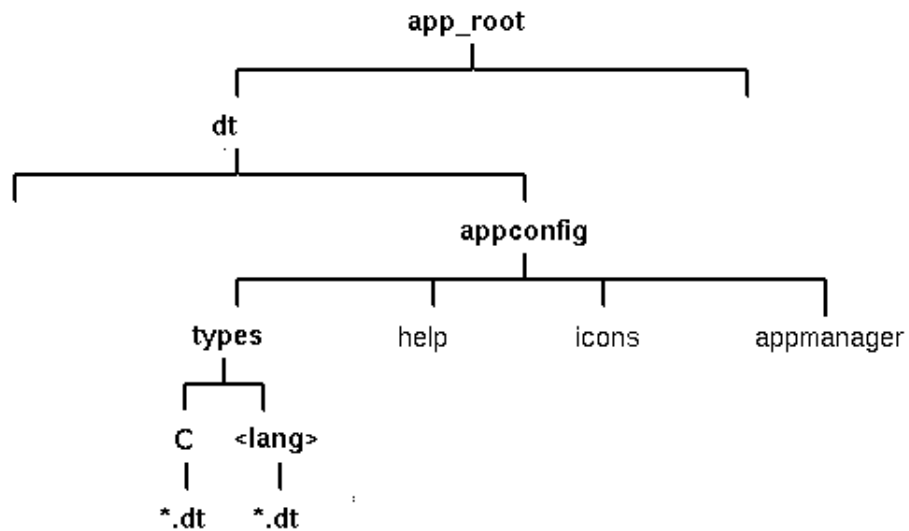
Abbildung 5-6 Definitionen für Aktionen und Datentypen
