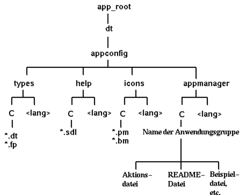
Abbildung 5-4 Ein Registrierungspaket unter einem Anwendungsstammverzeichnis
