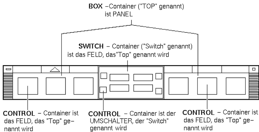
Abbildung 15-2 Hauptsteuerbereich-Container
