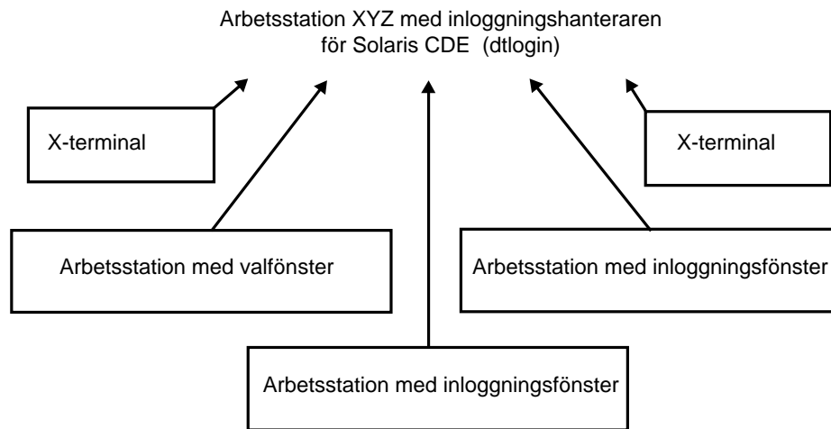
Figur 6-1 Nätverksanslutna skrivbord
