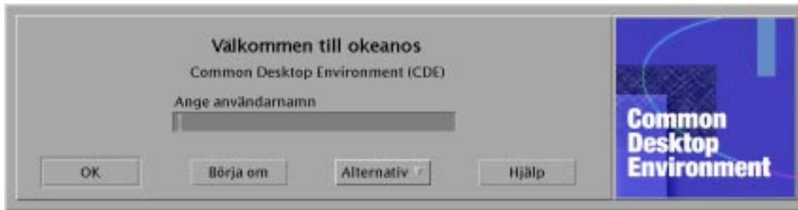
Figur 1-2 Inloggningsbilden
