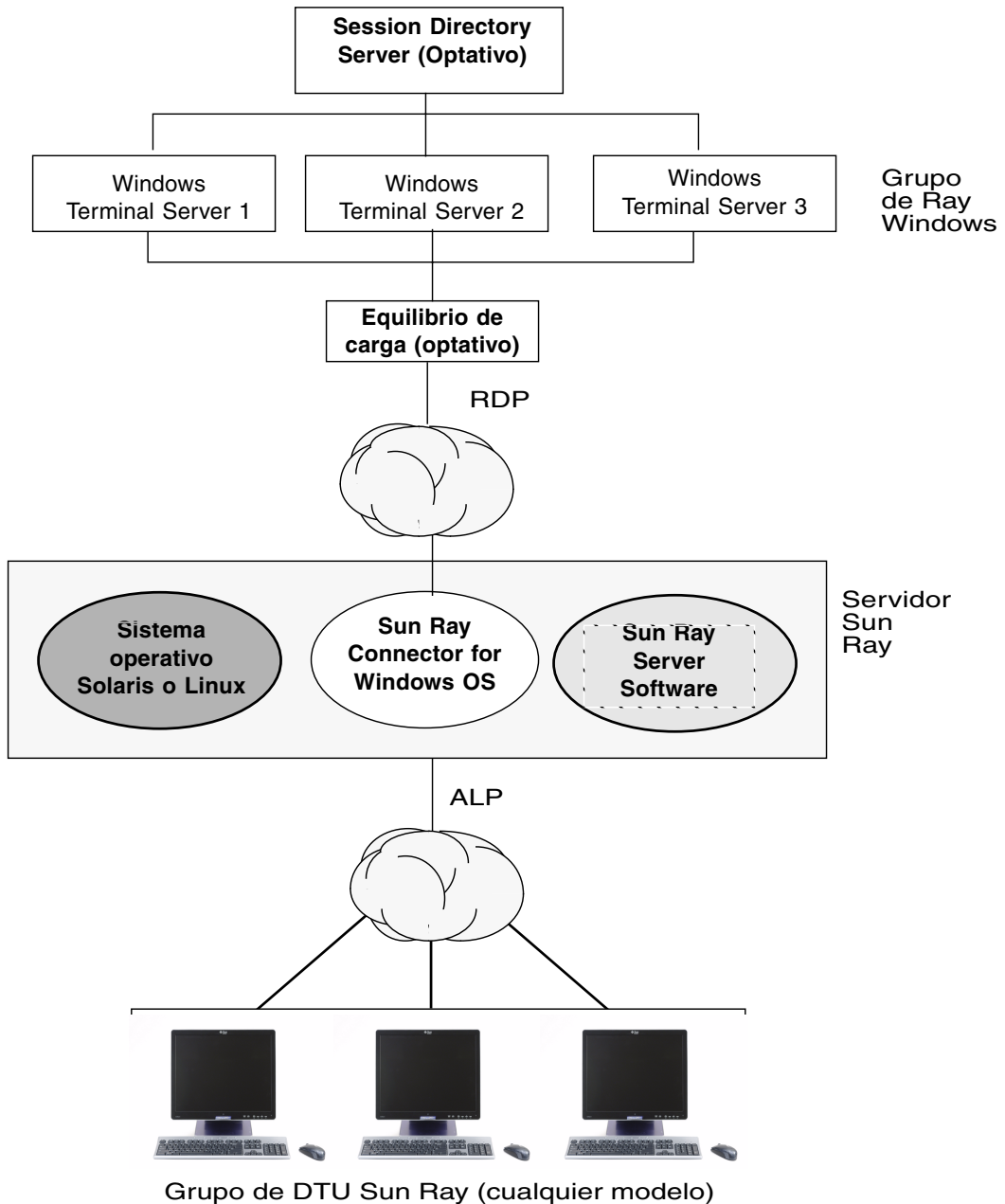
FIGURA 1 Conexión entre Sun Ray y Windows a través de los protocolos RDP y ALP, mostrando un servidor Session Directory y equilibrio de carga
