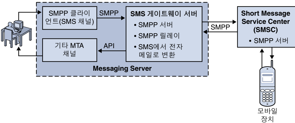
그림 D-1 단방향 및 양방향 SMS의 논리적 흐름
