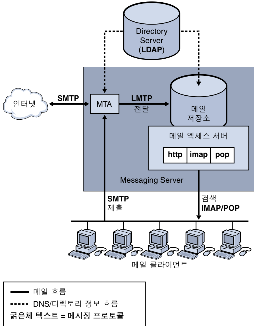
그림 8-1 Messaging Server, 단순화된 구성 요소 보기 (Communications Express는 표시되지 않음)
