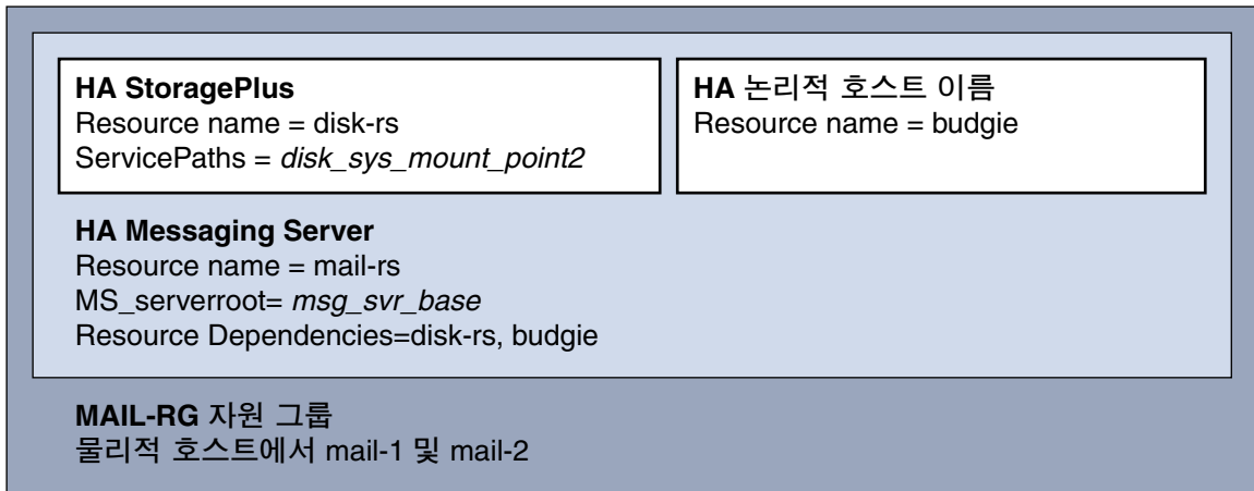
그림 3-3 간단한 Messaging Server HA 구성
