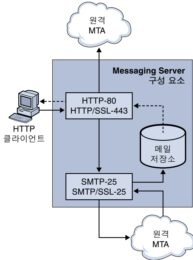
그림 5-1 HTTP 서비스 구성 요소
