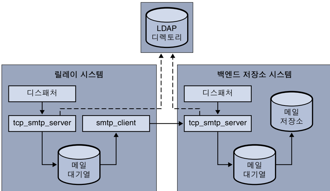
그림 15-1 LMTP를 사용하지 않는 2계층 배포
