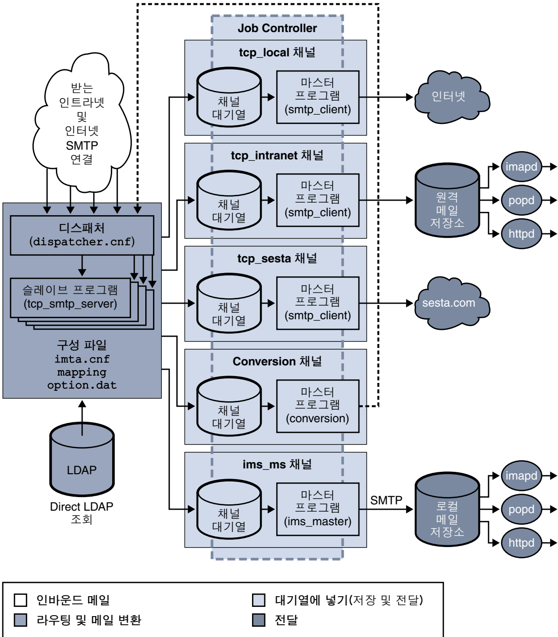
그림 8-2.MTA 구조
