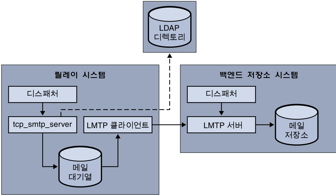
그림 15-2 LMTP를 사용하는 2계층 배포
