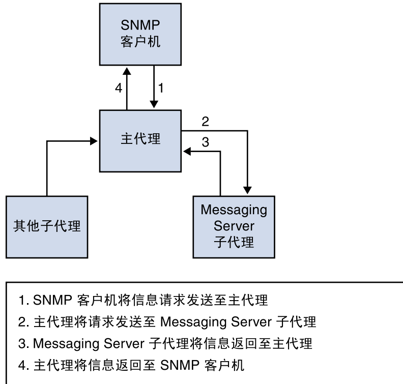
图 A-1 SNMP 信息流
