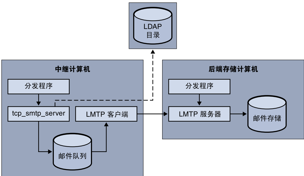
图 15-2 带有 LMTP 的两层部署
