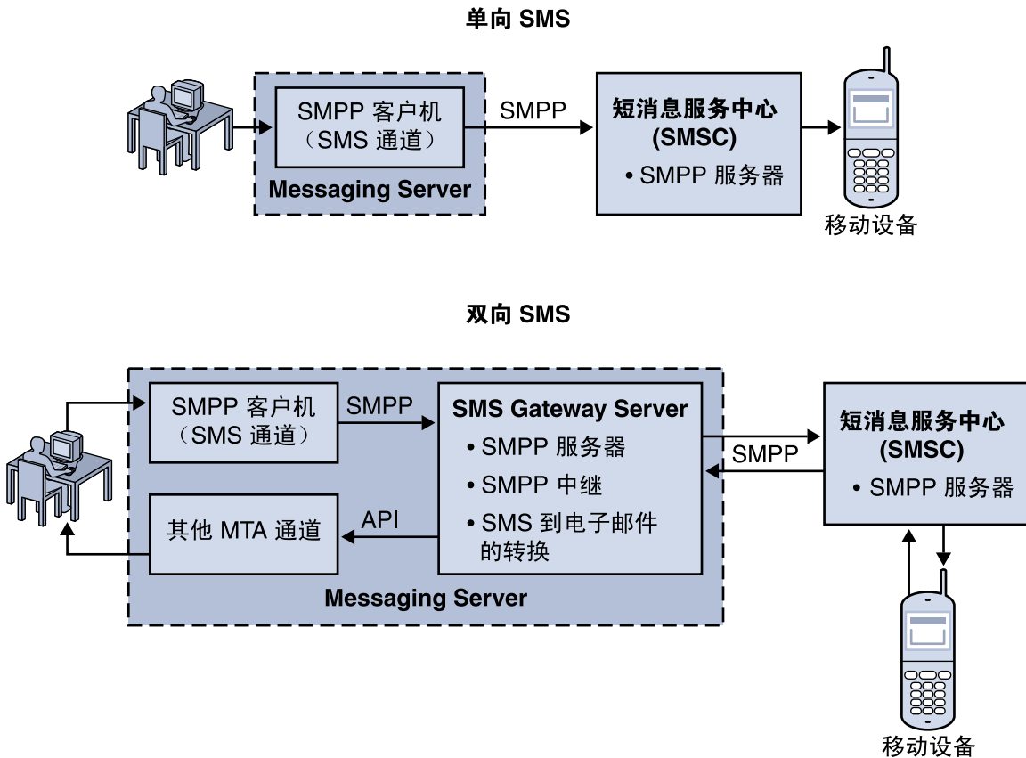
图 D-1 单向和双向 SMS 逻辑流
