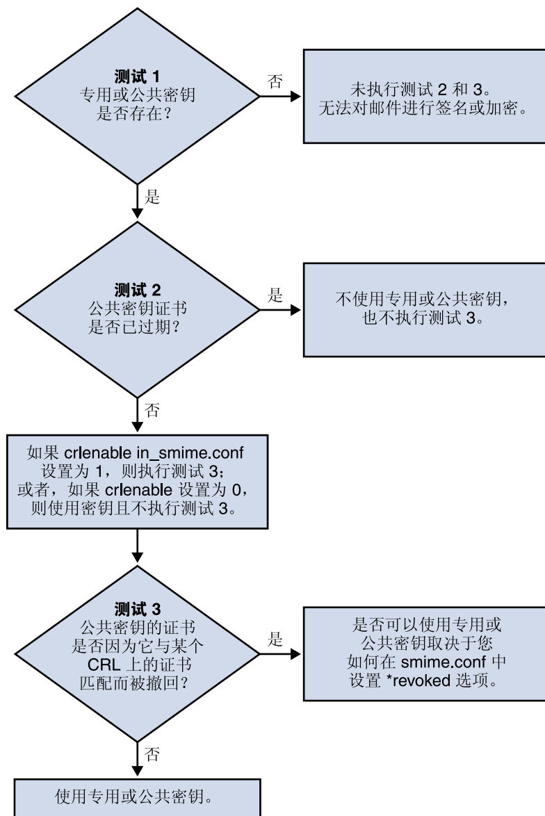
图 20-2 验证专用密钥和公共密钥。
