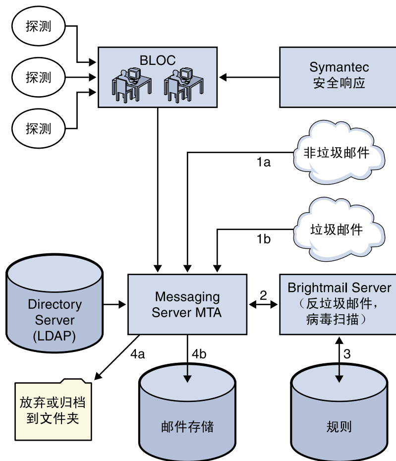
图 14-1 Brightmail 和 Messaging Server 体系结构
