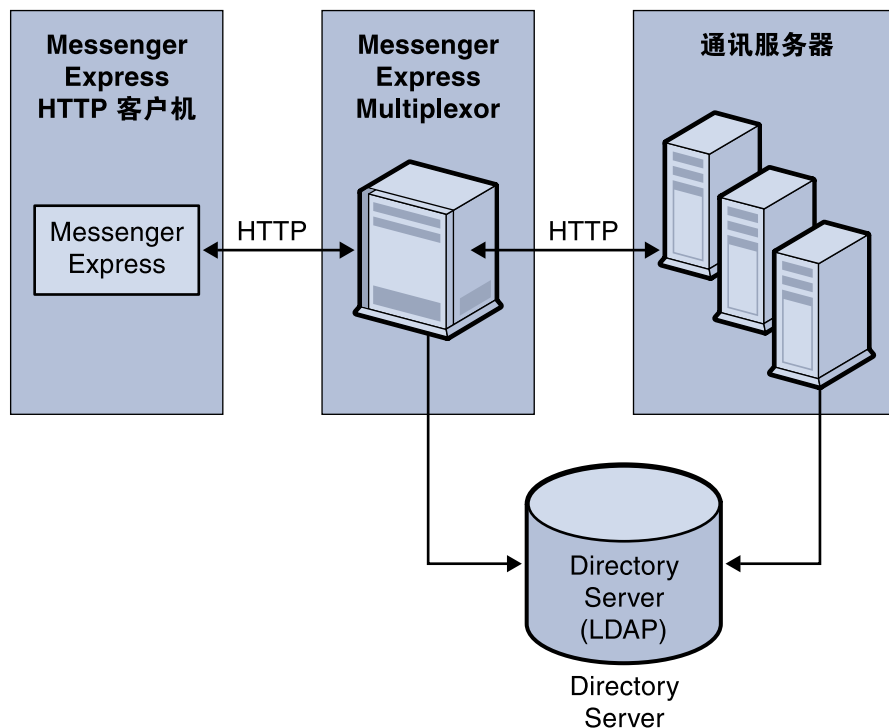
图 7-3 Messenger Express Multiplexor 概述
