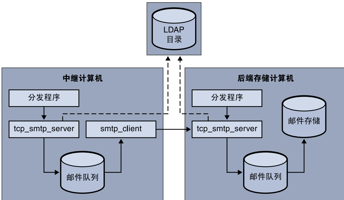
图 15-1 不带有 LMTP 的两层部署
