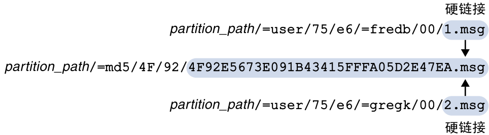
图 18-5 邮件存储摘要系统信息库
