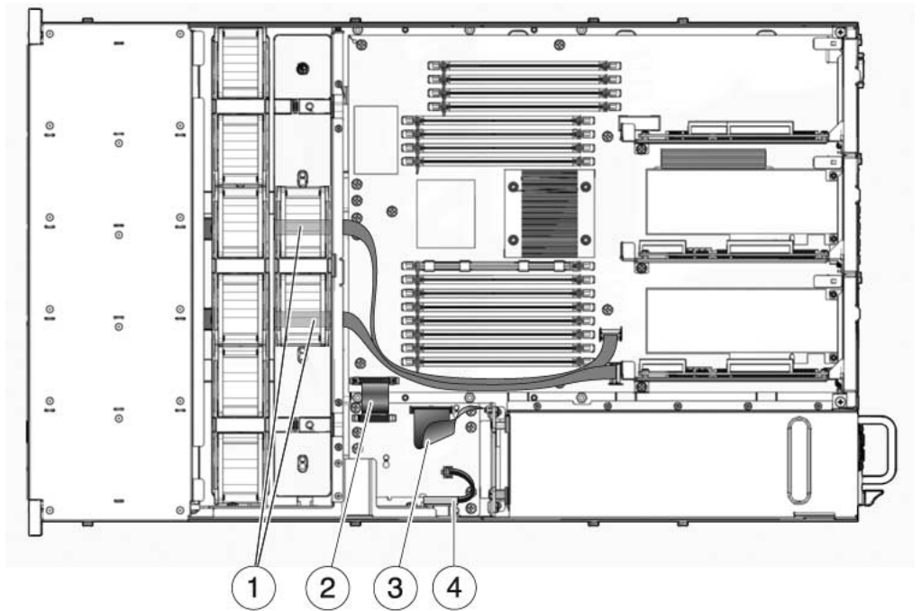
FIGURE A-12 Câbles (serveur Sun SPARC Enterprise T5220)
