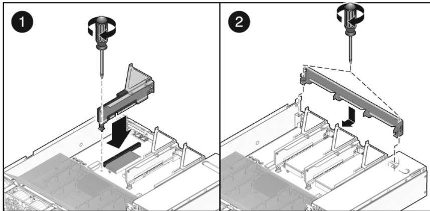
FIGURE 5-7 Installation d'une carte Riser PCIe/XAUI (serveur Sun SPARC Enterprise T5220)
