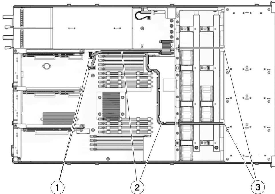
FIGURE A-6 Câbles HDD du contrôleur SAS intégré au backplane des unités de disque dur (Serveur Sun SPARC Enterprise T5120, capacité de 8 unités de disque dur)
