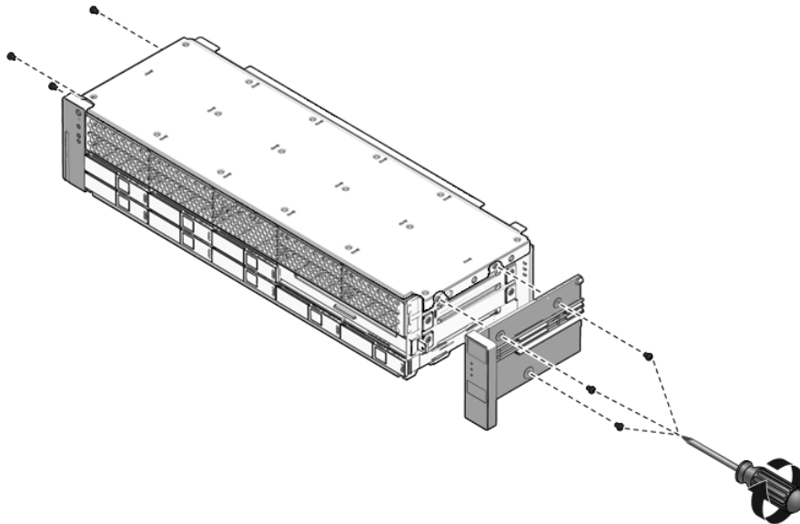
FIGURE 6-12 Installation de l'assemblage de voyants lumineux du panneau de contrôle (serveur Sun SPARC Enterprise T5220)
