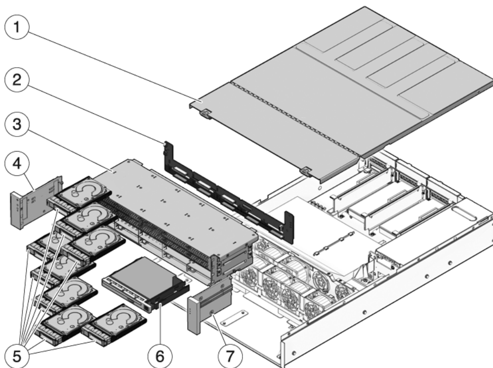
FIGURE A-9 Composants d'E/S (serveur Sun SPARC Enterprise T5220)
