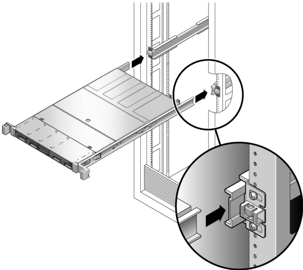
FIGURE 7-2 Réinstallation du serveur dans le rack (serveur Sun SPARC Enterprise T5120)
