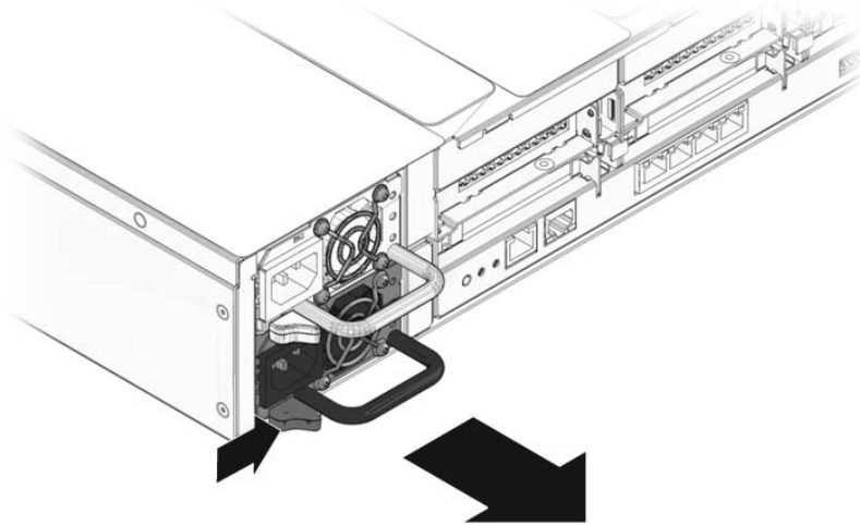
FIGURE 6-19 Retrait d'une unité d'alimentation (serveur Sun SPARC Enterprise T5220)
