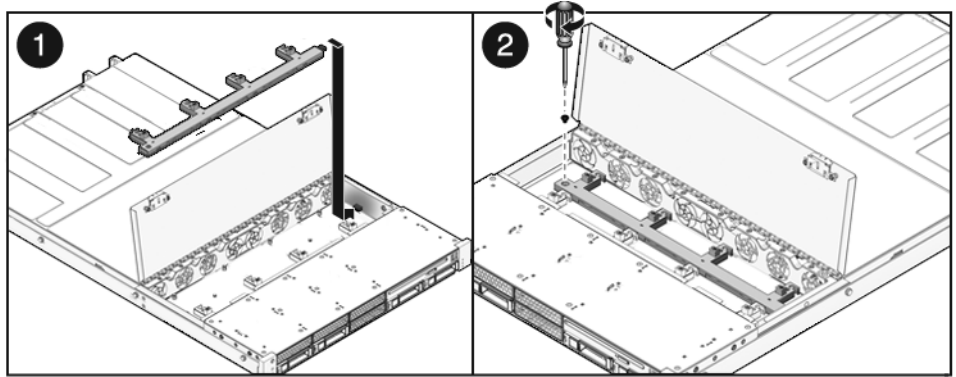
FIGURE 6-4 Installation d'une carte d'alimentation de ventilateur (serveur Sun SPARC Enterprise T5120)
