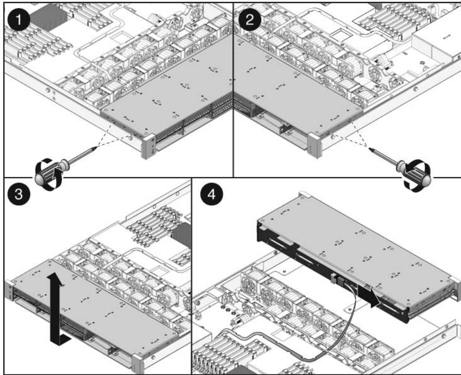
FIGURE 6-5 Retrait du panier de disque dur (serveur Sun SPARC Enterprise T5120)
