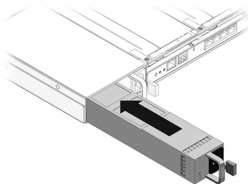
FIGURE 6-18 Installation d'une alimentation (serveur Sun SPARC Enterprise T5120)
