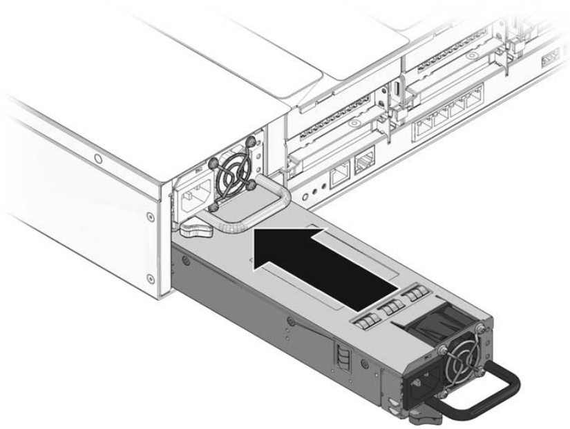
FIGURE 6-22 Installation d'une alimentation (serveur Sun SPARC Enterprise T5220)
