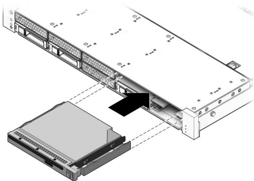
FIGURE 6-2 Installation du module DVD/USB (serveur Sun SPARC Enterprise T5120)
