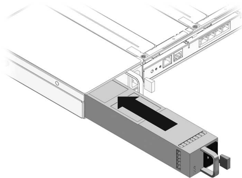
FIGURE 4-10 Installation d'une alimentation (Sun SPARC Enterprise T5120)
