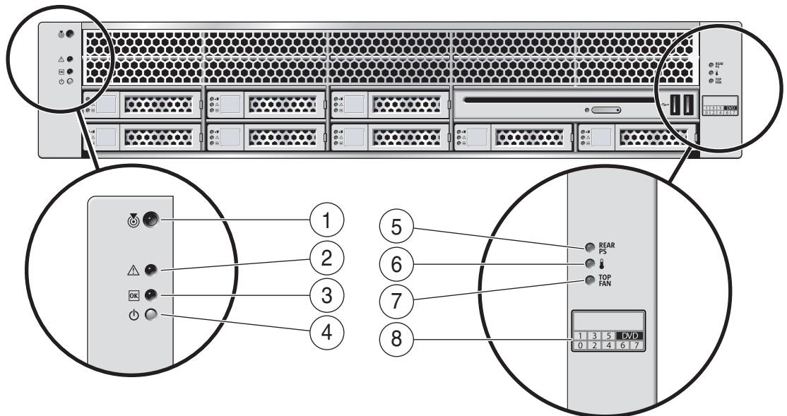
FIGURE 1-2 Accès aux composants situés à l'avant (serveur Sun SPARC Enterprise T5220)
