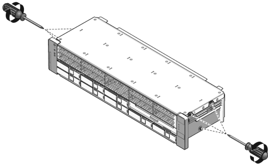
FIGURE 6-11 Retrait de l'assemblage de voyants lumineux du panneau de contrôle avant (serveur Sun SPARC Enterprise T5220)
