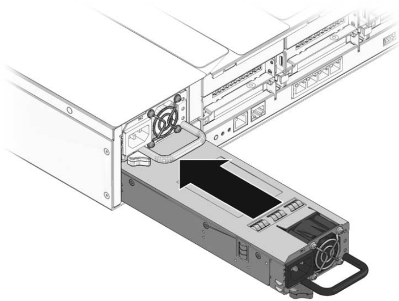
FIGURE 4-11 Installation d'une alimentation (Sun SPARC Enterprise T5220)
