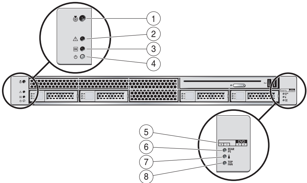
FIGURE 1-1 Accès aux composants situés à l'avant (serveur Sun SPARC Enterprise T5120)
