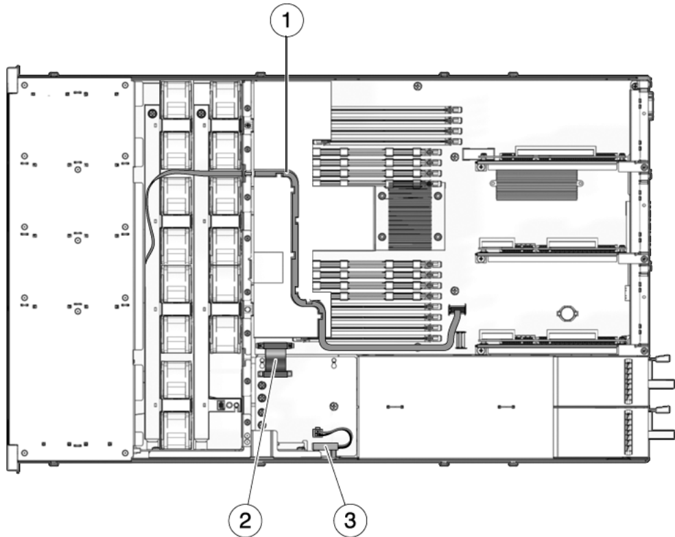
FIGURE A-4 Câbles (serveur Sun SPARC Enterprise T5120)
