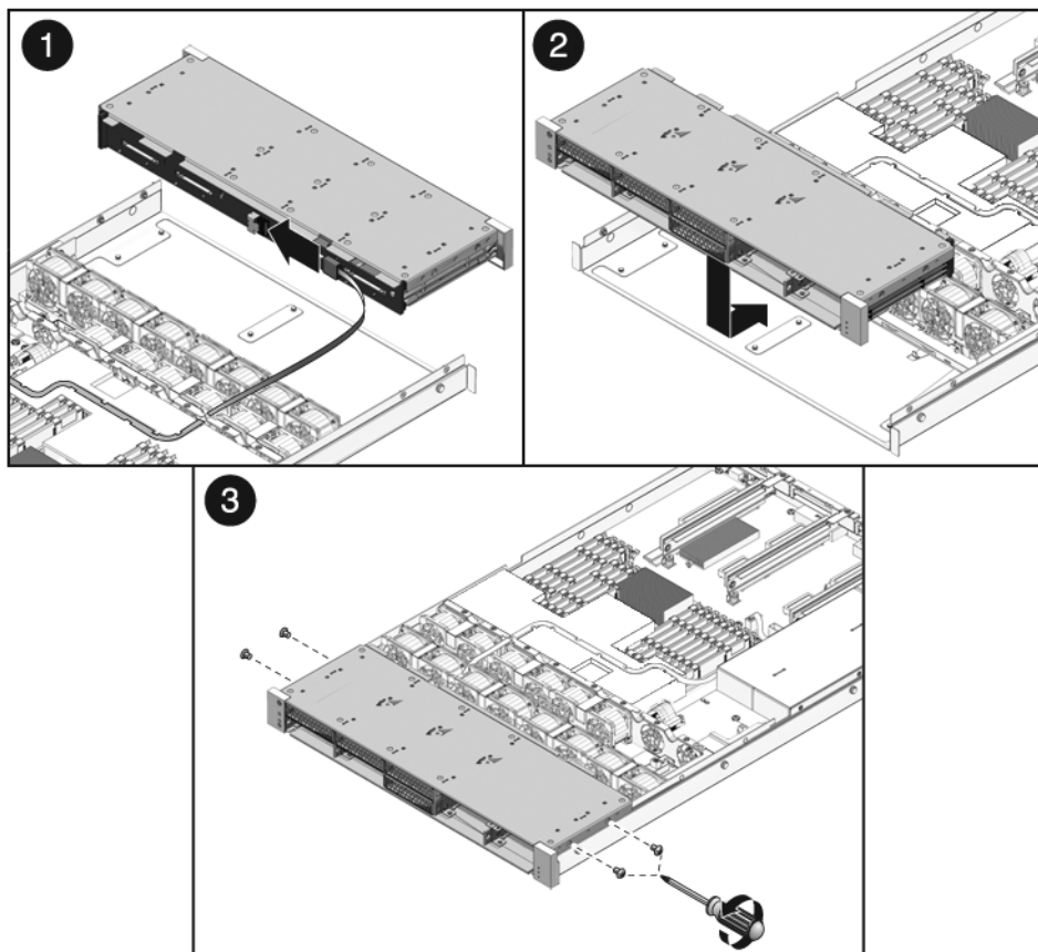
FIGURE 6-6 Installation du panier de disque dur (serveur Sun SPARC Enterprise T5120)
