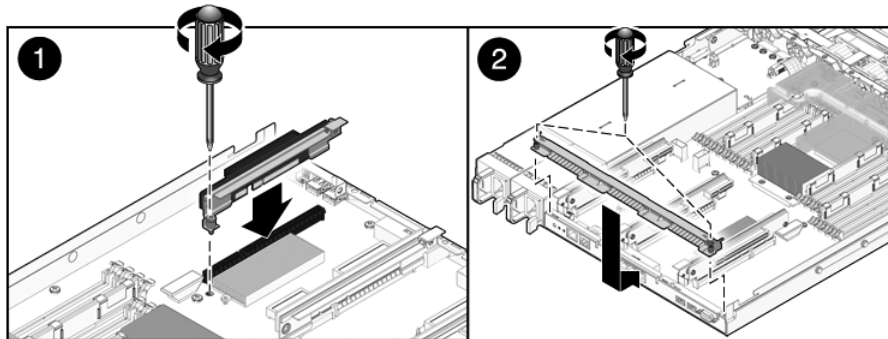
FIGURE 5-6 Installation d'une carte riser PCIe/XAUI (serveur Sun SPARC Enterprise T5120)
