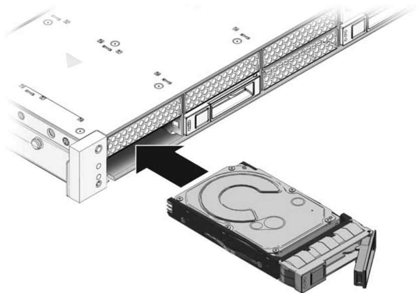
FIGURE 4-3 Installation d'un disque dur (serveur Sun SPARC Enterprise T5220)
