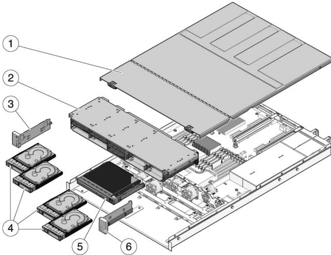
FIGURE A-1 Composants d'E/S (serveur Sun SPARC Enterprise T5120)
