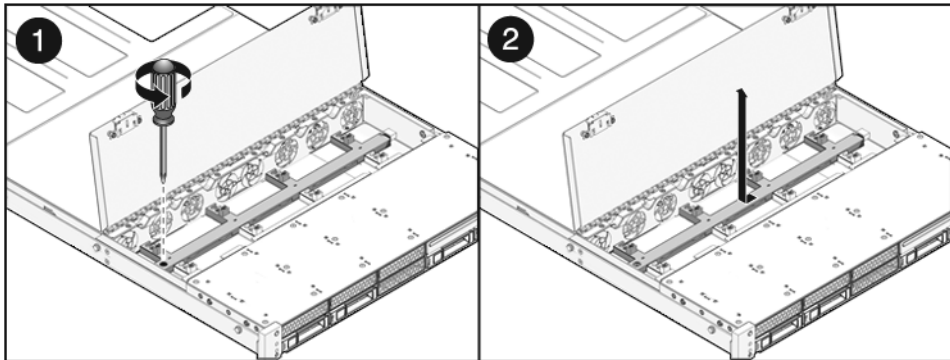
FIGURE 6-3 Retrait d’une carte d’alimentation de ventilateur (serveur Sun SPARC Enterprise T5120)
