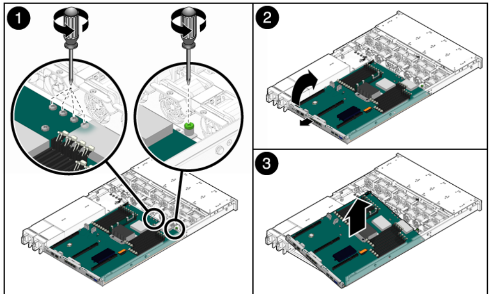
FIGURE 5-11 Retrait de l'assemblage de la carte mère (illustration du serveur Sun SPARC Enterprise T5120)
