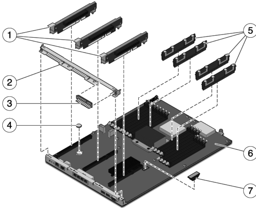
FIGURE A-2 Composants de la carte mère (serveur Sun SPARC Enterprise T5120)
