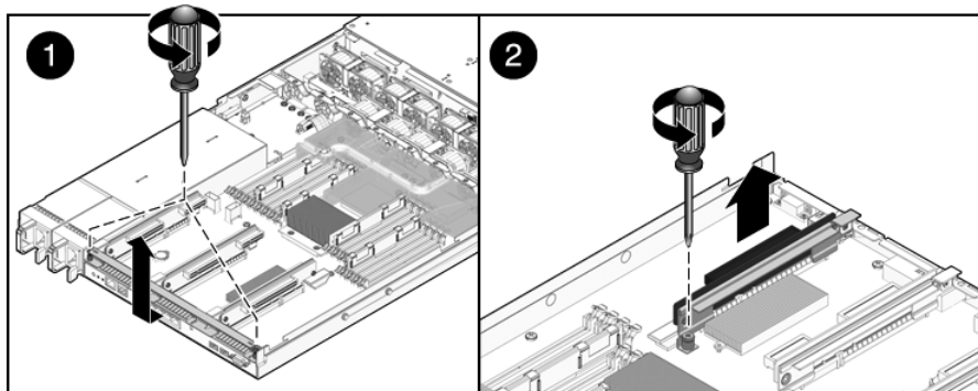
FIGURE 5-4 Retrait d'une carte riser PCIe/XAUI (serveur Sun SPARC Enterprise T5120)
