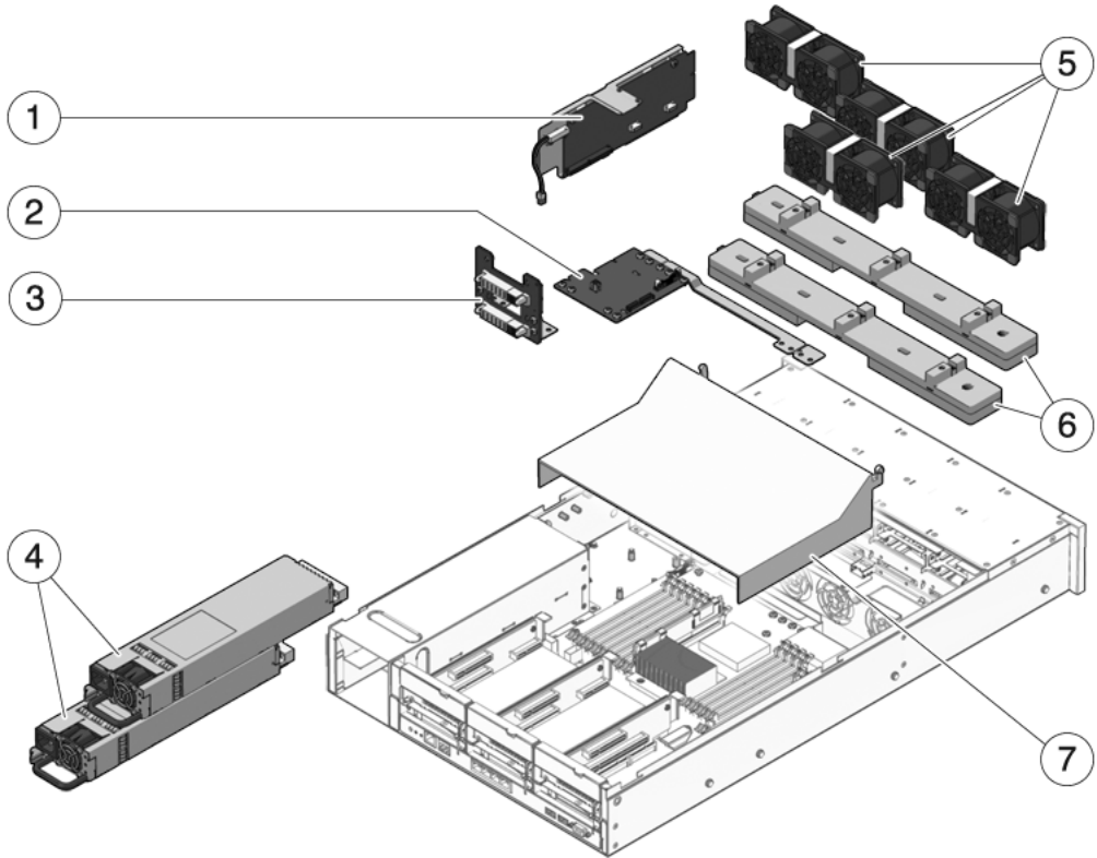
FIGURE A-11 Composants de distribution de puissance/module de ventilateur (serveur Sun SPARC Enterprise T5220)
