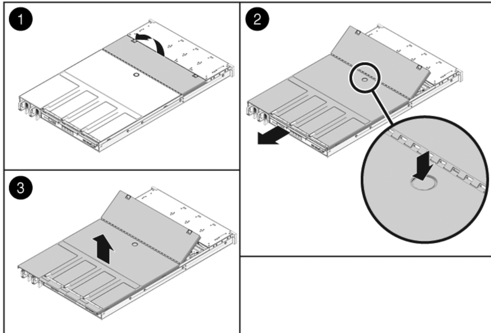
FIGURE 3-4 Retrait du capot supérieur (serveur Sun SPARC Enterprise T5120)
