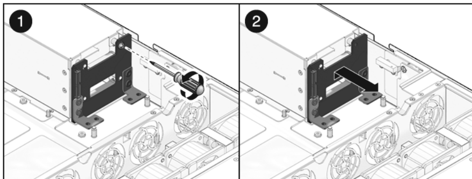
FIGURE 6-20 Retrait du backplane de l'alimentation (serveur Sun SPARC Enterprise T5220)
