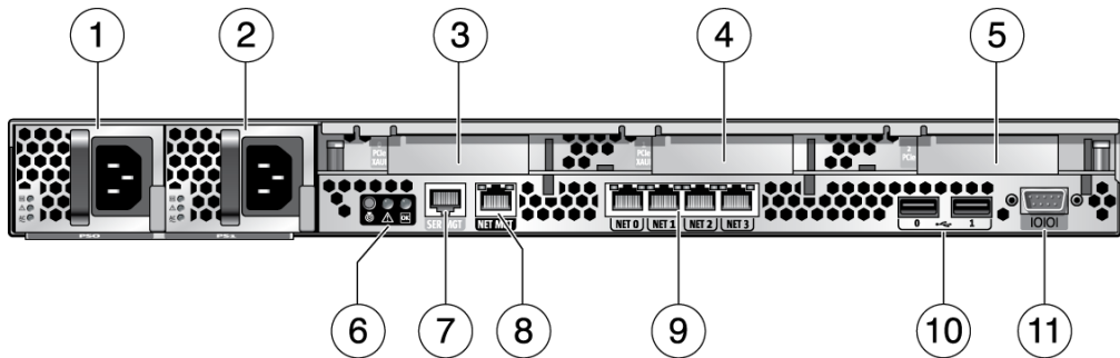
FIGURE 1-3 Accès arrière aux composants (serveur Sun SPARC Enterprise T5120)
