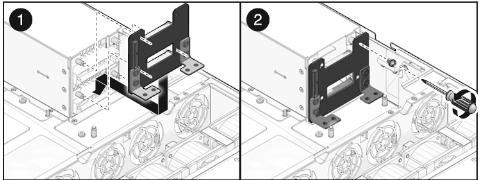
FIGURE 6-21 Installation du backplane de l'alimentation (serveur Sun SPARC Enterprise T5220)
