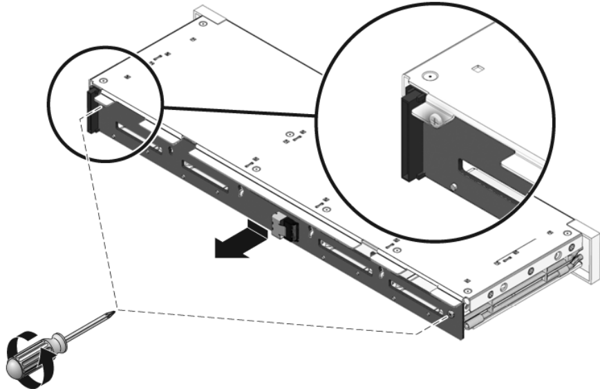
FIGURE 6-7 Retrait du backplane de disques durs (serveur Sun SPARC Enterprise T5120)
