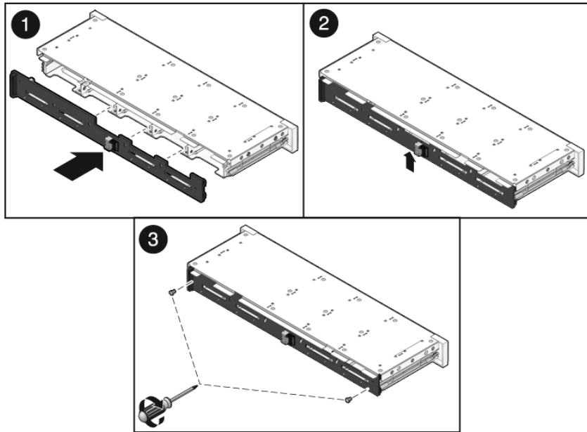
FIGURE 6-9 Installation du backplane d'unités de disque dur (serveur Sun SPARC Enterprise T5120)
