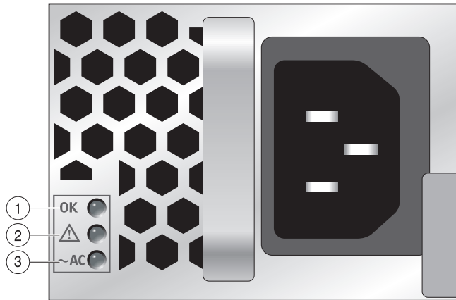
FIGURE 4-6 DEL d'état des alimentations (illustration d'un Sun SPARC Enterprise T5120)
