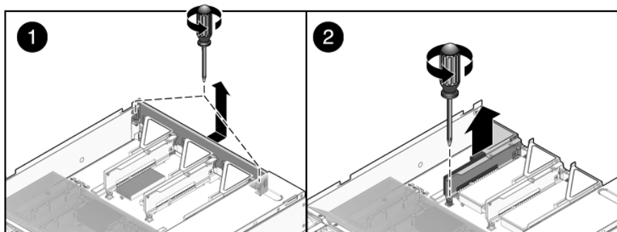
FIGURE 5-5 Retrait d'une carte Riser PCIe/XAUI (serveur Sun SPARC Enterprise T5220)
