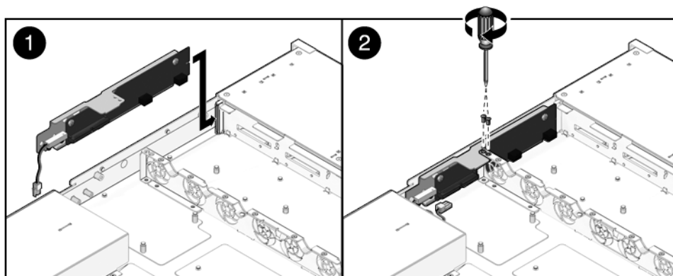
FIGURE 6-24 Installation de la carte d'accès (serveur Sun SPARC Enterprise T5120)
