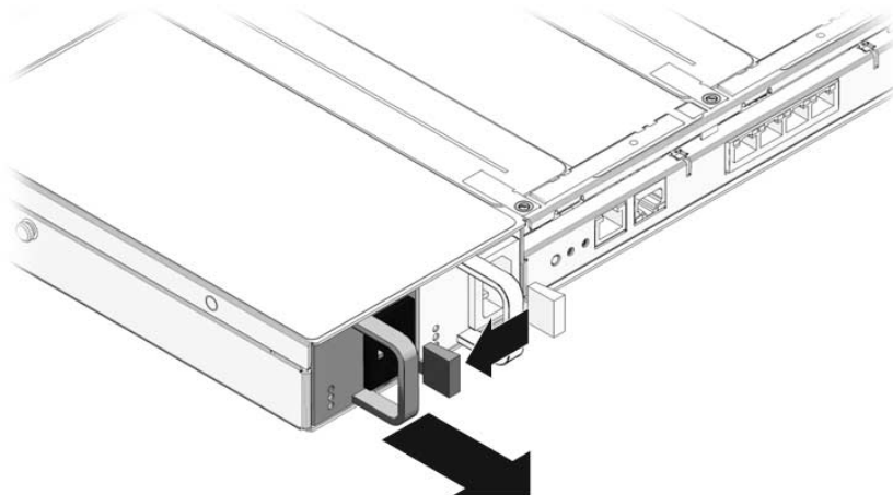
FIGURE 4-9 Poignée de dégagement d'unité d'alimentation (Sun SPARC Enterprise T5220)
