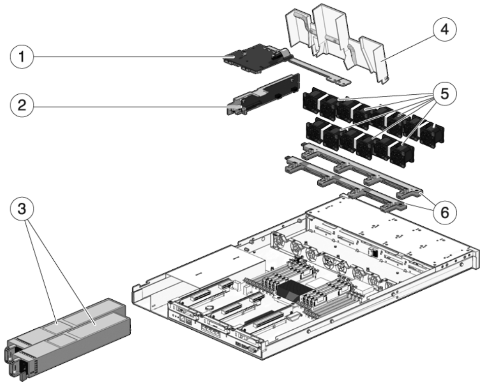
FIGURE A-3 Composants de distribution de puissance/module de ventilateur (serveur Sun SPARC Enterprise T5120)
