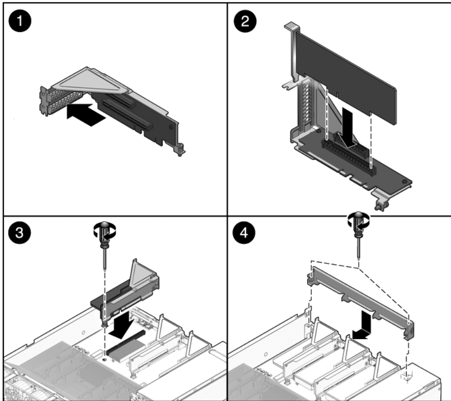
FIGURE 5-9 Installation d'une carte PCIe (Sun SPARC Enterprise T5220)
