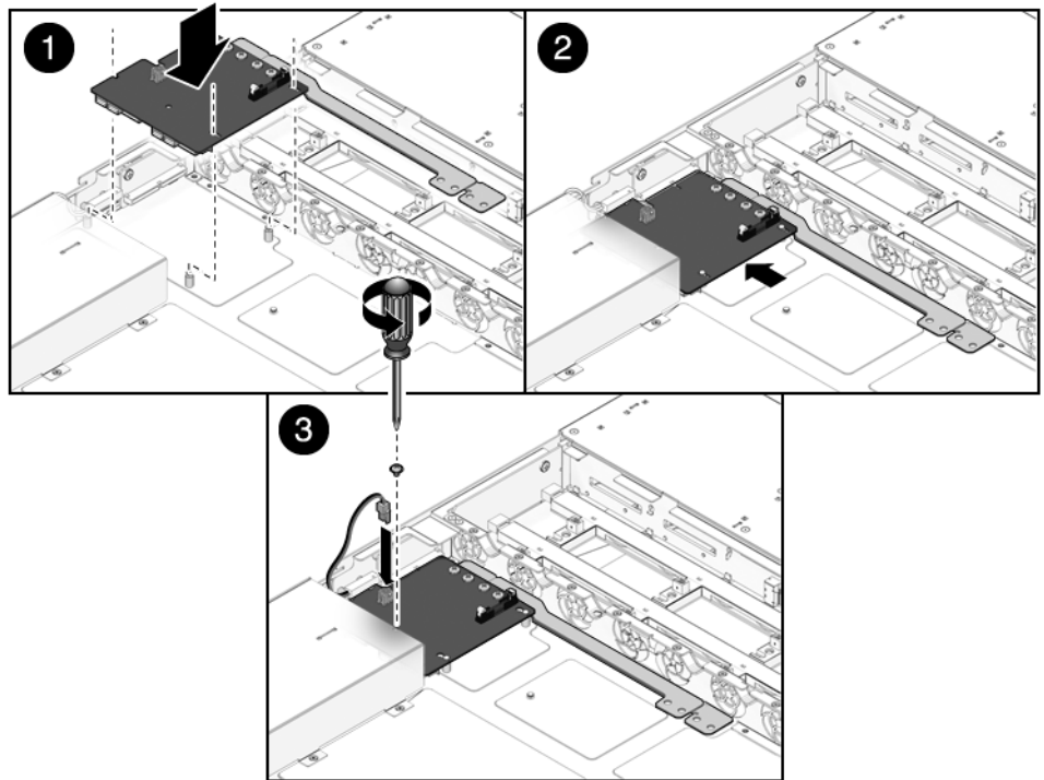
FIGURE 6-16 Installation de la carte de distribution de puissance (serveur Sun SPARC Enterprise T5120)
