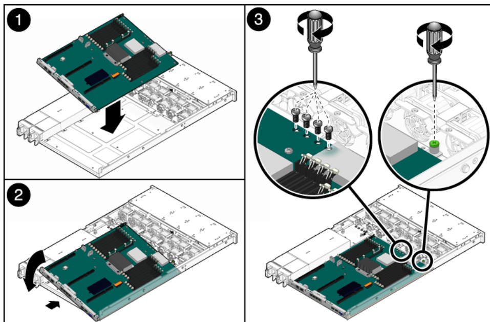
FIGURE 5-12 Installation de l'ensemble carte mère (serveur Sun SPARC Enterprise T5120)
