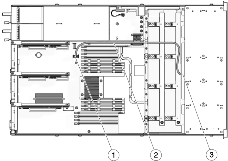
FIGURE A-5 (Serveur Sun SPARC Enterprise T5120, capacité de 4 unités de disque dur) Câbles HDD du contrôleur SAS intégré au backplane des unités de disque dur
