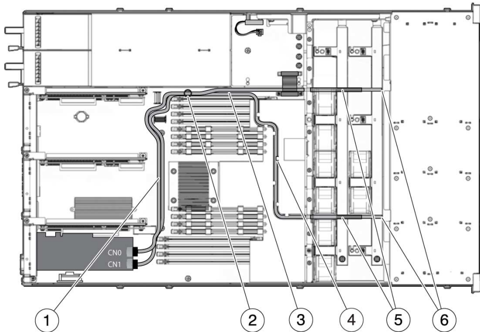
FIGURE A-8 Câbles HDD de la carte PCIe de HBA au backplane des unités de disque dur (Serveur Sun SPARC Enterprise T5120, capacité de 8 unités de disque dur)
