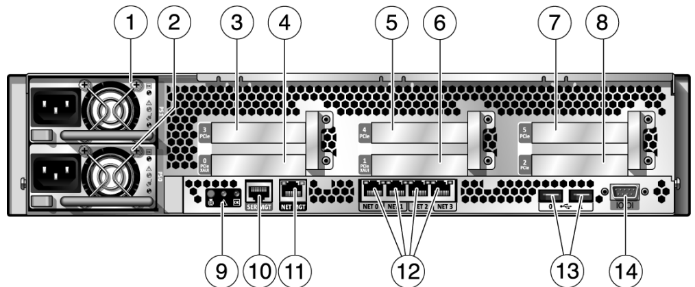
FIGURE 1-4 Accès arrière aux composants (serveur Sun SPARC Enterprise T5220)
