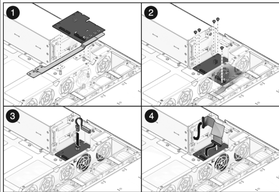
FIGURE 6-17 Installation de la carte de distribution de puissance (serveur Sun SPARC Enterprise T5220)
