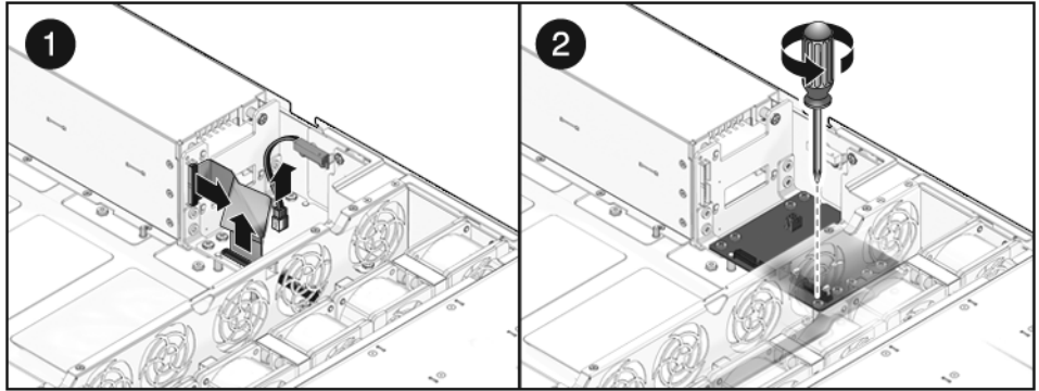
FIGURE 6-14 Retrait de la carte de distribution de puissance (serveur Sun SPARC Enterprise T5220)
