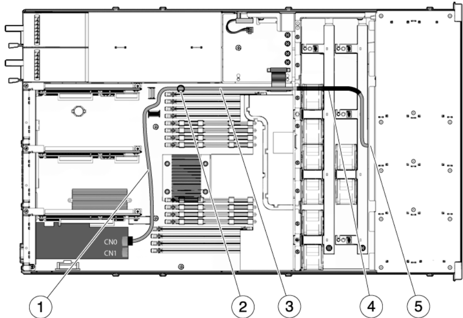
FIGURE A-7 Câbles HDD de la carte PCIe de HBA au backplane des unités de disque dur (Serveur Sun SPARC Enterprise T5120, capacité de 4 unités de disque dur)
