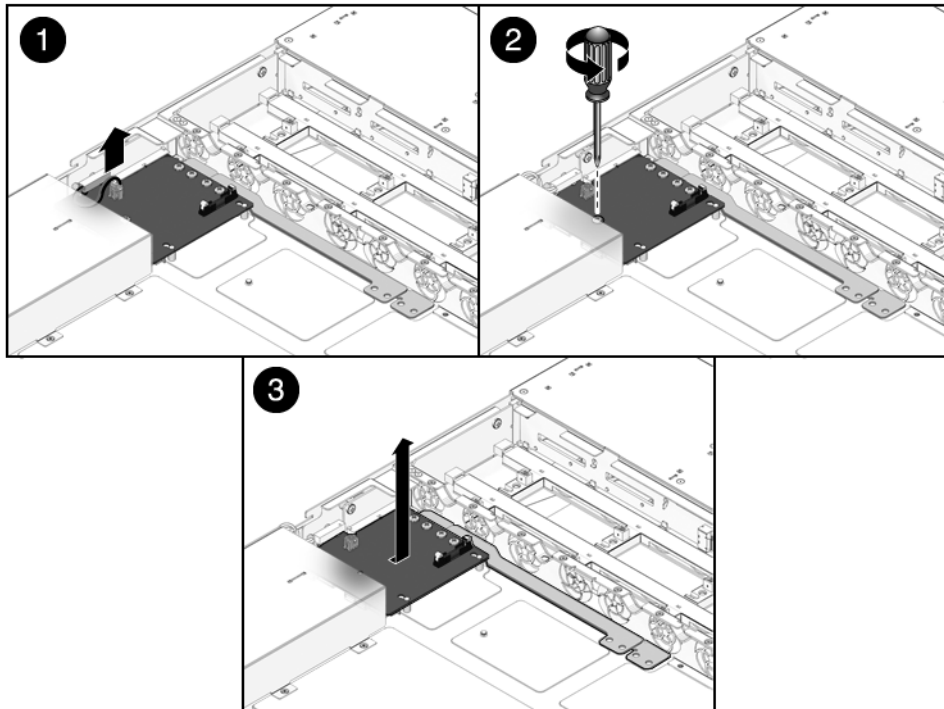
FIGURE 6-15 Retrait de la carte de distribution de puissance (serveur Sun SPARC Enterprise T5120)
