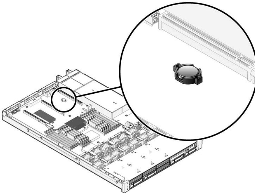
FIGURE 5-10 Emplacement de la batterie (serveur Sun SPARC Enterprise T5120)
