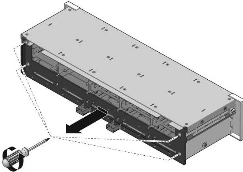
FIGURE 6-8 Retrait du backplane de disques durs (serveur Sun SPARC Enterprise T5220)
