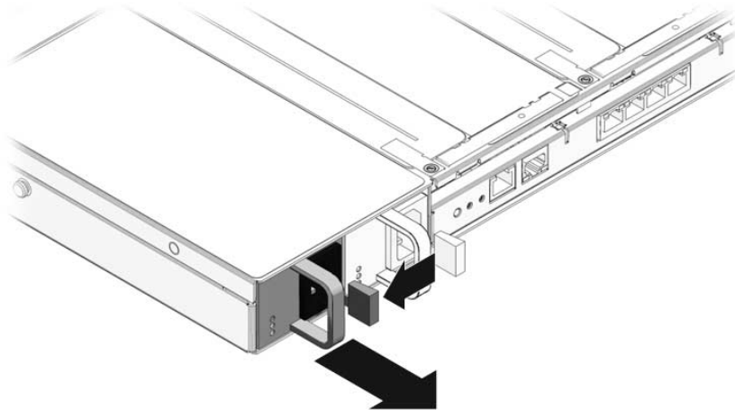
FIGURE 6-13 Retrait d'une unité d'alimentation (serveur Sun SPARC Enterprise T5120)
