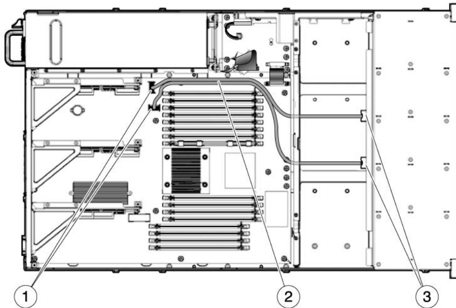
FIGURE A-13 Câbles HDD du contrôleur SAS intégré vers le backplane des unités de disque dur (Serveur Sun SPARC Enterprise T5220)
