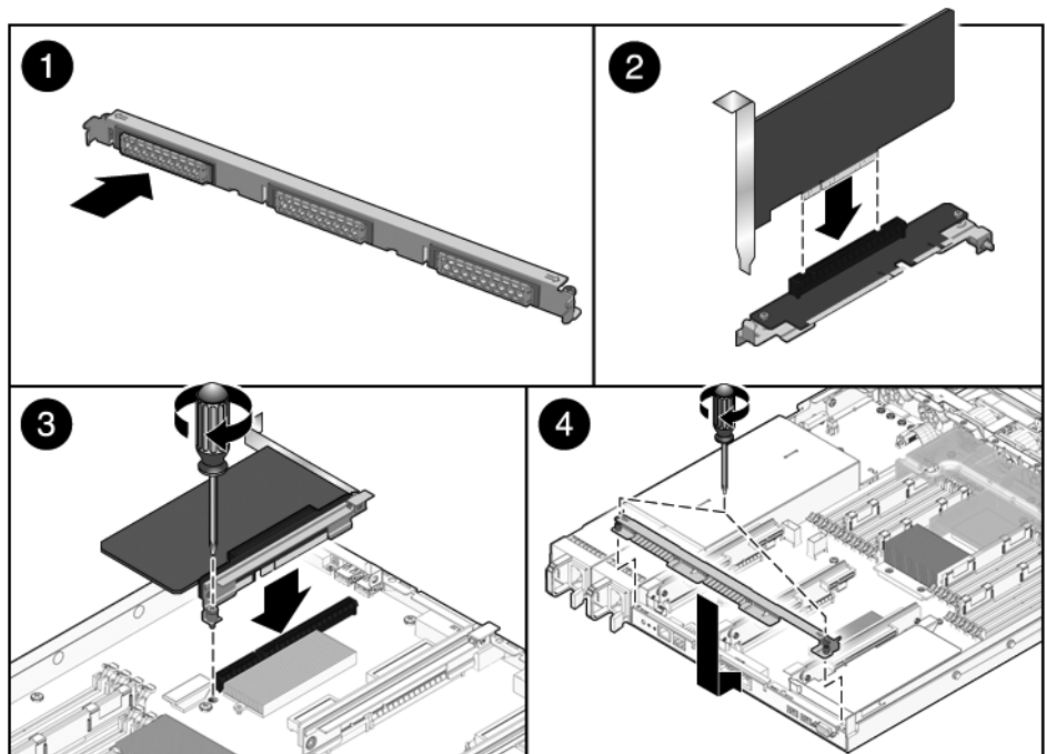
FIGURE 5-8 Installation d'une carte PCIe (Sun SPARC Enterprise T5120)
