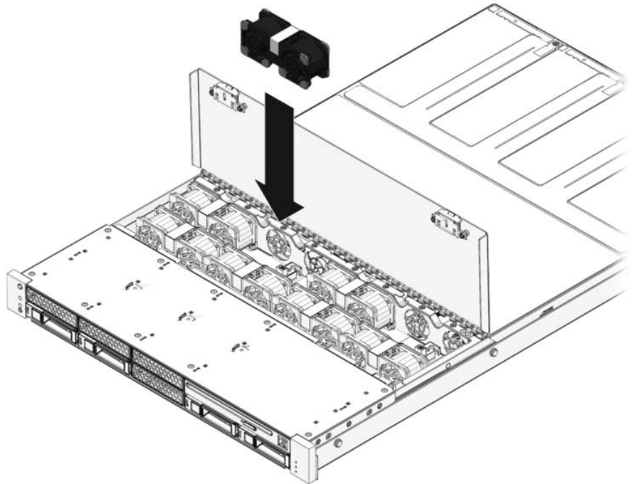
FIGURE 4-5 Installation d'un module de ventilateur
