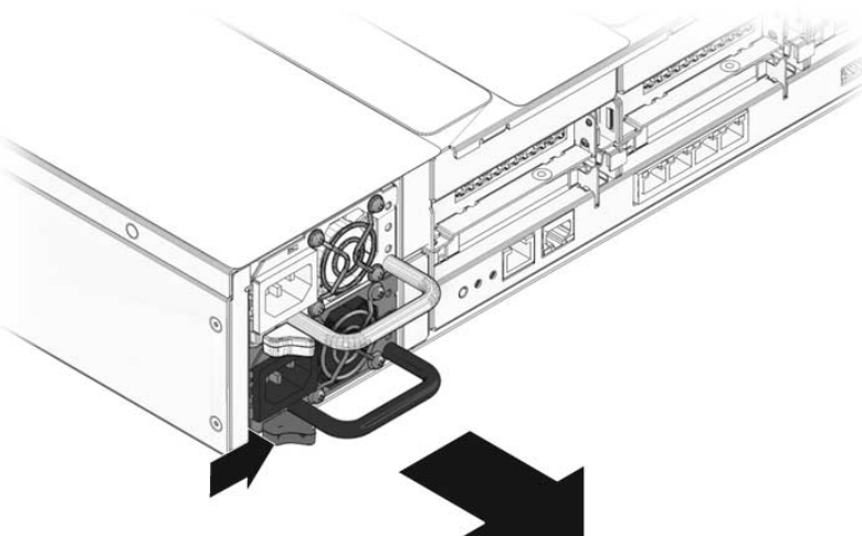
FIGURE 4-9 Poignée de dégagement d'unité d'alimentation (Sun SPARC Enterprise T5220)
