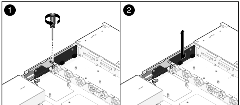
FIGURE 6-23 Retrait de la carte d'accès (serveur Sun SPARC Enterprise T5120)
