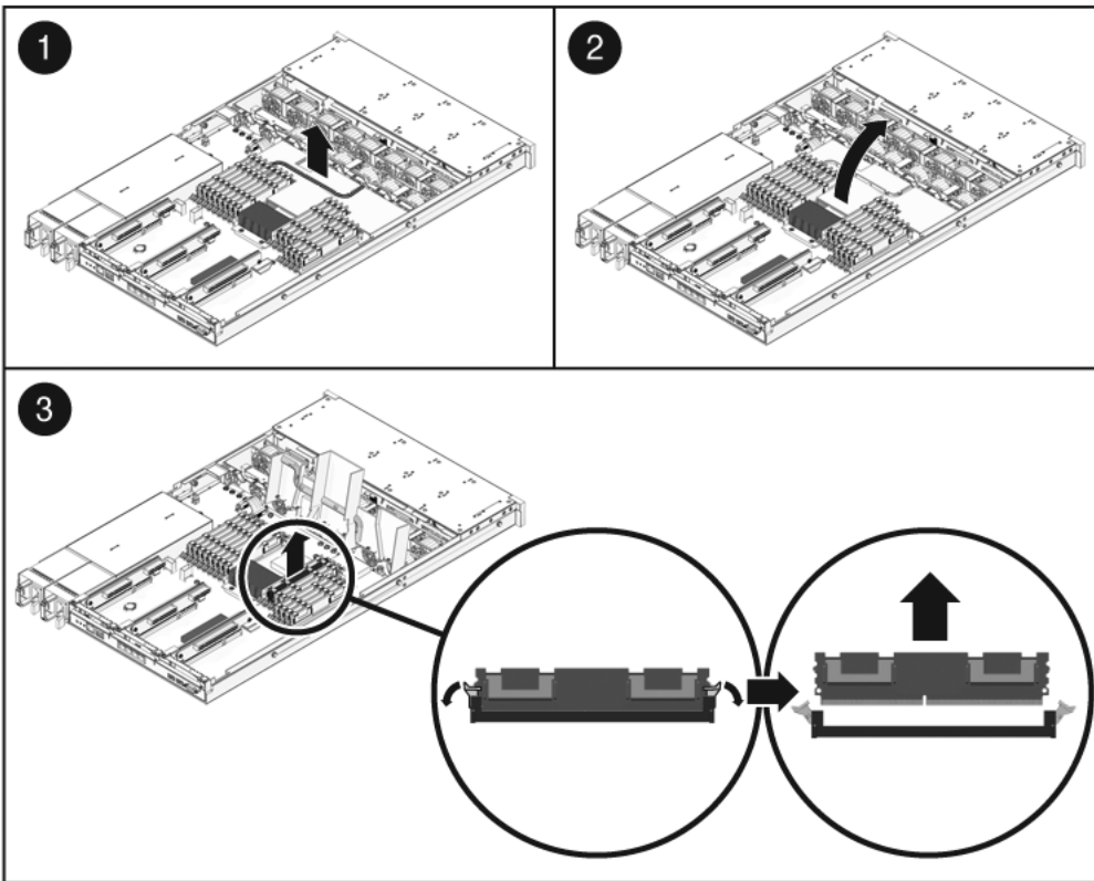
FIGURE 5-1 Retrait des modules de mémoire FB-DIMM
