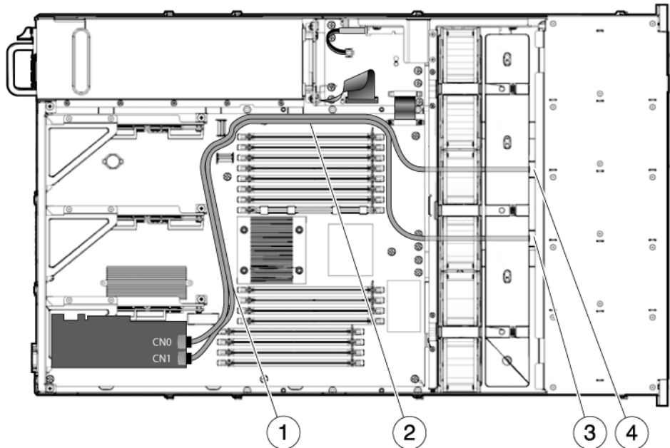
FIGURE A-14 Câbles HDD de la carte PCIe de HBA vers le backplane des unités de disque dur (Serveur Sun SPARC Enterprise T5220)
