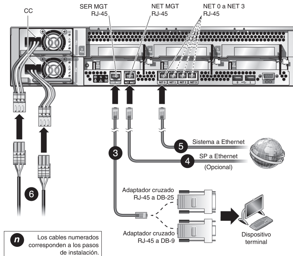
FIGURA 2 Conexiones del servidor
