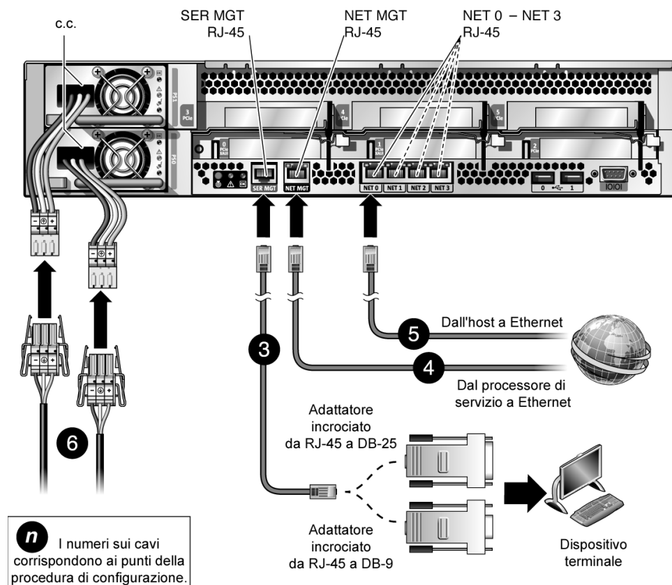
FIGURA 2 Connessioni del server
