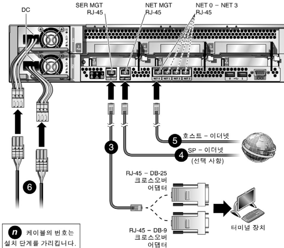
그림 2 서버 연결
