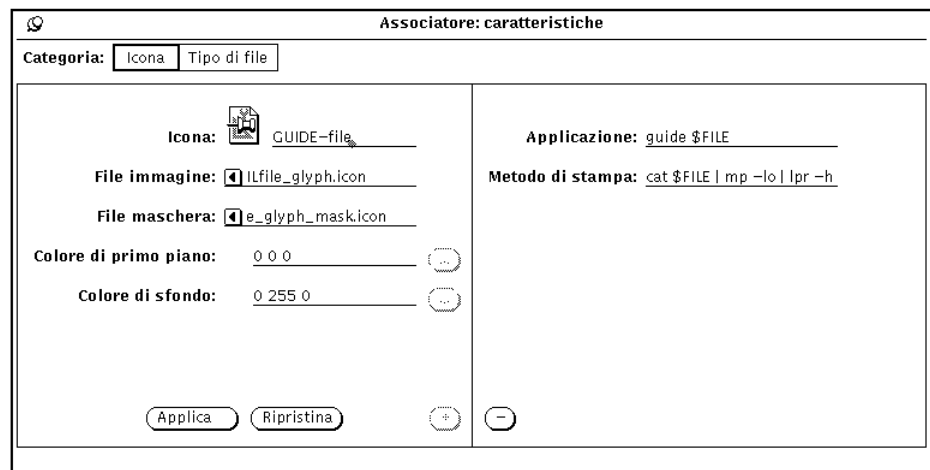
Figura 16-5 Finestra Caratteristiche Icona (completa)
