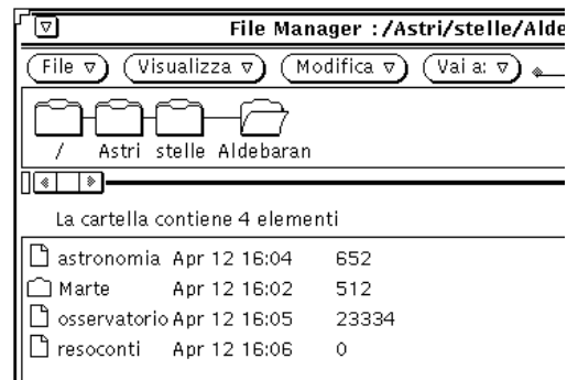
Figura 2-16 Esempio di visualizzazione in forma di lista
