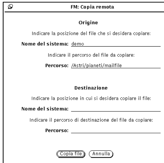
Figura 2-22 La finestra pop-up “Copia remota”
