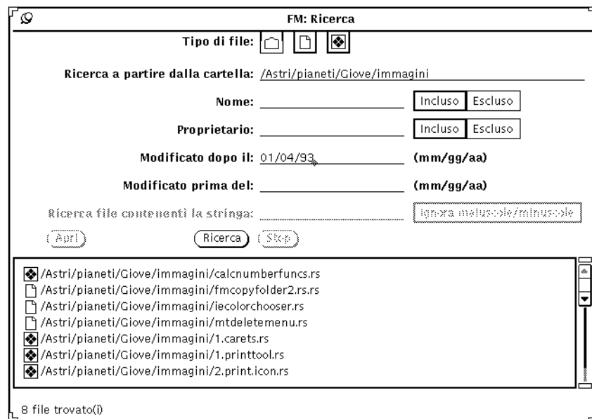
Figura 2-26 Risultati di una ricerca per data
