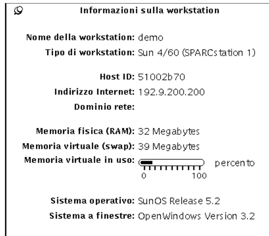
Figura 17-1 La finestra “Informazioni sulla workstation”
