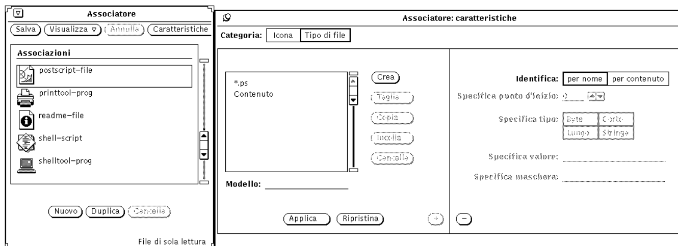
Figura 16-10 Tipo di file *.ps
