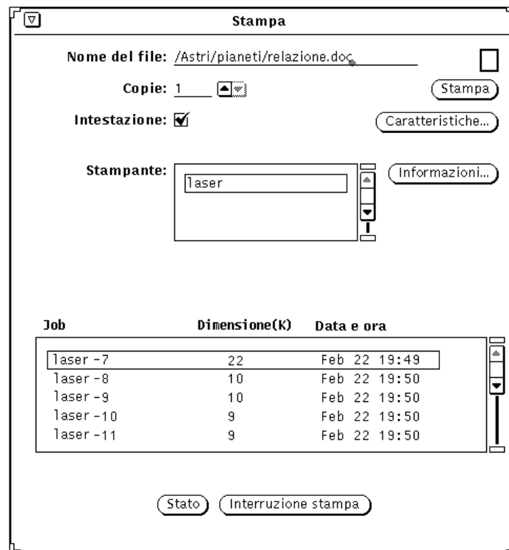
Figura 10-4 Esempio di file nella coda di stampa
