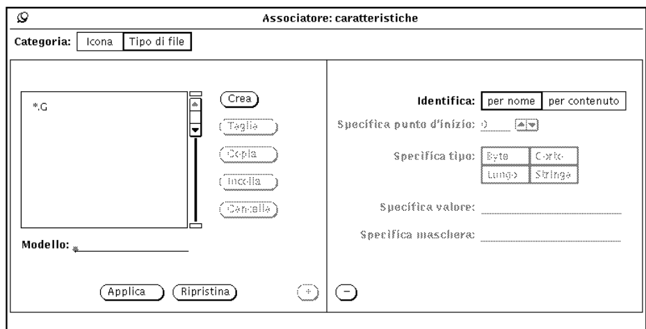
Figura 16-8 La finestra Caratteristiche Tipo di file (completa)
