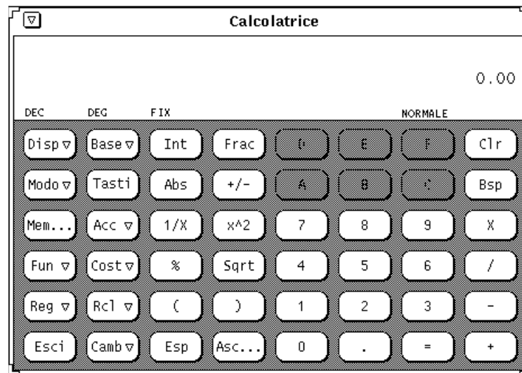
Figura 8-14 Disposizione dei tasti numerici a destra
