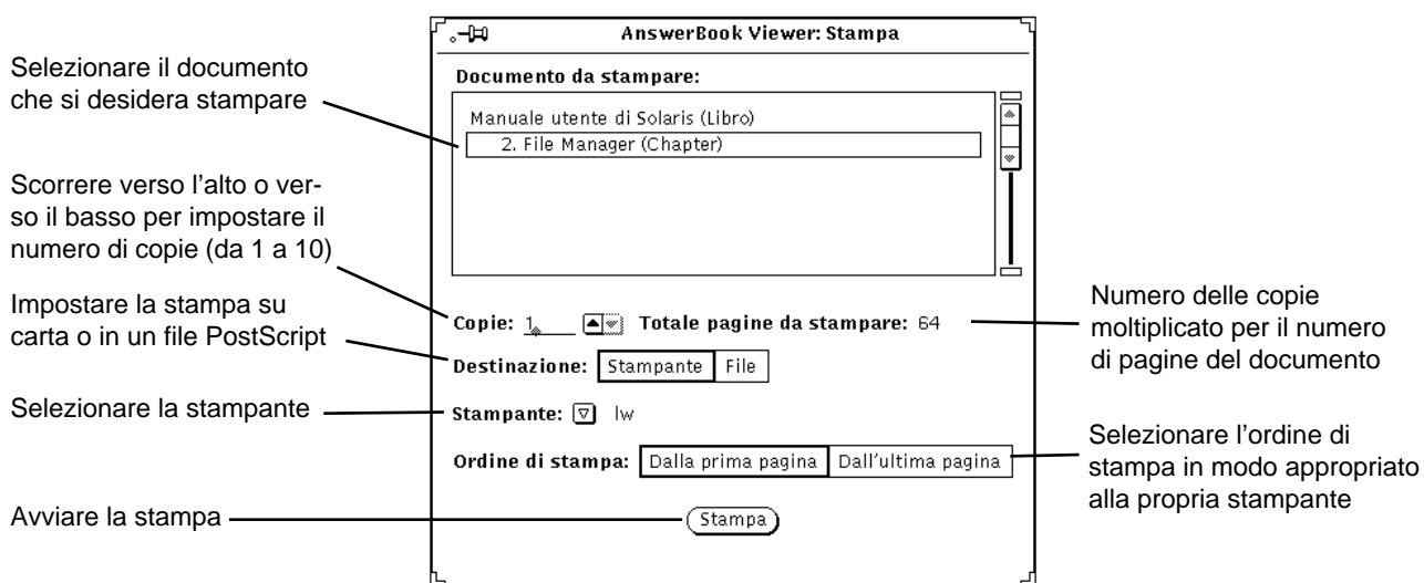
Figura 19-22 Finestra di stampa
