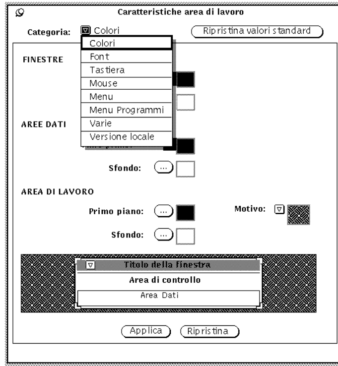
Figura 17-2 Il menu Categoria
