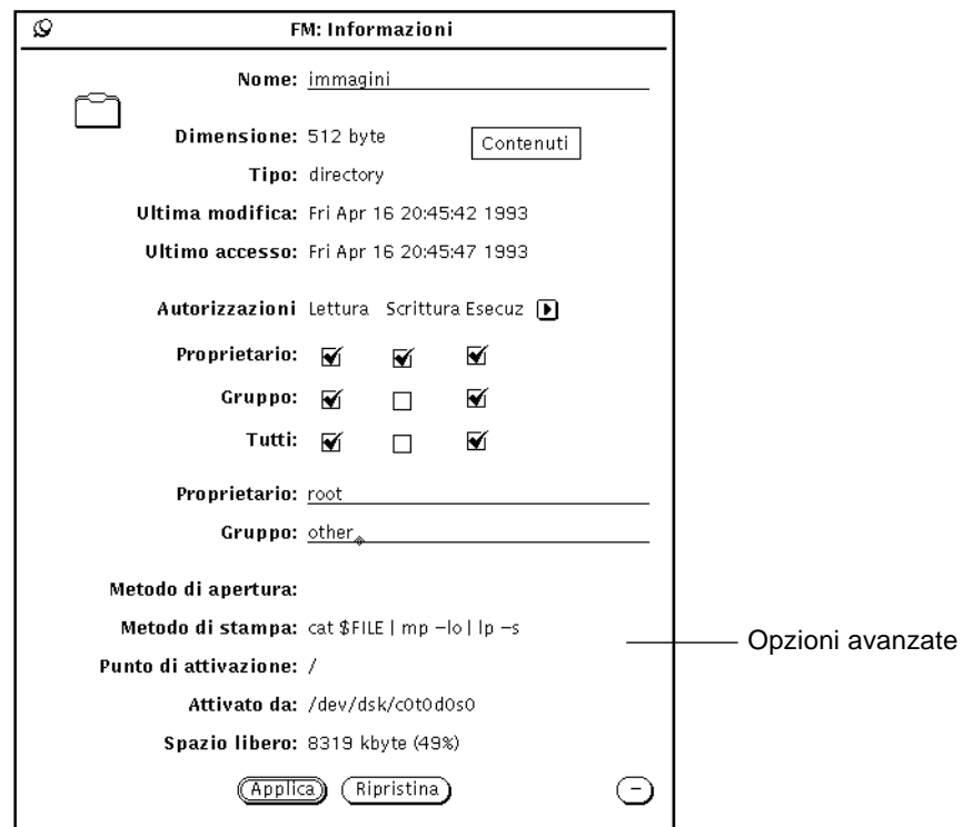
Figura 2-32 Esempio di finestra Informazioni
