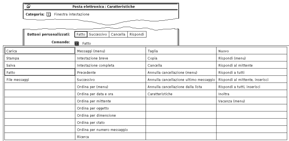
Figura 4-32 Il menu Comando nelle caratteristiche "Finestra intestazioni"
