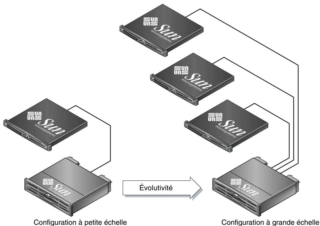
FIGURE 3 Architecture optimisée pour les serveurs d'applications
