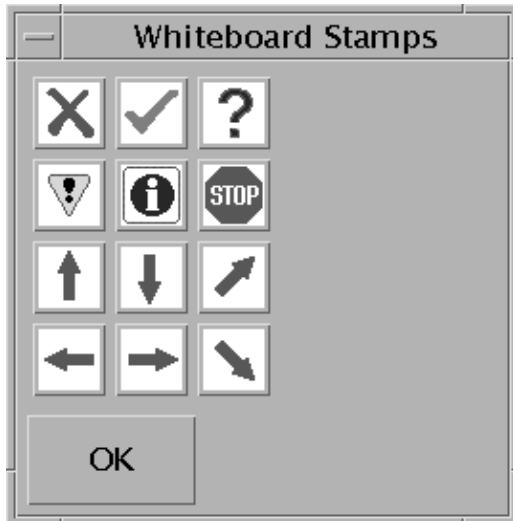
ABBILDUNG 2-9 Fenster "Whiteboard-Stempel"
