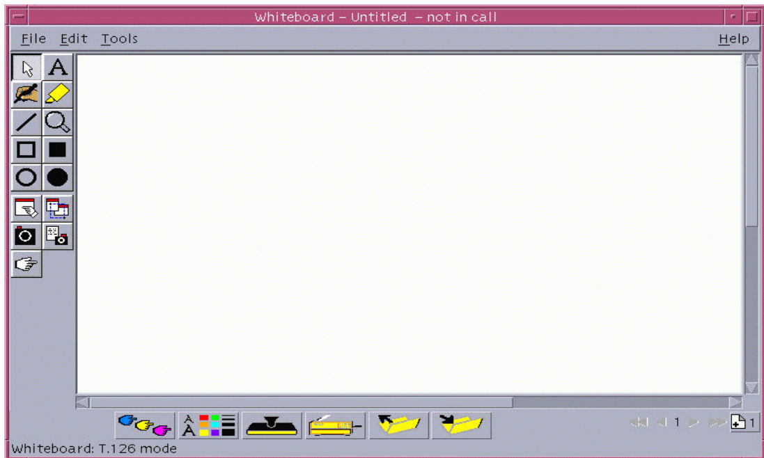
그림 2-4 SunForum 3.2 화이트보드
