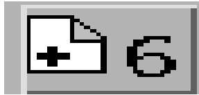
圖 2-10 「新頁面」按鈕
