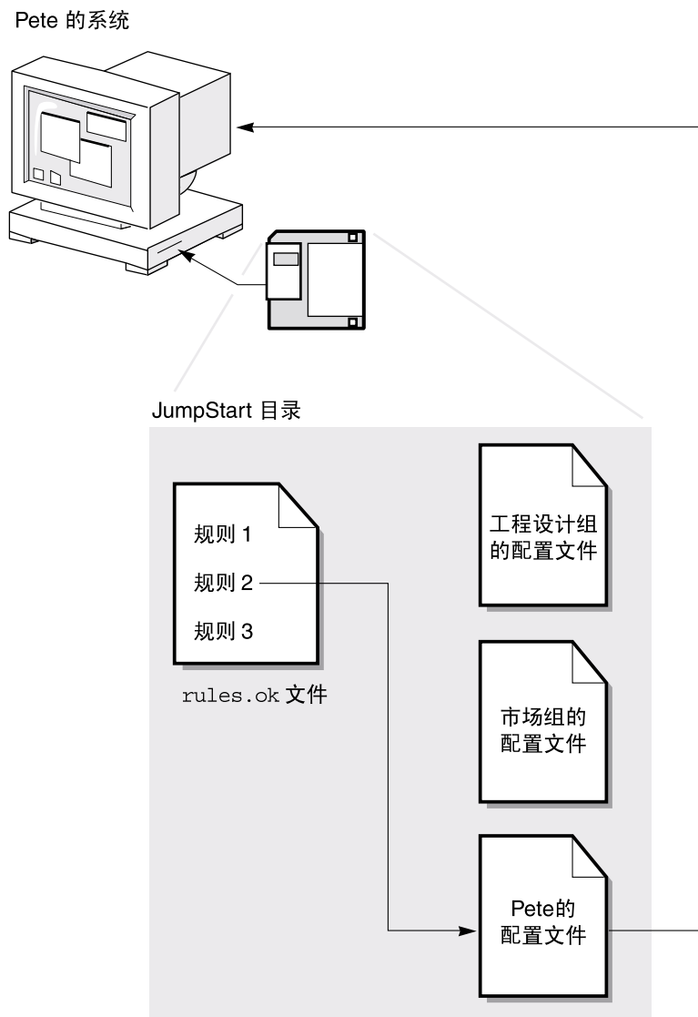
图形 22-1 定制 JumpStart 安装的工作原理：非联网示例
