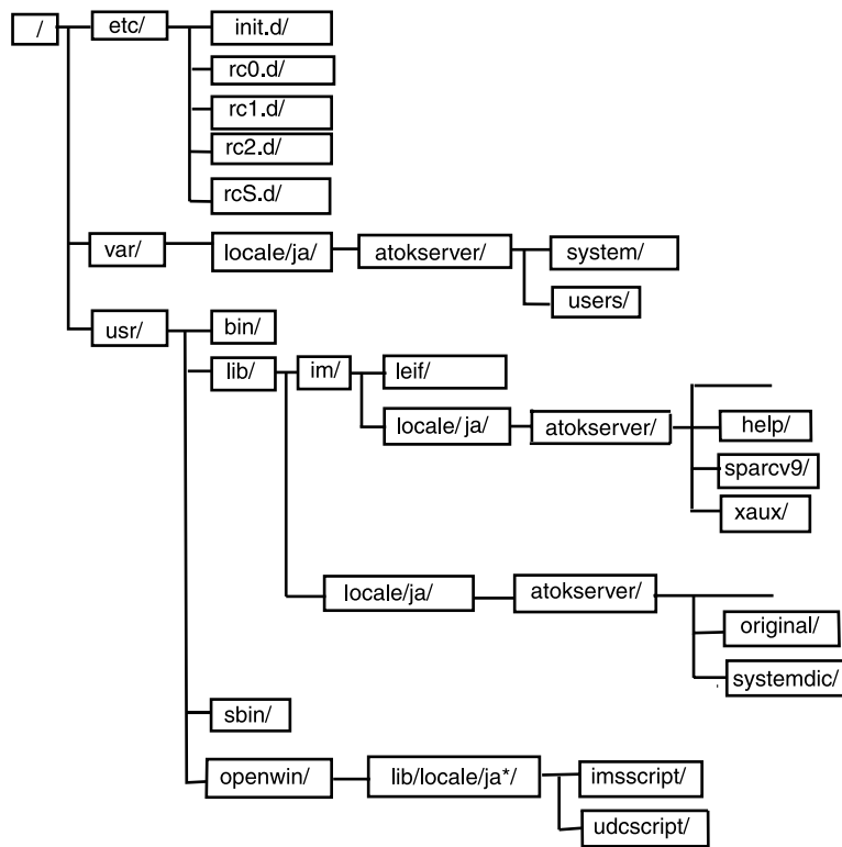
図 2-1 図 2-1 ATOK12 のディレクトリ構造
