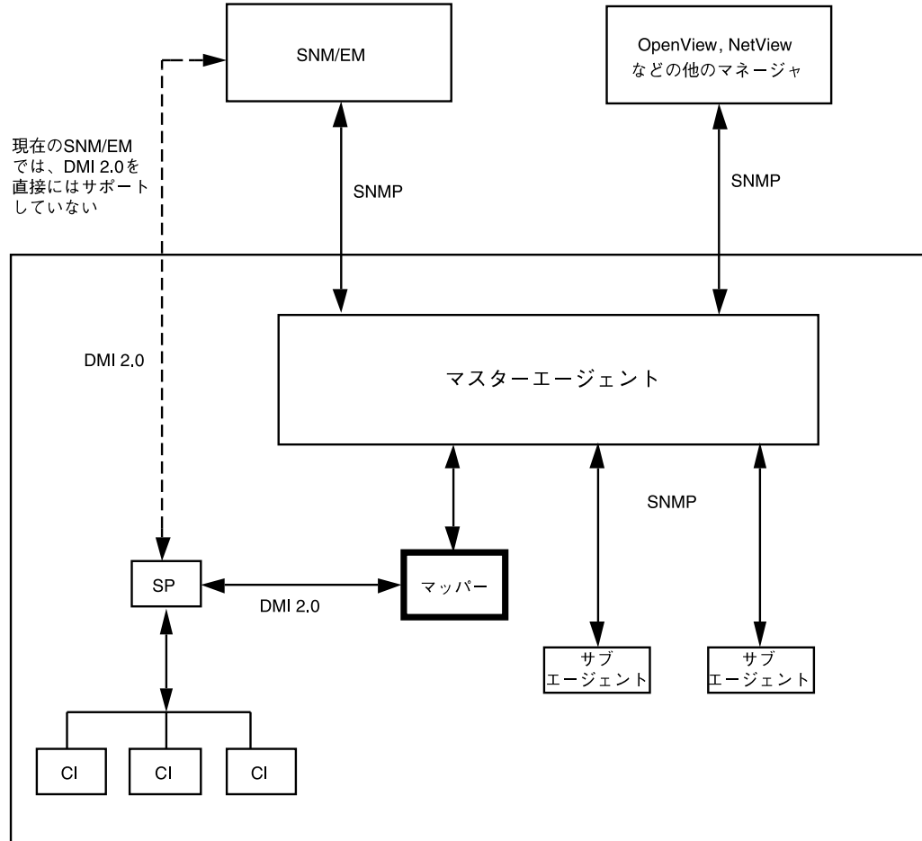
図 6-1 snmpXdmid の概要
