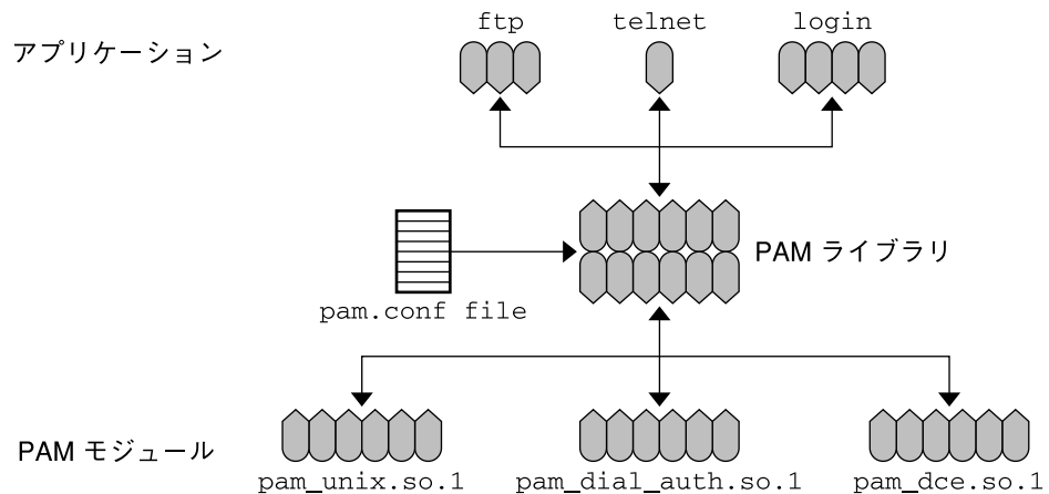
図 3-1 PAM の動作
