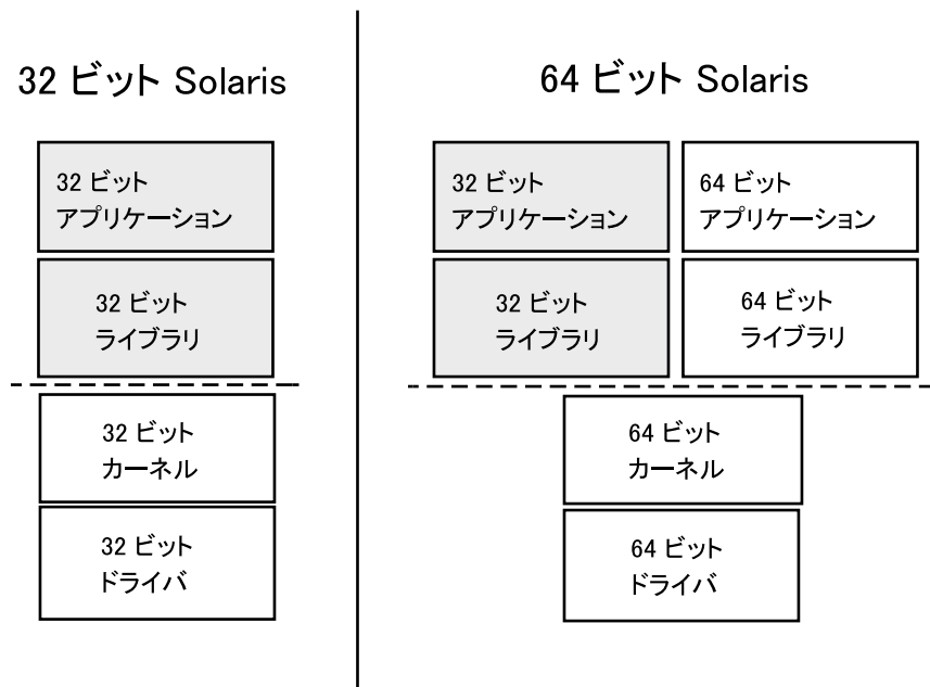
図 2-1 Solaris オペレーティング環境のアーキテクチャ
