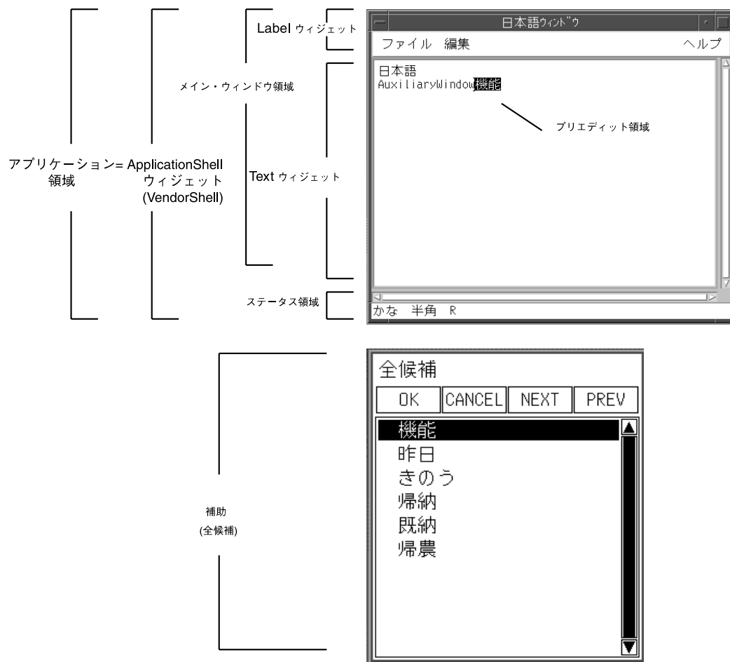
図 1-3 VendorShell ウィジェットと補助の例 (日本語)
