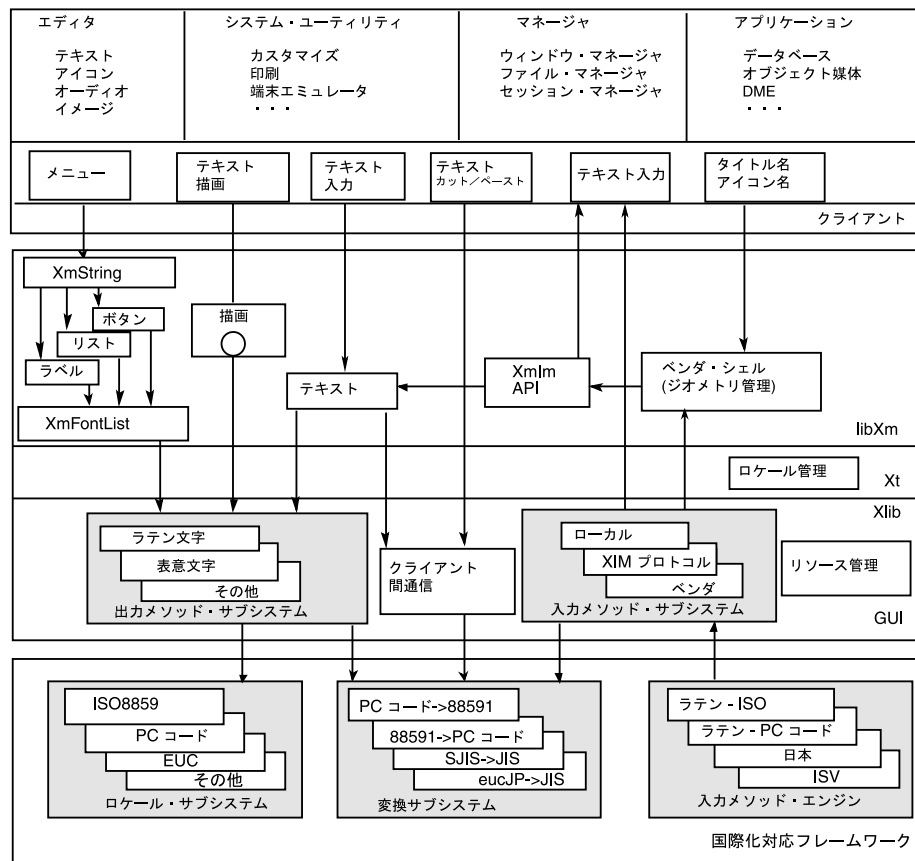
図 1-2 共通国際化対応システム
