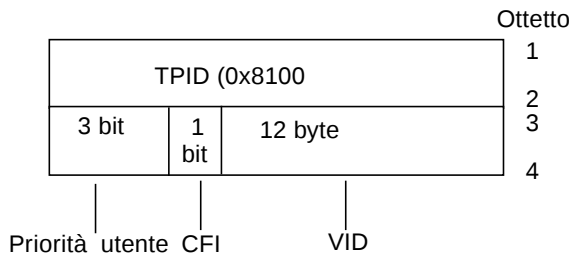
FIGURA 3-1 Formato Ethernet Tag Header
