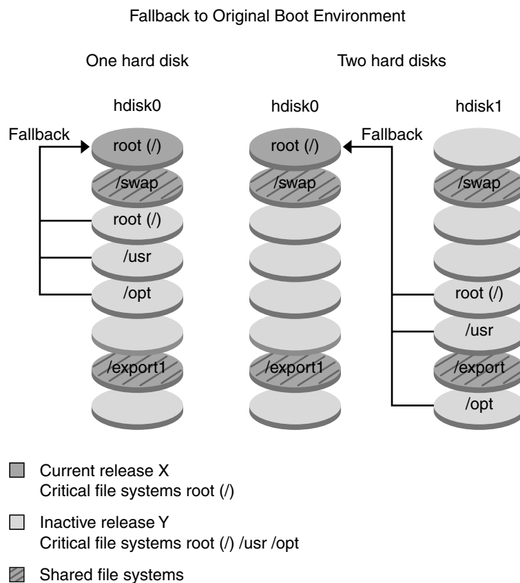
图形 30-7 回退到原始引导环境
