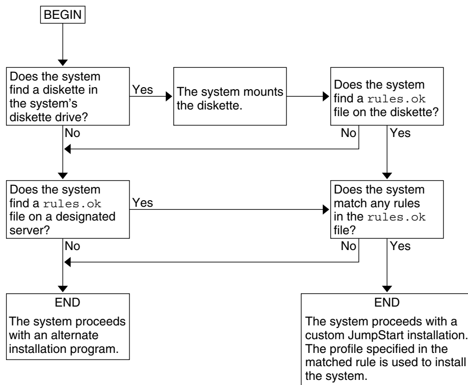
圖 22-3 自訂 JumpStart 安裝過程中會出現的情況
