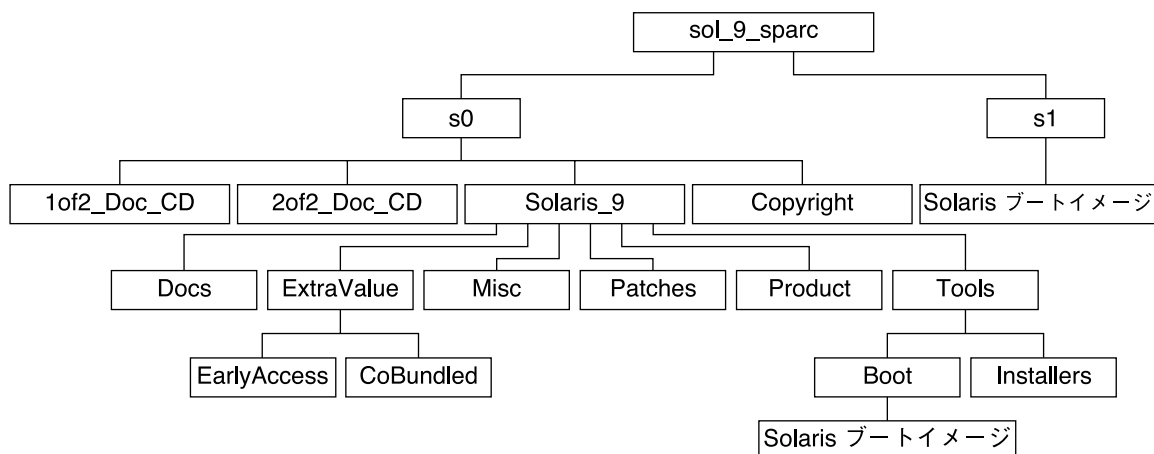
図 B-1 Solaris 9 DVD (SPARC 版)
