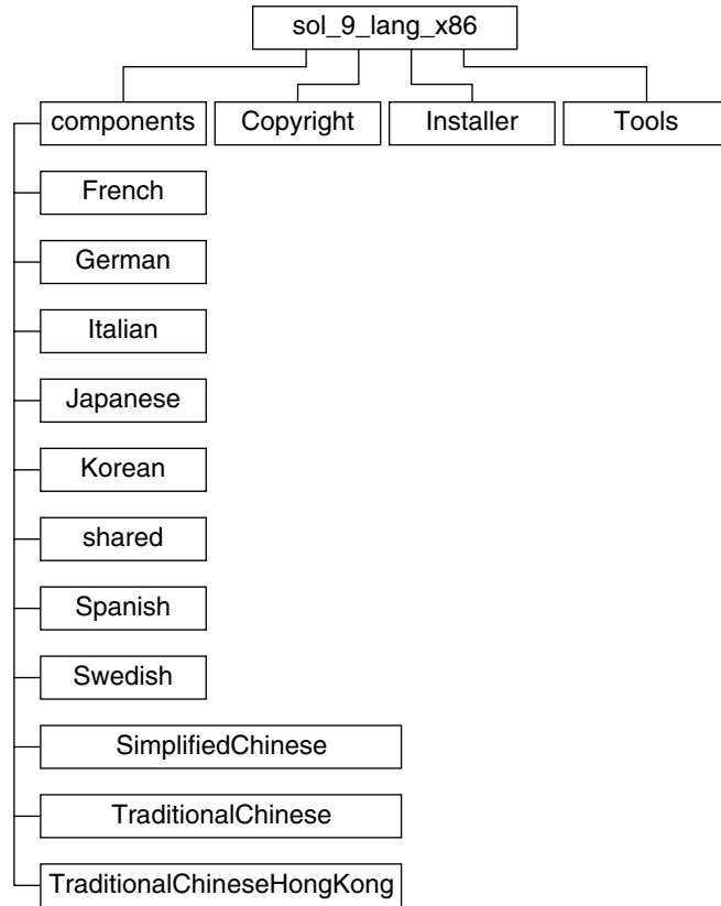
그림 B-10 Solaris 9 x86 Platform Edition Languages CD
