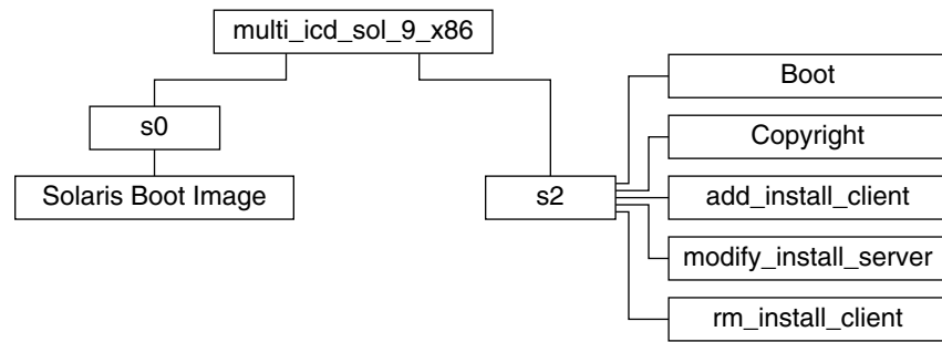
그림 B-7 x86: Solaris 9 x86 Platform Edition Installation CD
