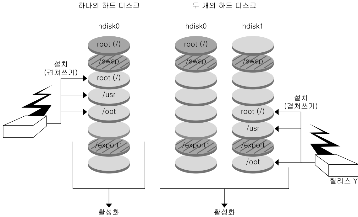
플래시 아카이브 설치
