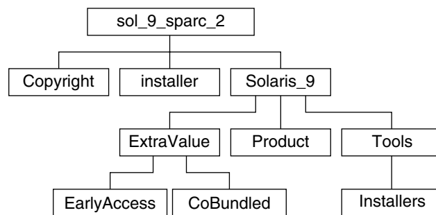
그림 B-4 SPARC: Solaris 9 Software 2 of 2 SPARC Platform Edition CD
