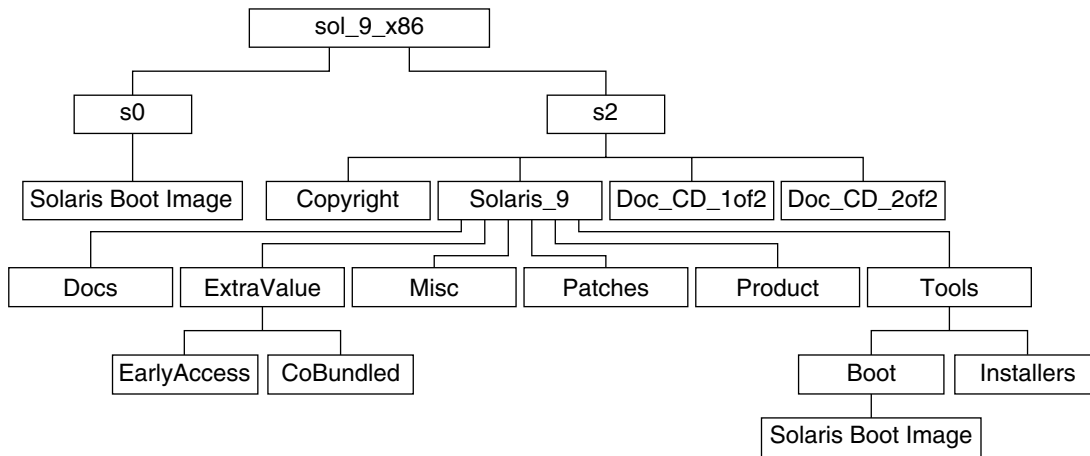
그림 B-6 Solaris 9 x86 Platform Edition DVD
