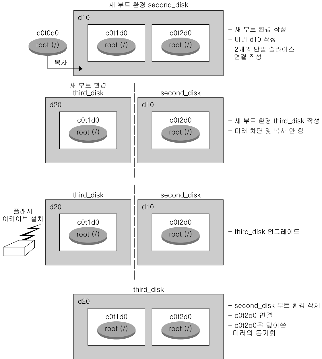
그림 35-2 RAID-1 볼륨(미러)의 한 쪽을 분리하고 업그레이드(계속)
