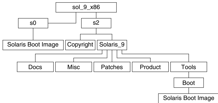
그림 B-8 x86: Solaris 9 Software 1 of 2 x86 Platform Edition CD
