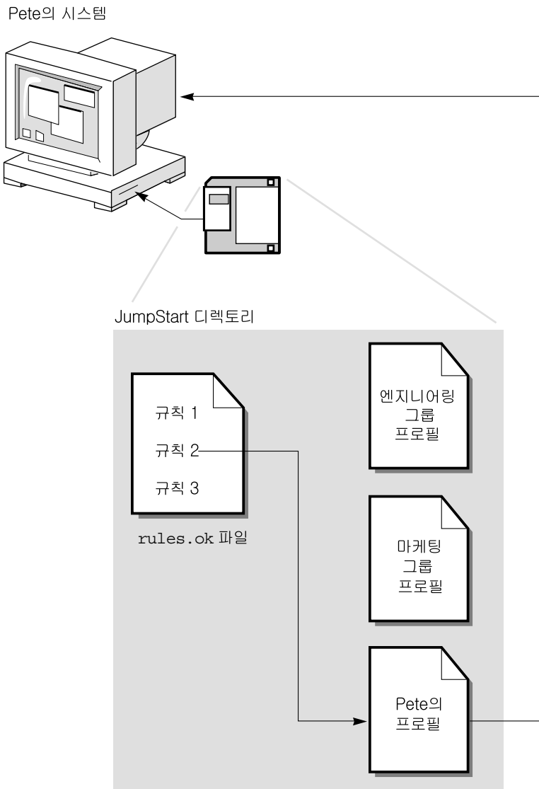
그림 22-1 사용자 정의 JumpStart 설치 작업: 네트워크에 연결되지 않은 예
