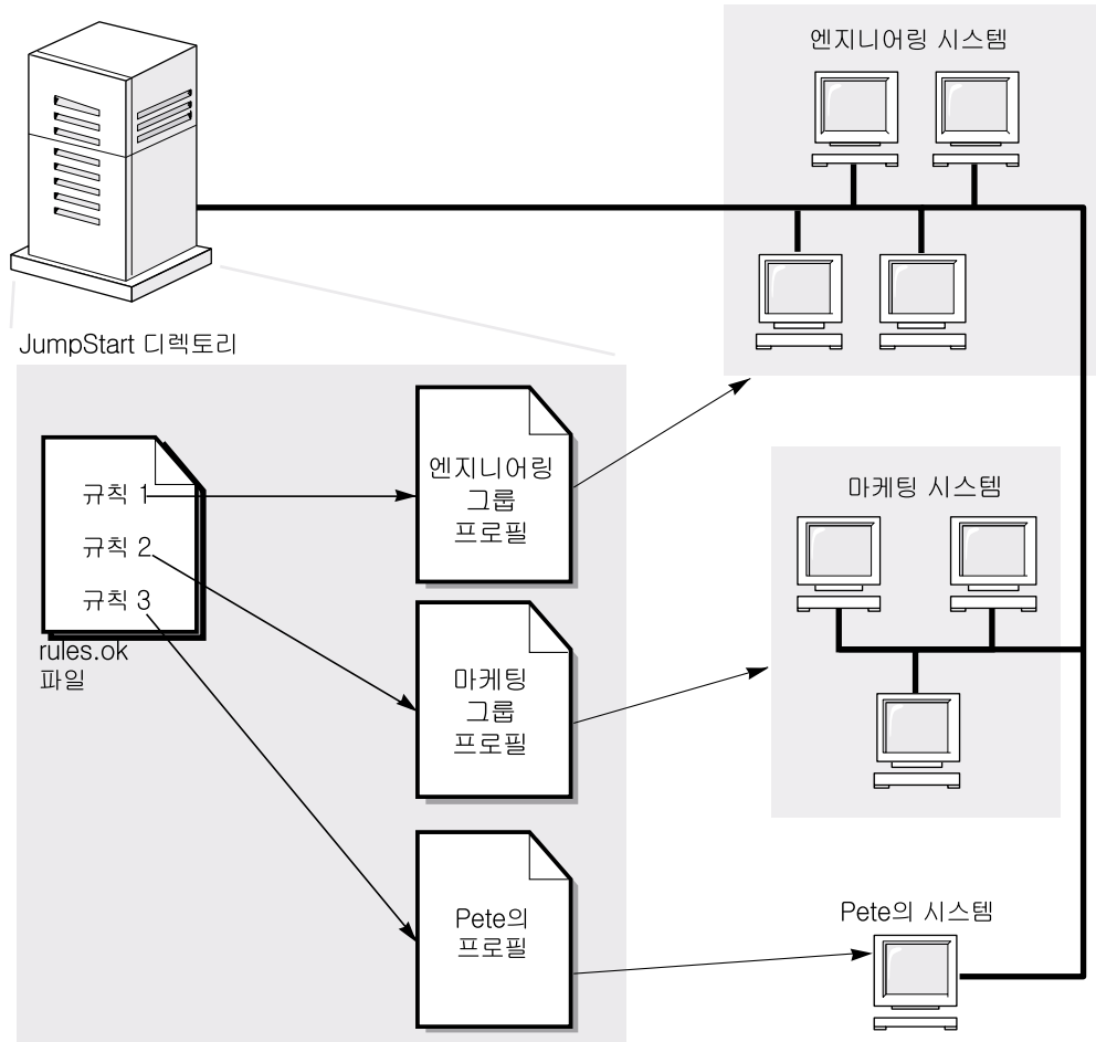
그림 22-2 사용자 정의 JumpStart 설치 작업: 네트워크에 연결된 예
