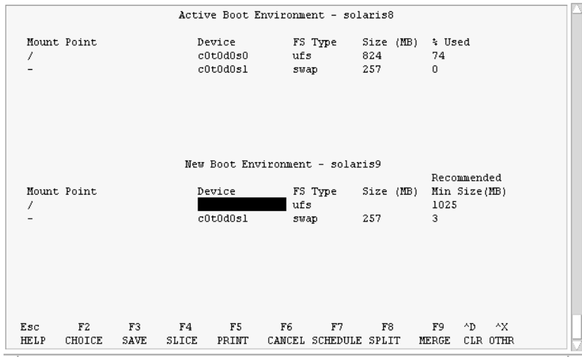
그림 35-4 Solaris Live Upgrade 구성 메뉴
