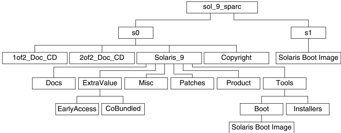
그림 B-1 Solaris 9 SPARC Platform Edition DVD
