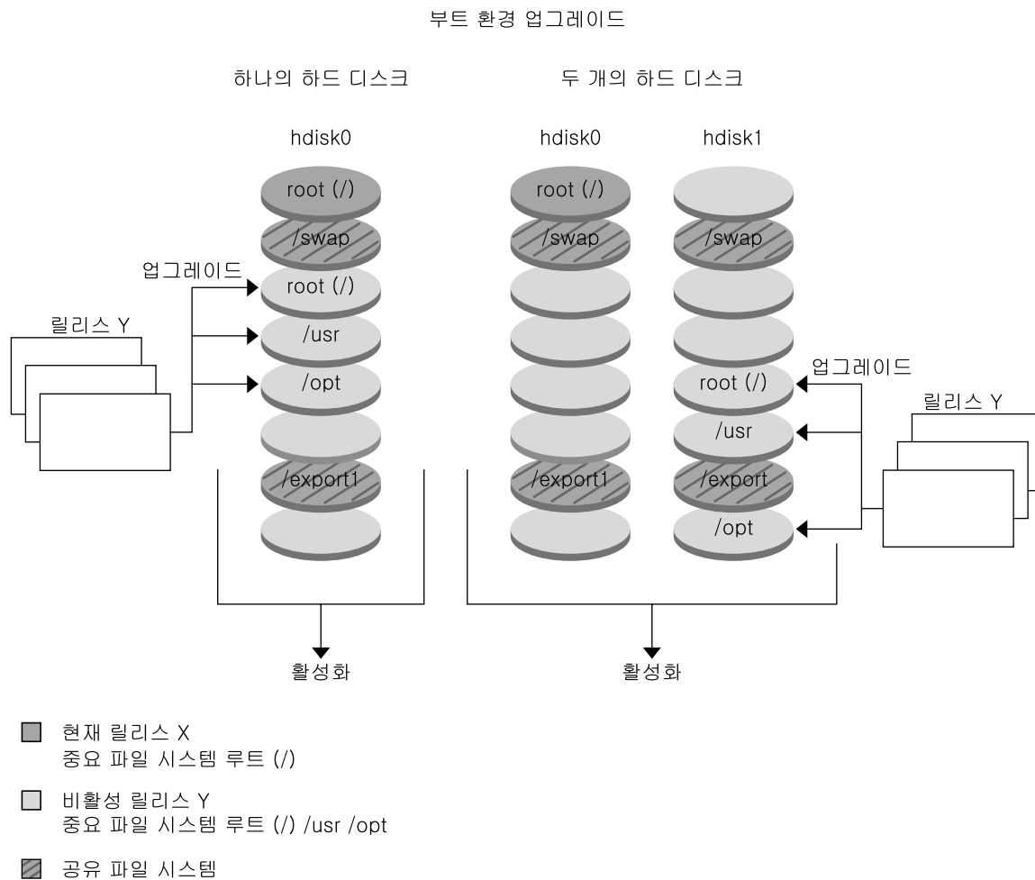
그림 30-6 비활성 부트 환경 업그레이드
