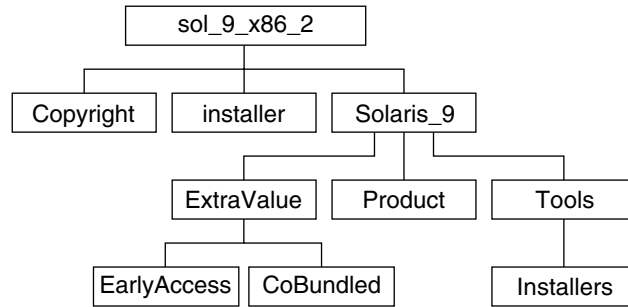
그림 B-9 Solaris 9 Software 2 of 2 x86 Platform Edition CD
