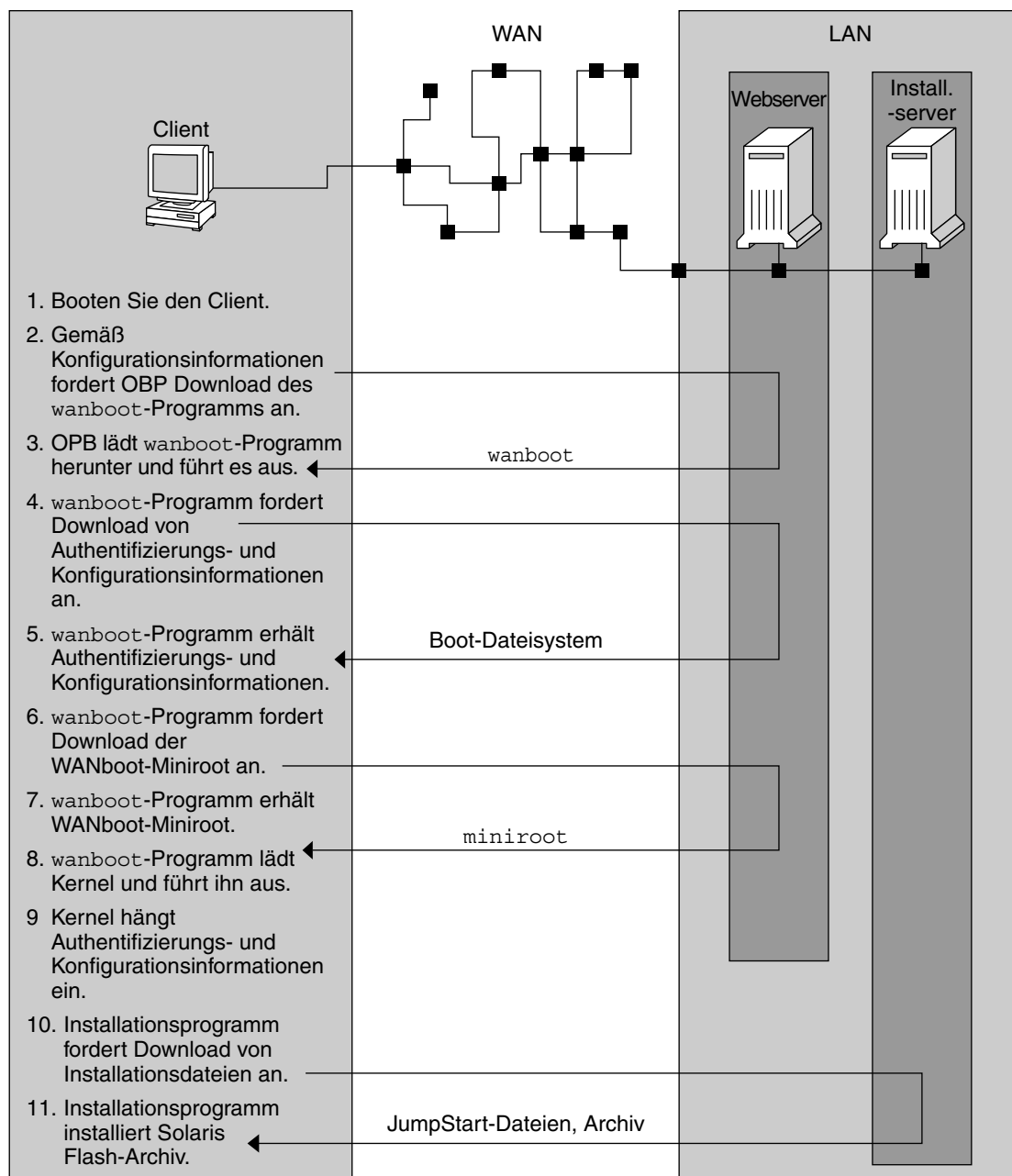
ABBILDUNG 38-1 Ereignisabfolge in einer WAN-Boot-Installation
