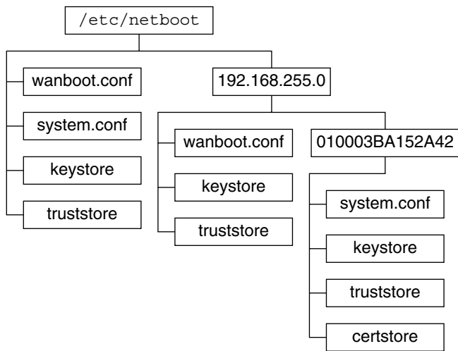
ABBILDUNG 39-2 Beispiel für das Verzeichnis /etc/netboot
