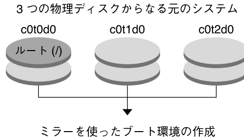
図 35-1 RAID-1 ボリューム (ミラー) の一方を切り離し、アップグレードする
