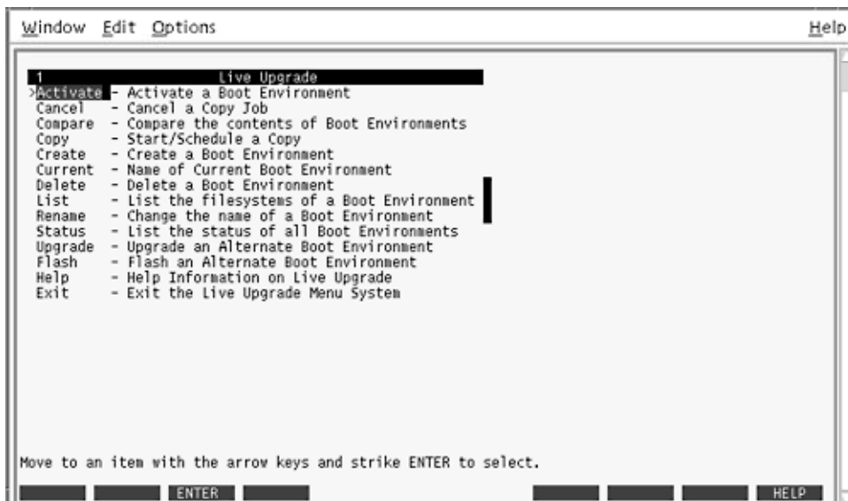
図 35-3 Solaris Live Upgrade のメインメニュー
