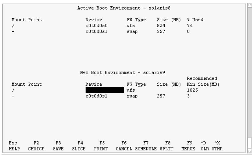
図 35-4 Solaris Live Upgrade の「Configuration」メニュー
