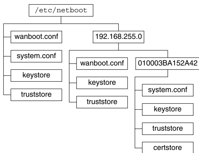
図 39-2 /etc/netboot ディレクトリの例
