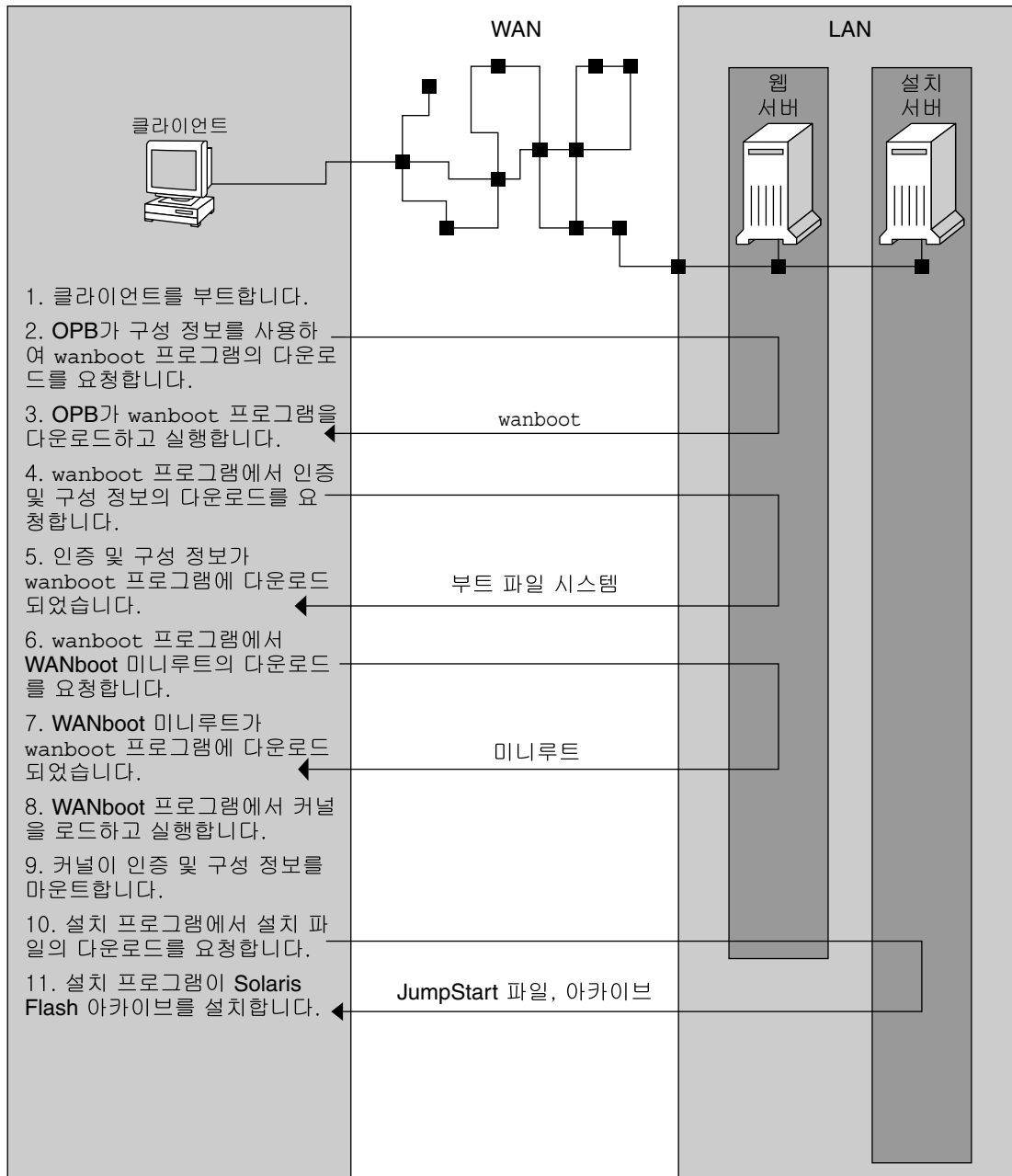
그림 38-1 WAN 부트 설치 시 이벤트 순서
