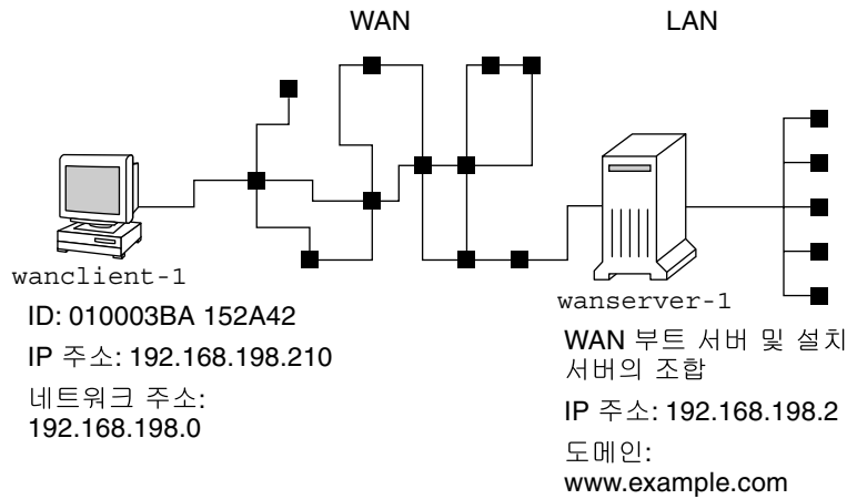
그림 42-1 WAN 부트 설치의 샘플 사이트
