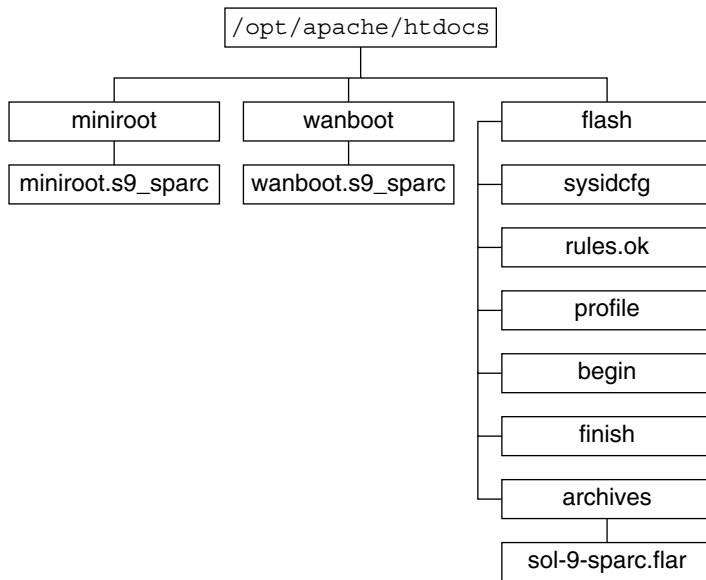
그림 39-1 문서 루트 디렉토리의 샘플 구조
