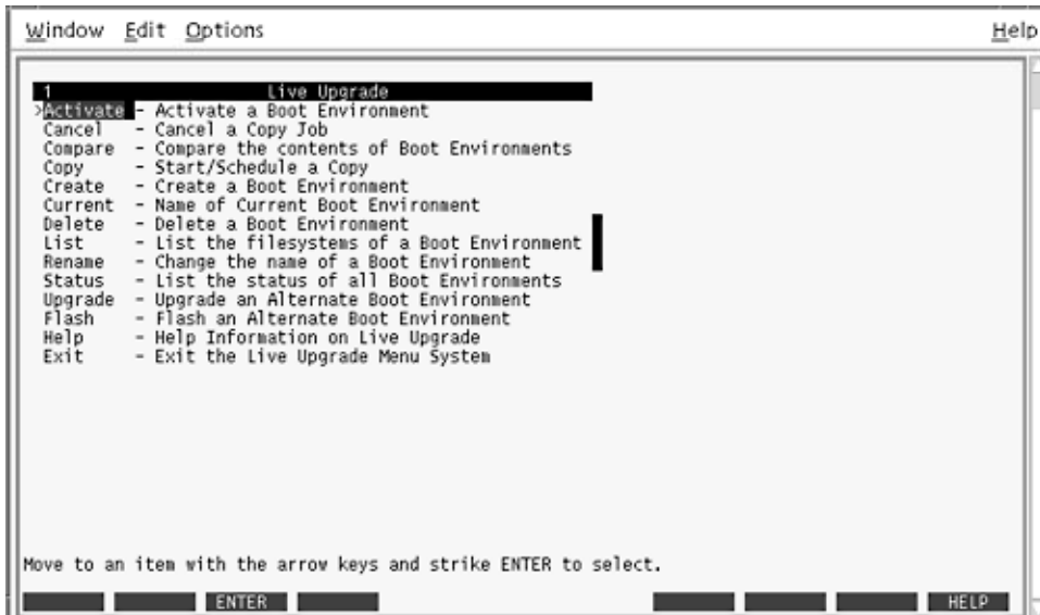
그림 35-3 Solaris Live Upgrade 기본 메뉴
