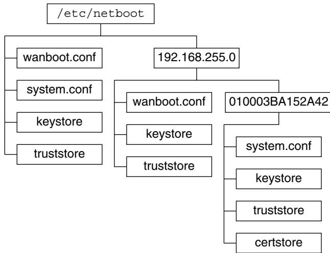
그림 39-2 샘플 /etc/netboot 디렉토리
