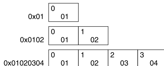
図 7-3 データの符号化方法 ELFDATA2MSB
