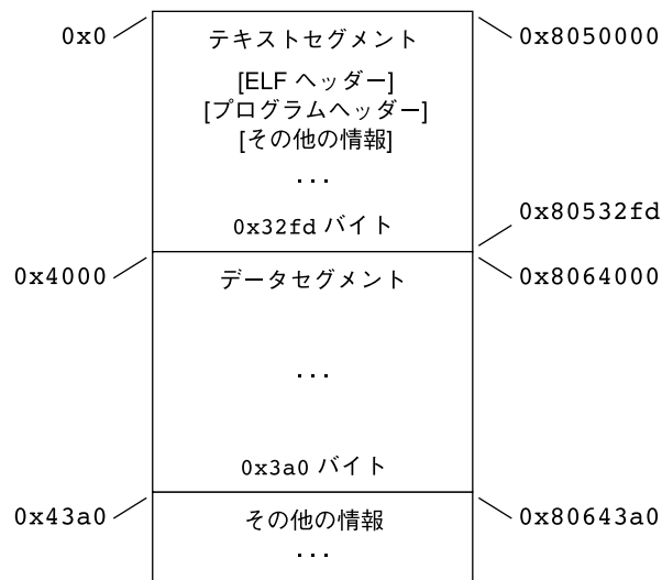
図 7-9 x86: 実行可能ファイル (64K に整列)
