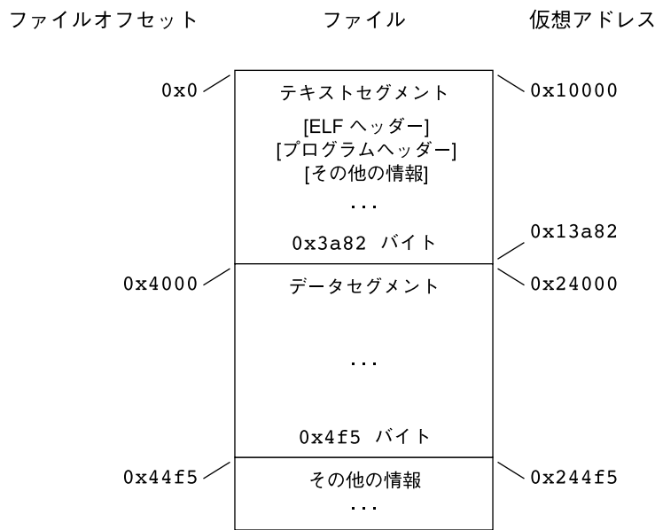
図 7-8 SPARC: 実行可能ファイル (64K に整列)
