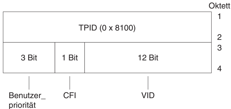
ABBILDUNG 3-1 Ethernet Tag Header Format
