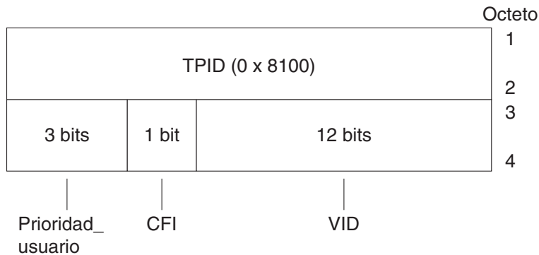
FIGURA 3-1 Formato de la cabecera de marca en la trama Ethernet
