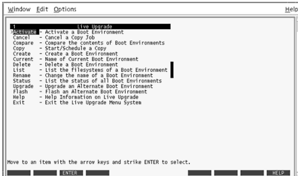
ABBILDUNG 35-2 Das Hauptmenü von Solaris Live Upgrade
