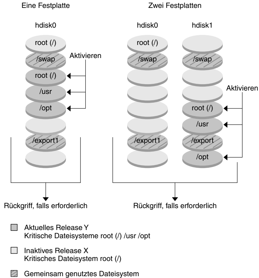
ABBILDUNG 33-8 Aktivieren einer inaktiven Boot-Umgebung
