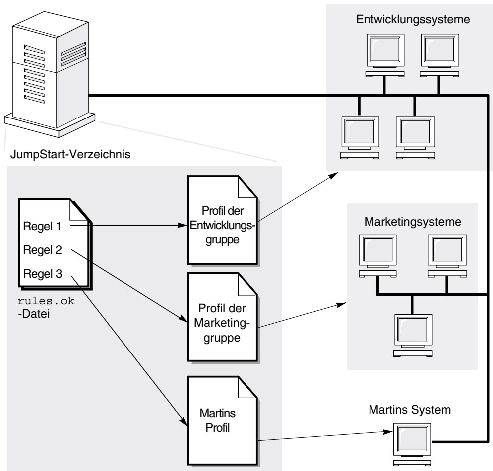
ABBILDUNG 25-2 Prinzip einer benutzerdefinierten JumpStart-Installation: Beispiel für vernetzte Systeme
