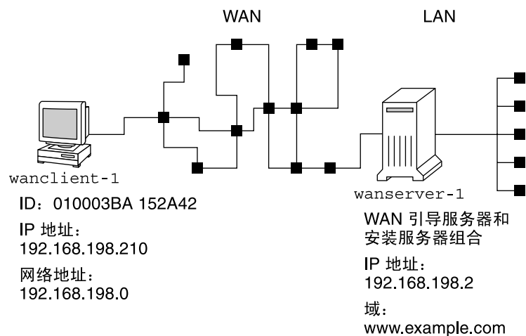
图 45-1 WAN Boot 安装的站点样例
