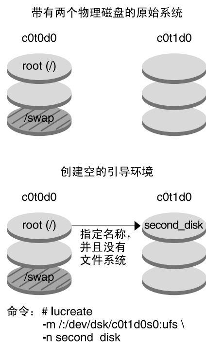
图 35-4 创建空引导环境
