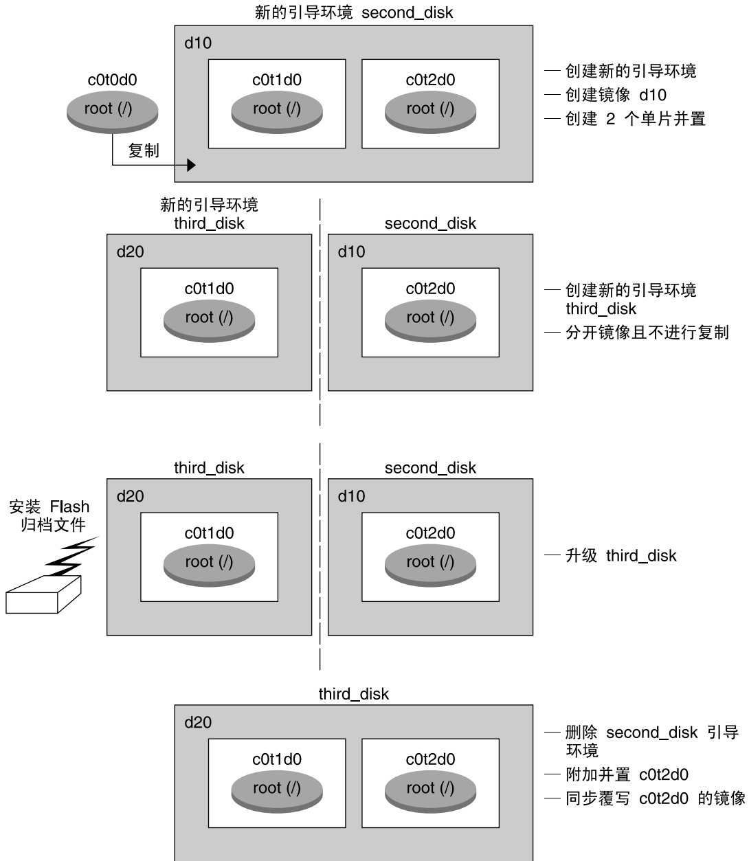
图 38-2 分离和升级 RAID-1 卷（镜像）的一面（继续）
