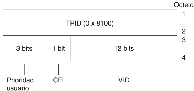
FIGURA 2-1 Formato de la cabecera de marca en la trama Ethernet
